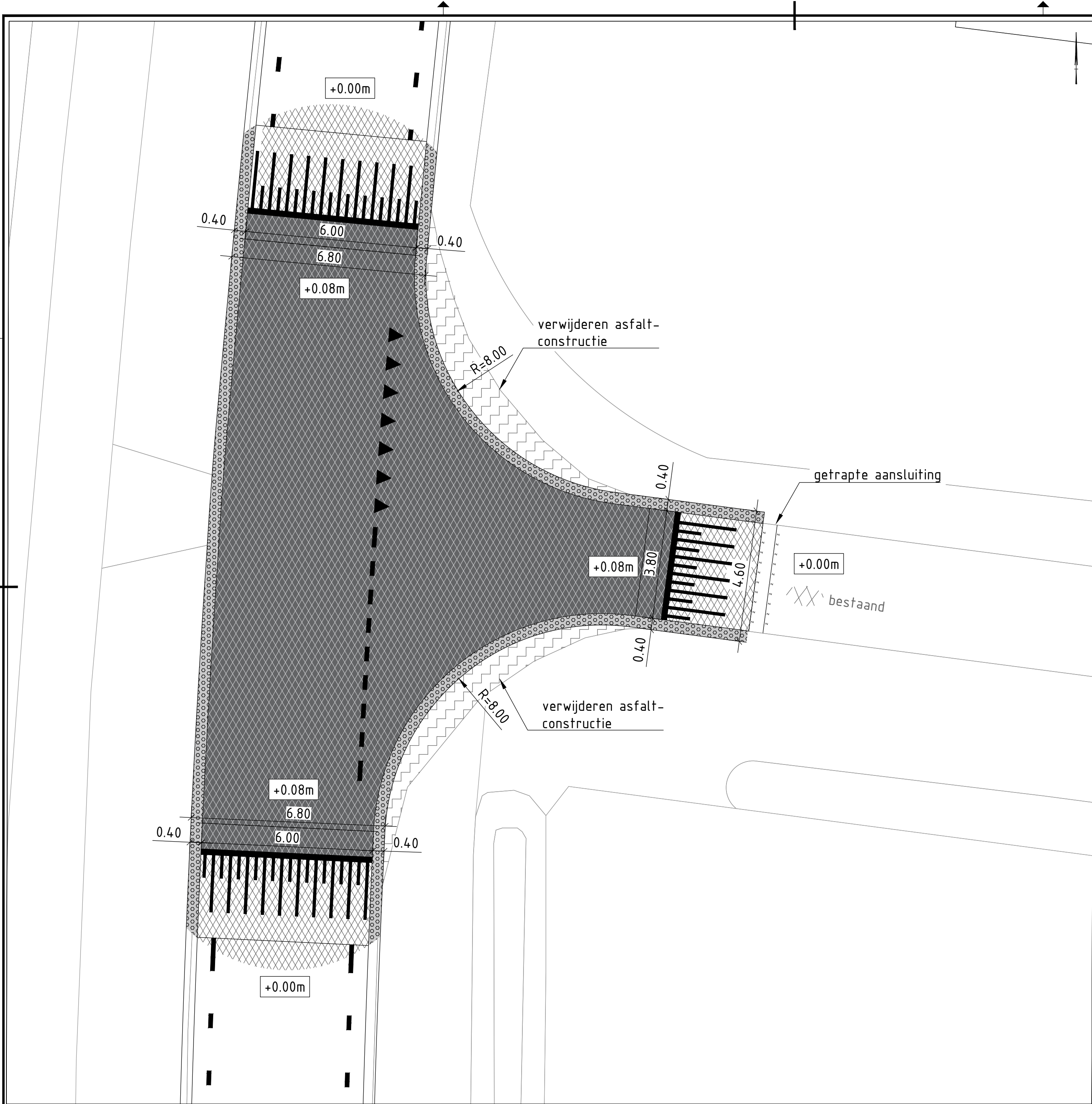
Kruising De Steegde - Grondselweg Schaal 1 : 100
