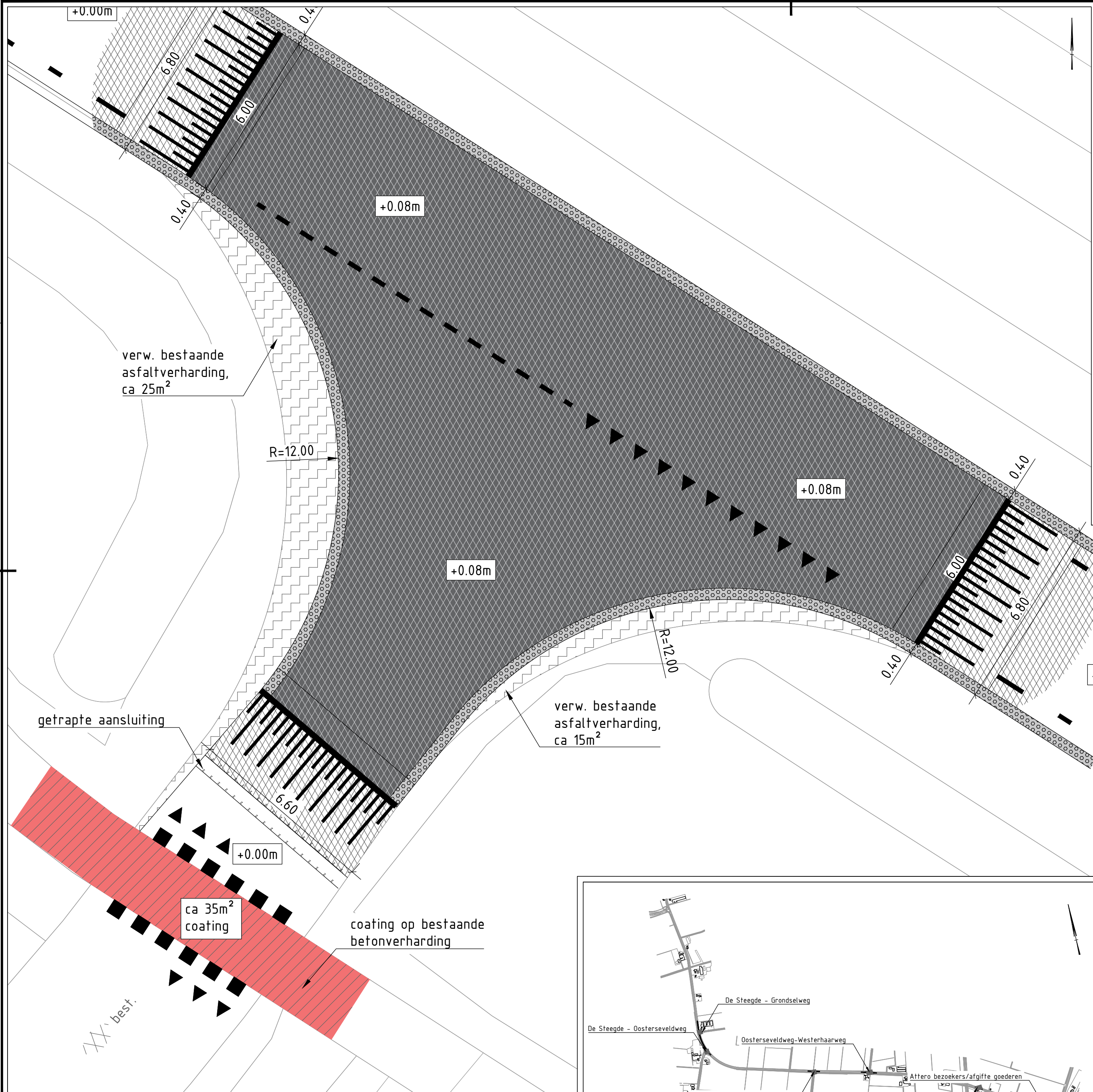
Kruising Oosterseveldweg - Nijverheidsweg Schaal 1 : 100
