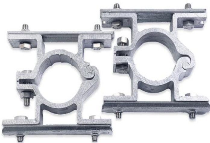
Afbeelding 3 (scharnierbeugels)
