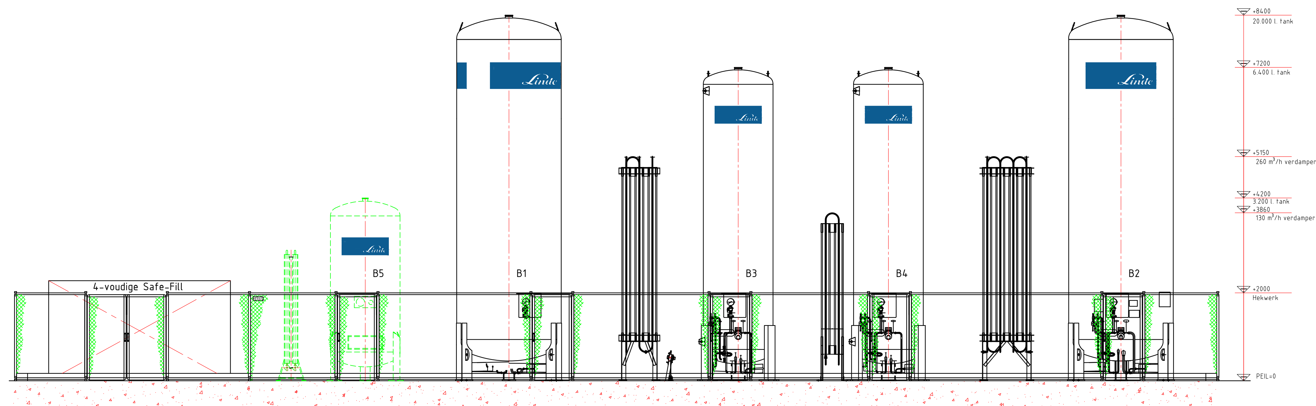
Aanzicht A-A
