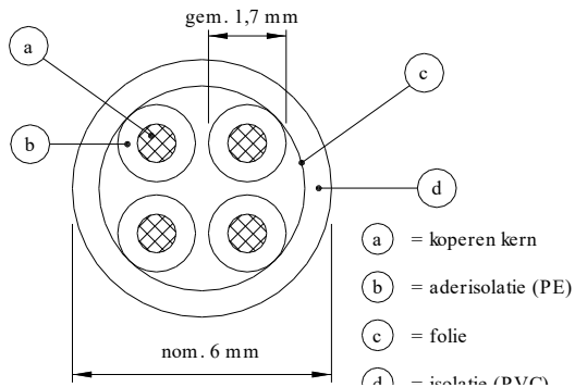
..... Figuur A.1. Kabeldoorsnede luskabel
