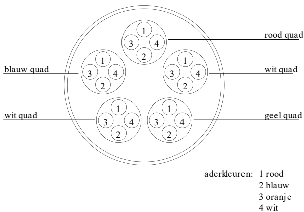
..... Figuur C.1. Doorsnede detectorkabel
