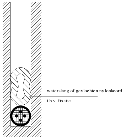
..... Figuur 5.8 Fixeren van lustoe- voer- en luskabel in zaagsnede
