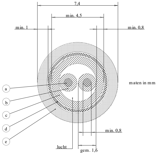
..... Figuur B.1. Doorsnede lustoeverkabel
