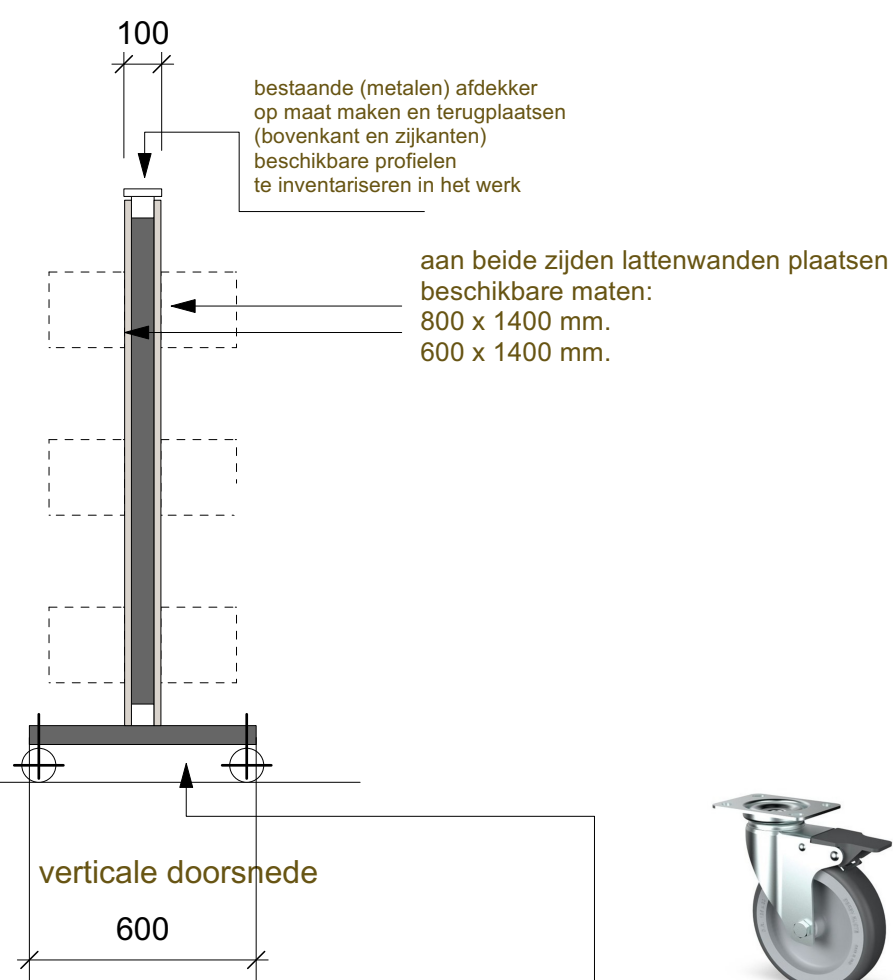
aangelast dwars-profiel met 4 x zwenkwiel met rem
