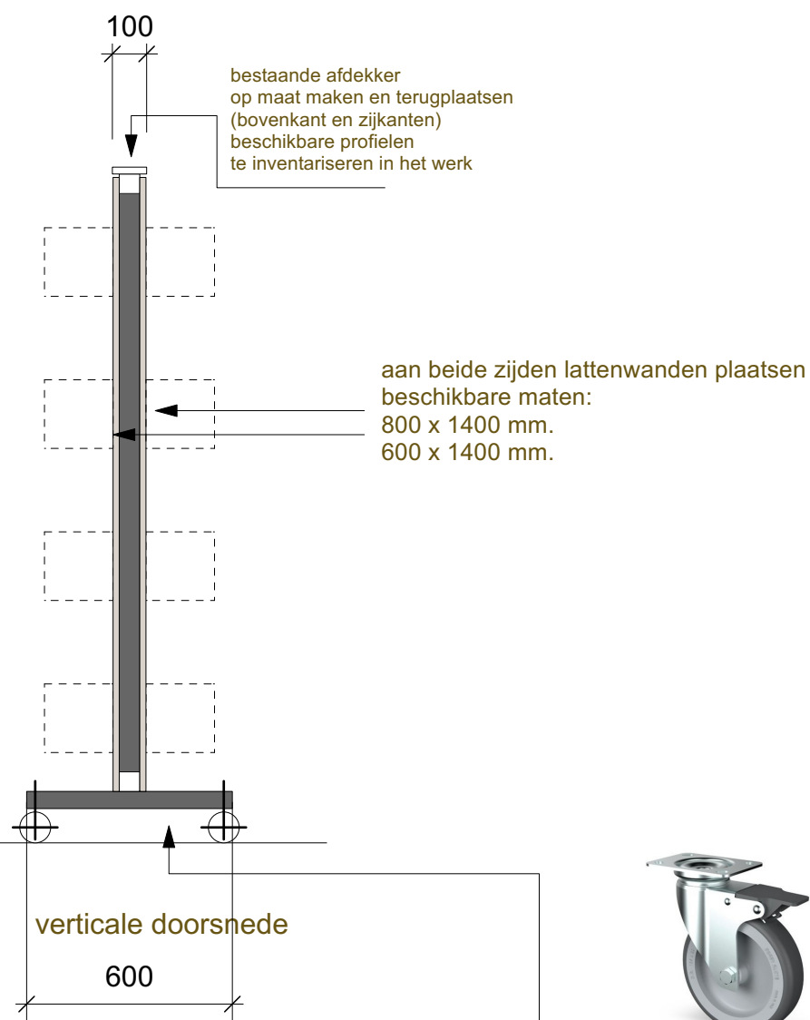
aangelast dwars-profiel met 4 x zwenkwiel met rem
