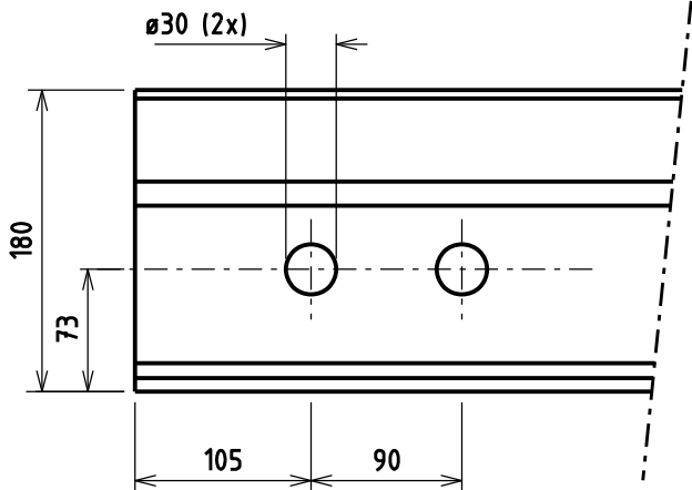
Gatenpatroon t.b.v. lasplaten. Schaal 1:5
