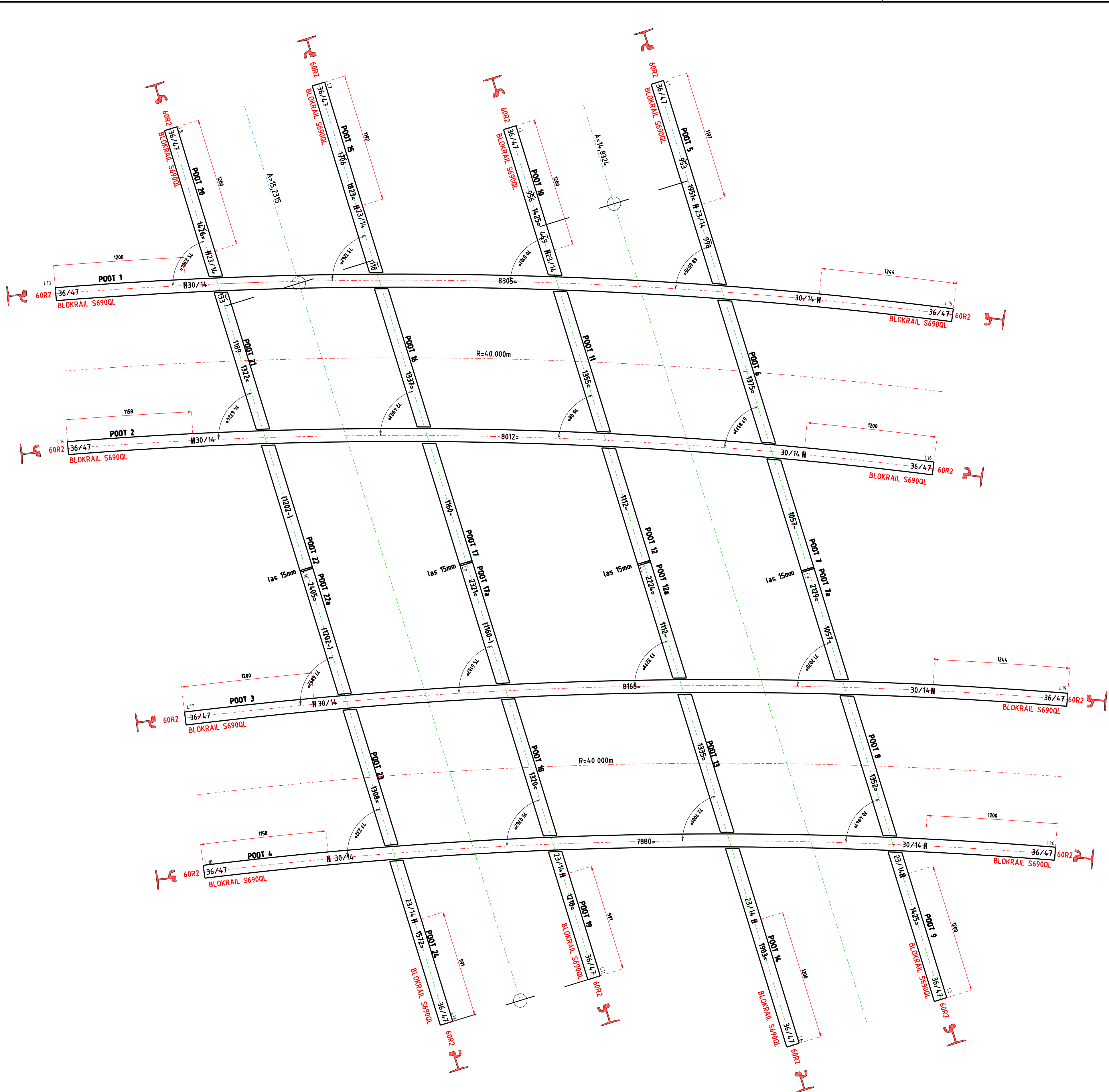
Gatenpatroon t.b.v. lasplaten. Schaal 1:5
