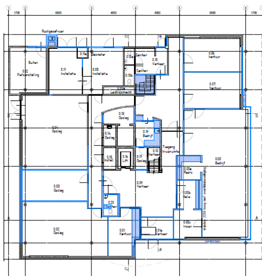
BG huidige indeling
