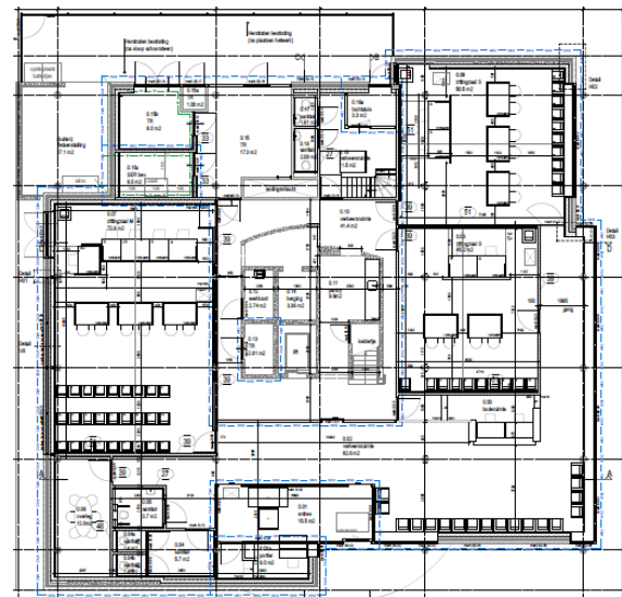
BG Nieuwe indeling
