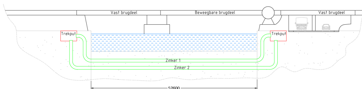
Figuur 2, principeschets dubbele zinkerconstructie
