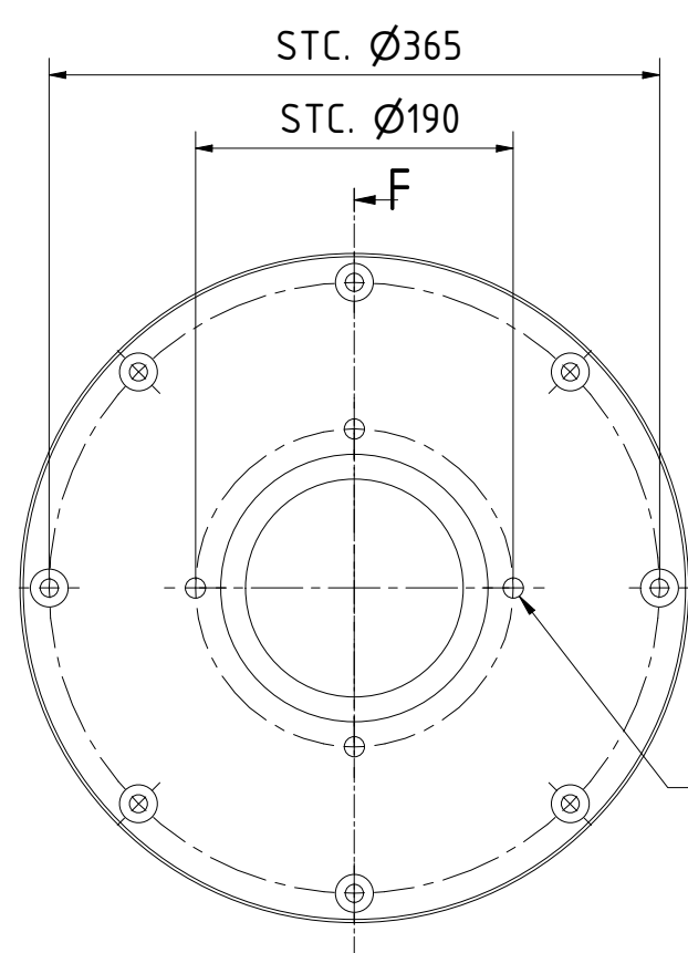
Lagerplaat 1 : 5
