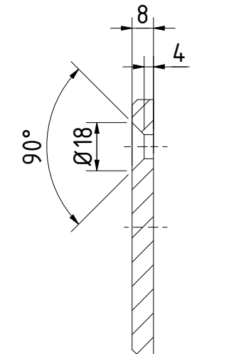
DOORSNEDE D-D 1 : 2
