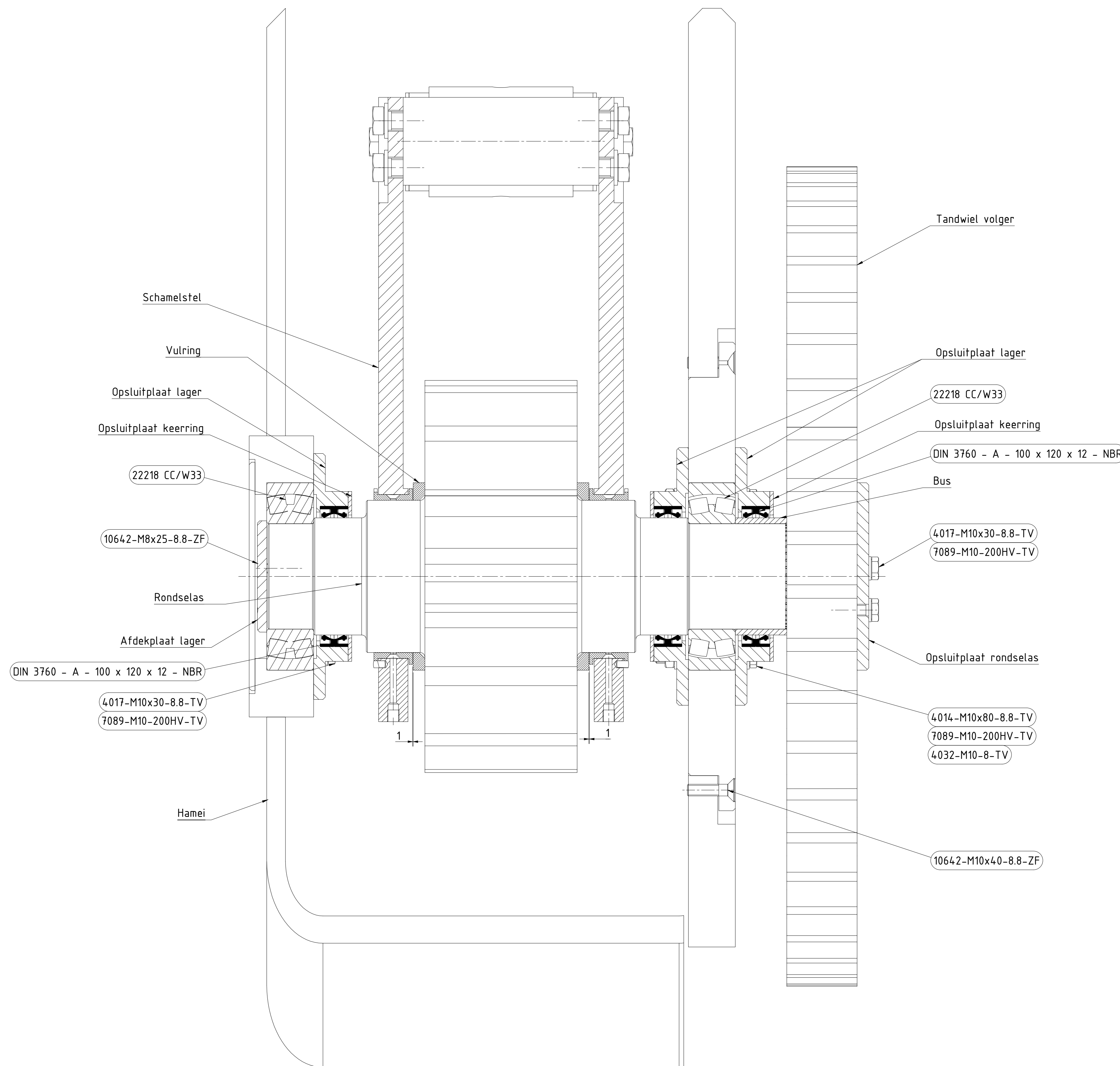
Sam. rondselas / schamelstel 1 : 2
