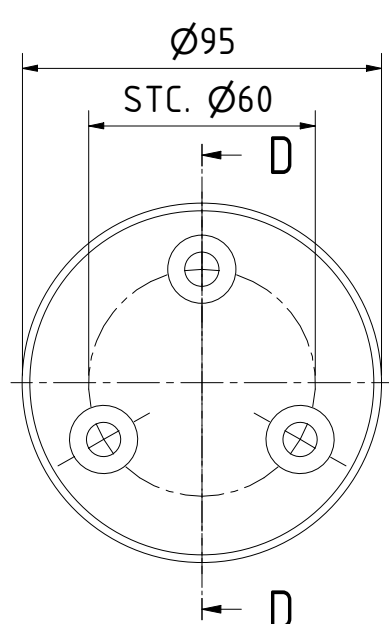
Afdeksplaat lager 1 : 2
