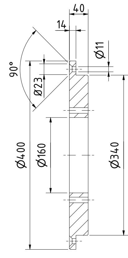
DOORSNEDE F-F 1 : 5
