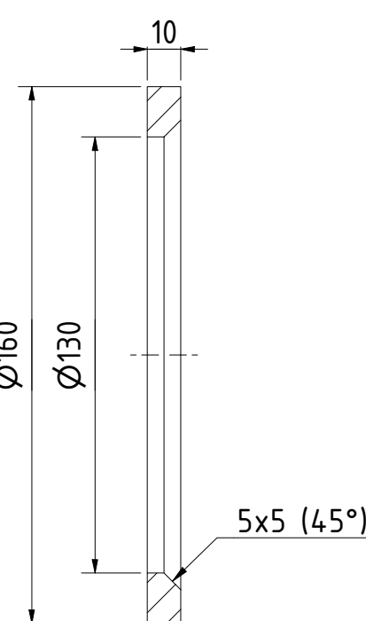
DOORSNEDE E-E 1 : 2
