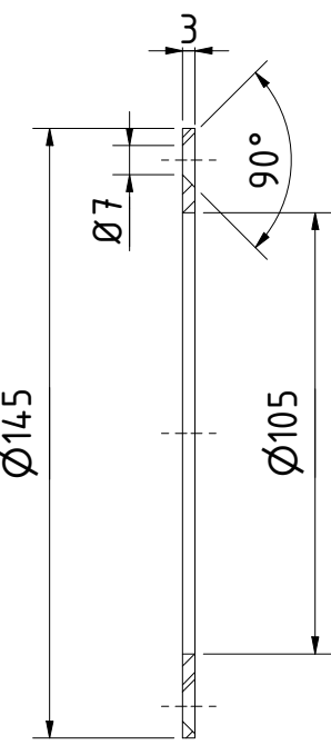
DOORSNEDE C-C 1 : 2
