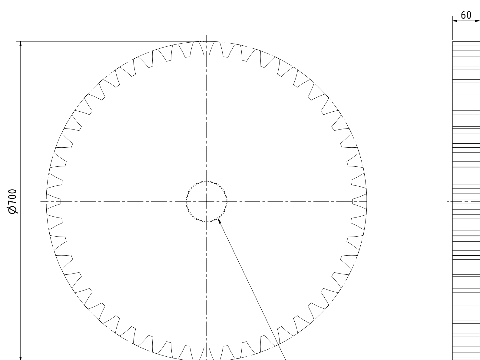
Tandwiel volger 1 : 5
