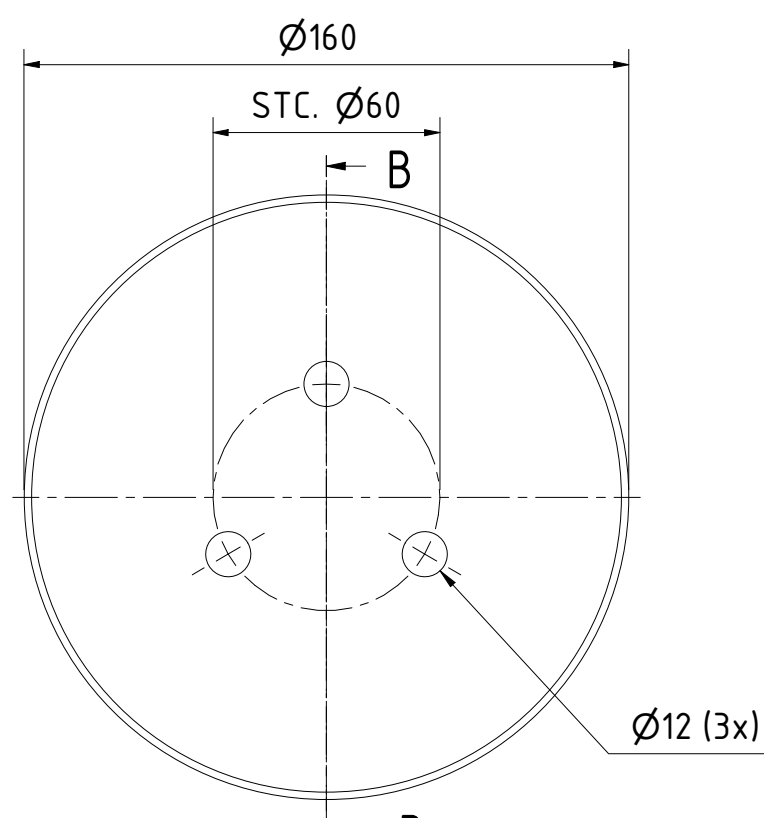
Opsluitplaat rondselas 1 : 2
