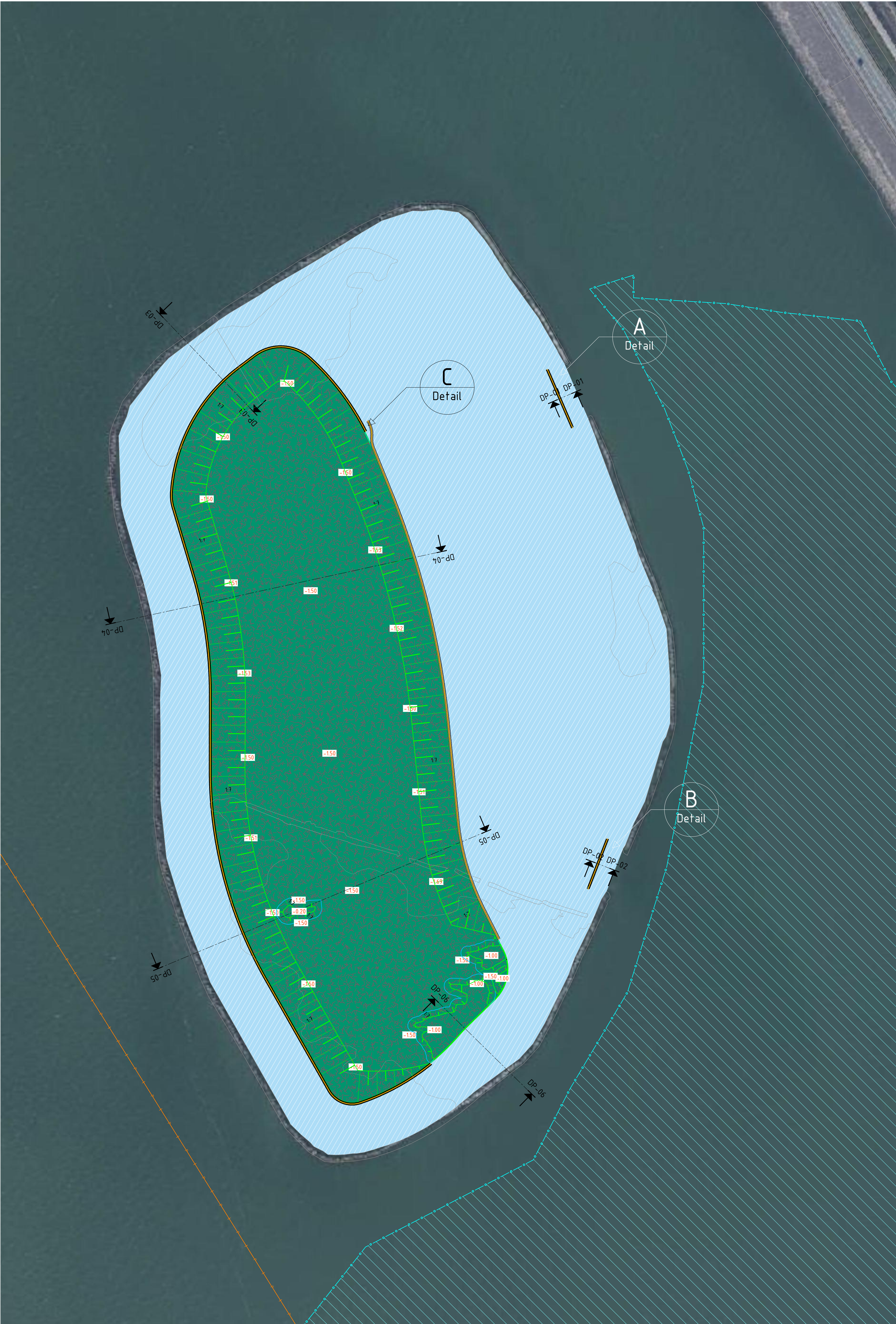
Overzichtstekening Proefmoeras Ierst
