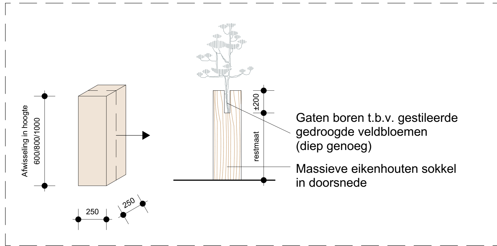
Schaal 1:20
