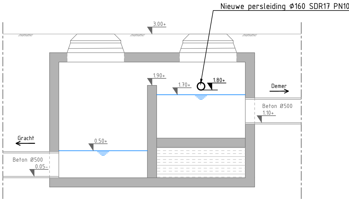
Bestaande overstortput; profiel A-A Schaal 1:50
