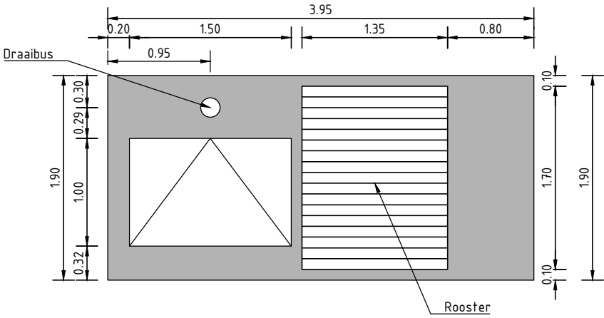
Bovenaanzicht dekplaat tbv sparigen Schaal 1:50
