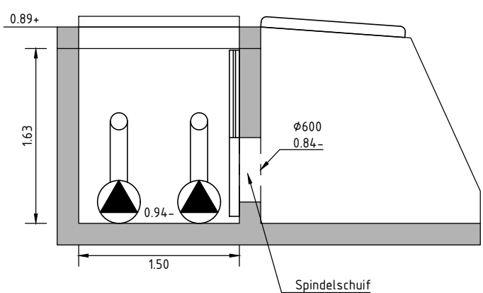
Doorsnede A-A Schaal 1:50
