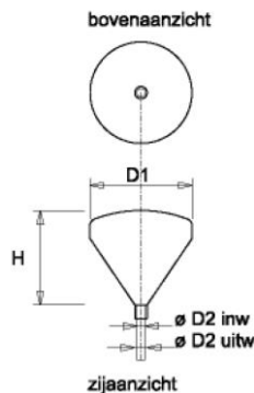
Figuur 4: Kegelmiddel armaturen
