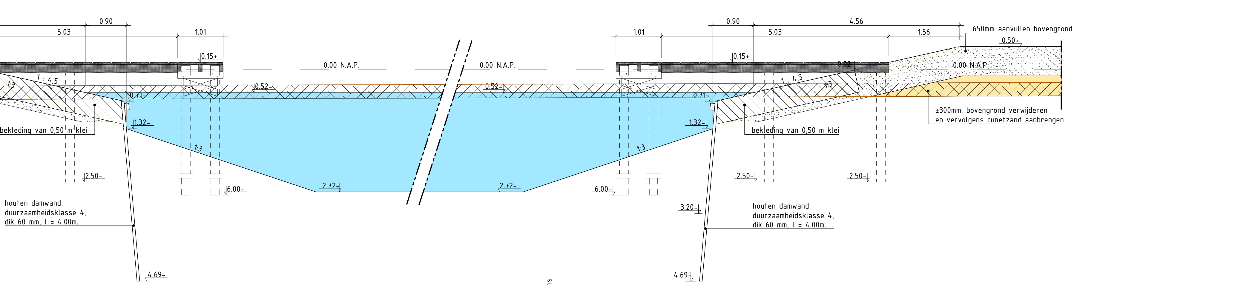
Profiel 12-12
