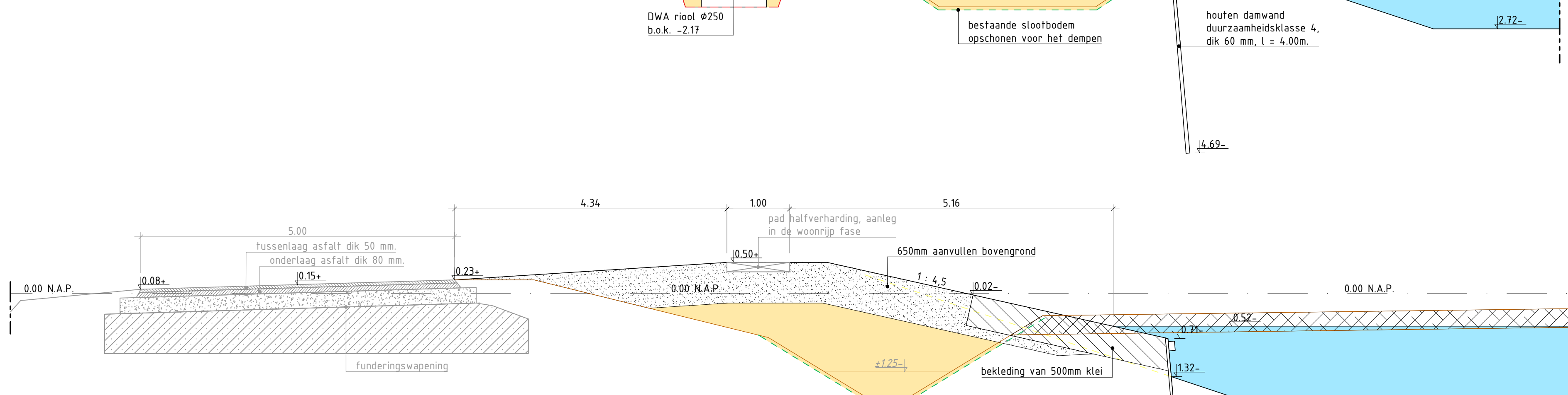
Profiel 7-7
