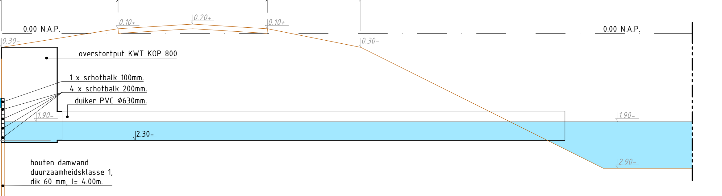
Profiel 9-9
