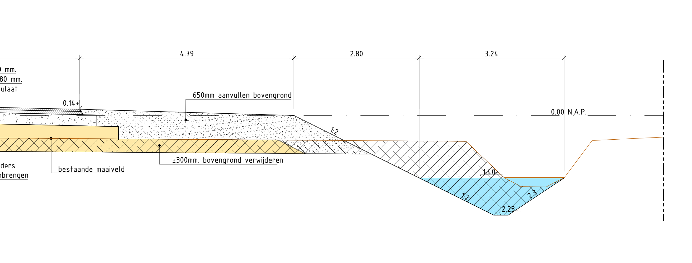
Profiel 12-12
