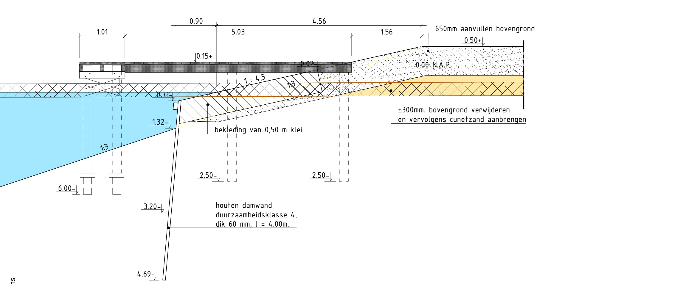
Profiel 12-12
