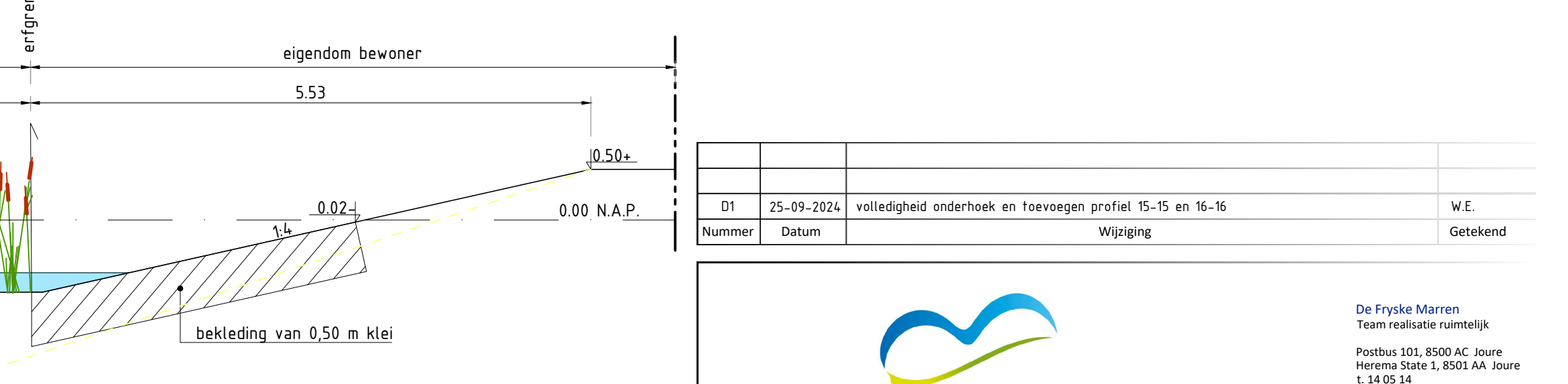
Profiel 14-14
