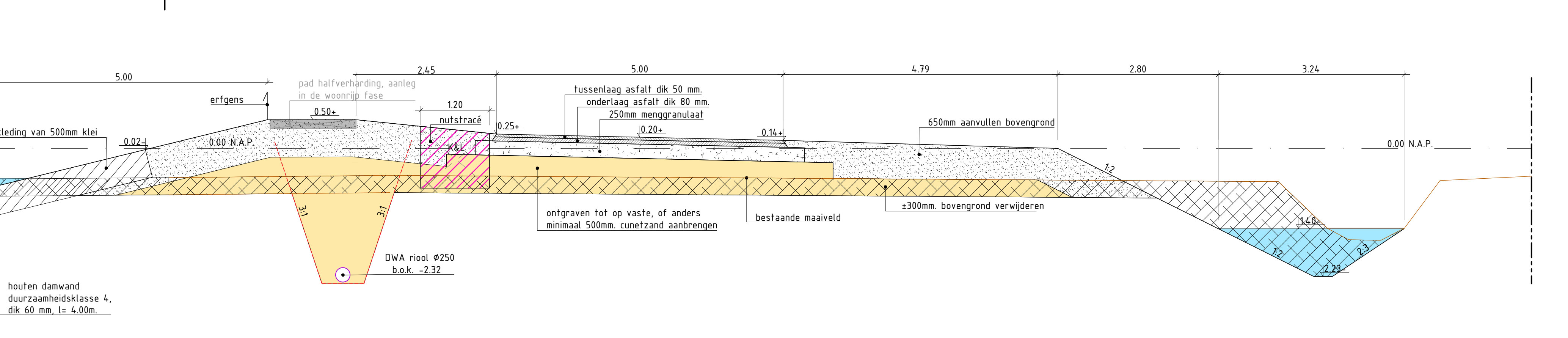
Profiel 12-12
