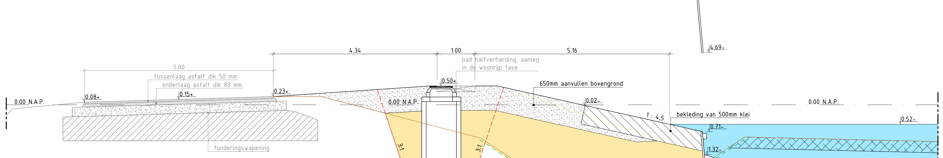
Profiel 6-6
