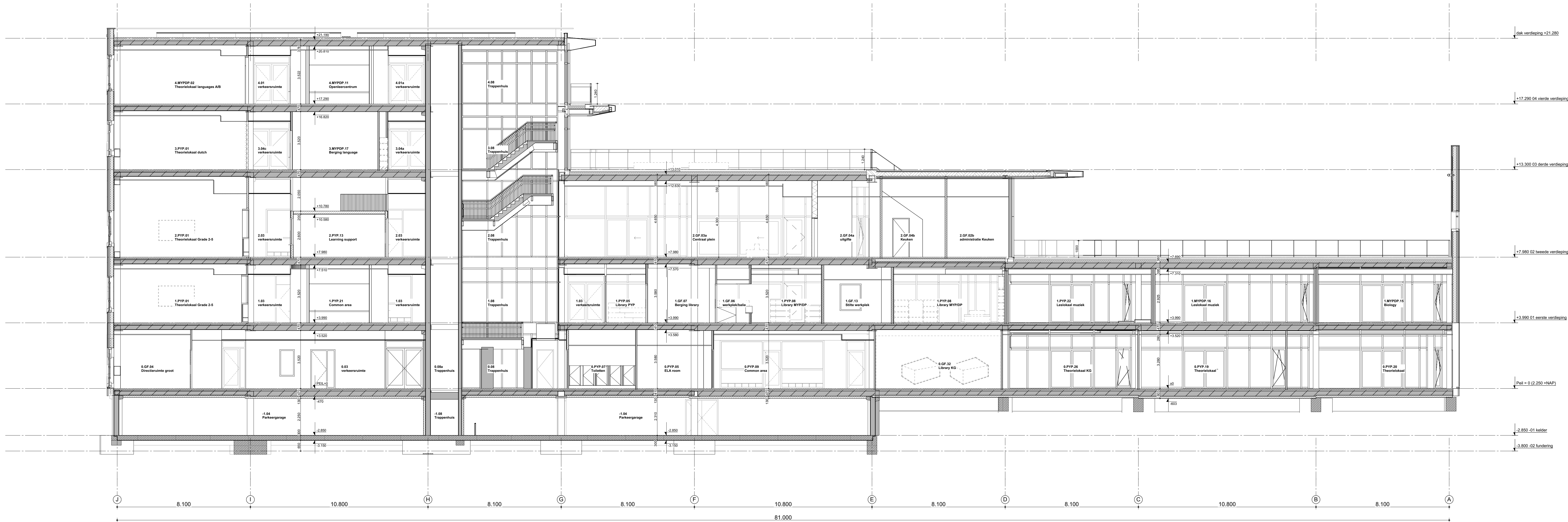
Doorsnede D-D
