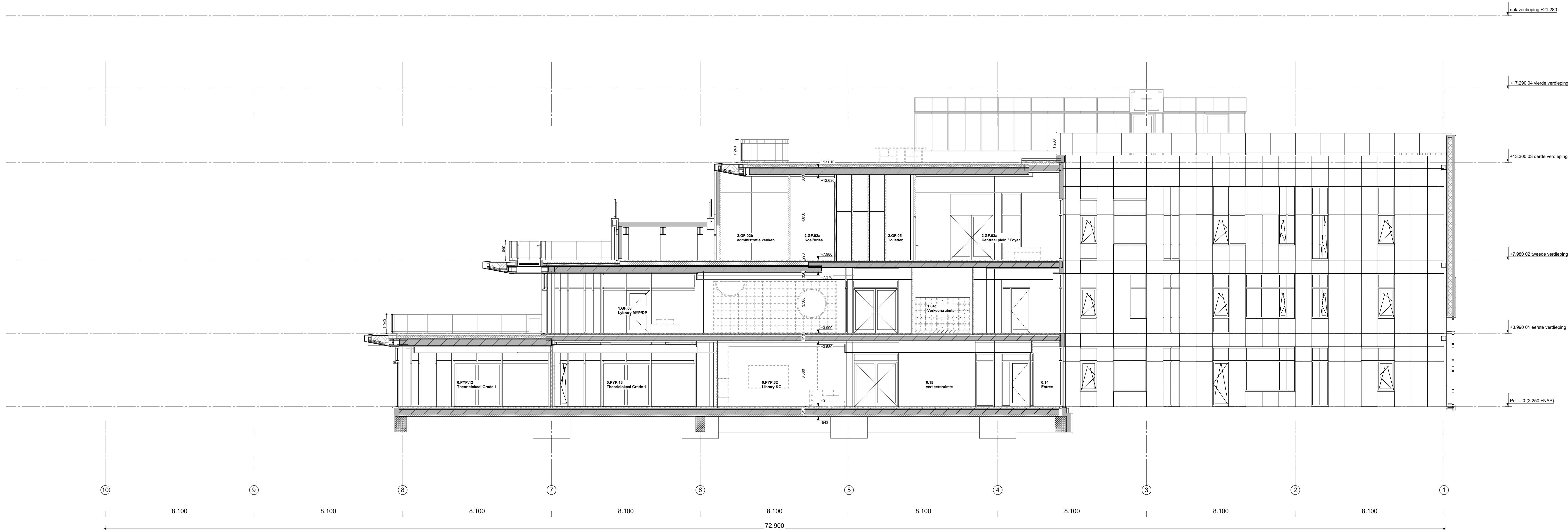
Doorsnede C-C
