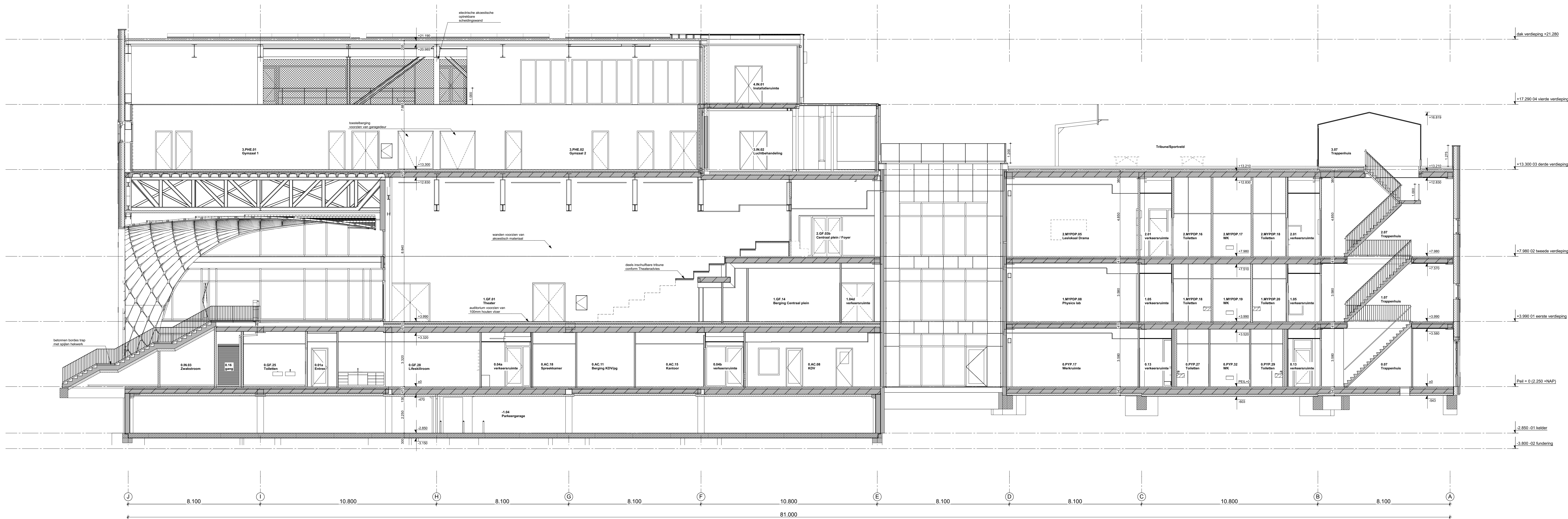
Doorsnede B-B
