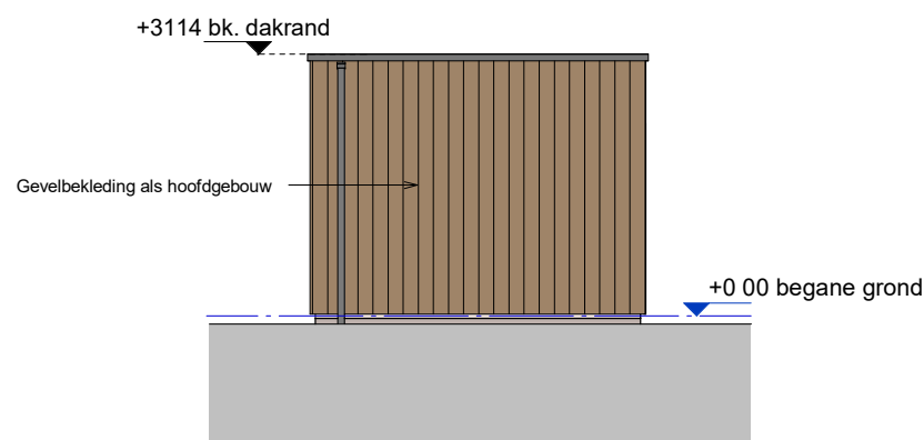
Achtergevel
