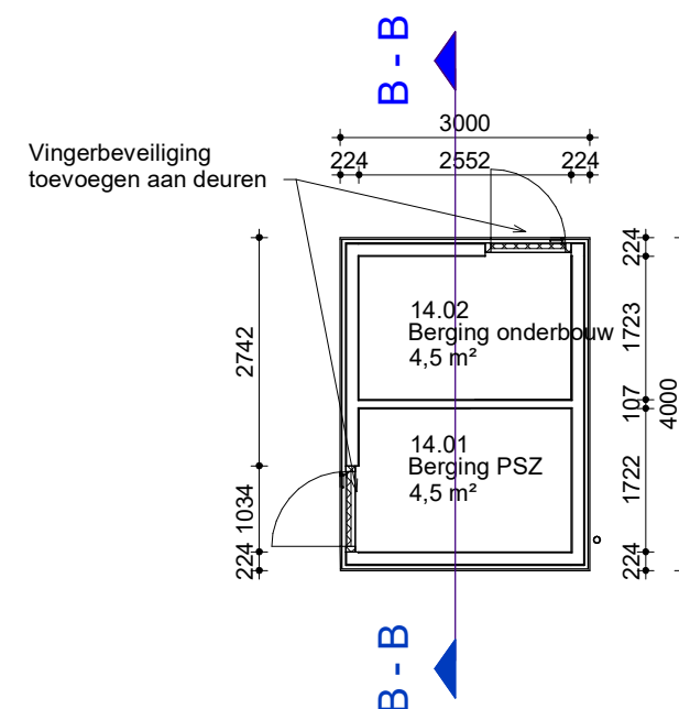
Begane grond
