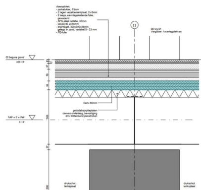
Figuur 13: Vloeropbouw begane grond vloer Circl
