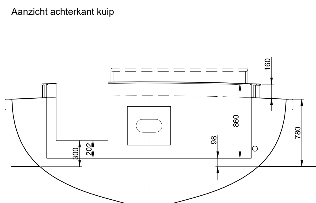
Aanzicht achterkant kuip
