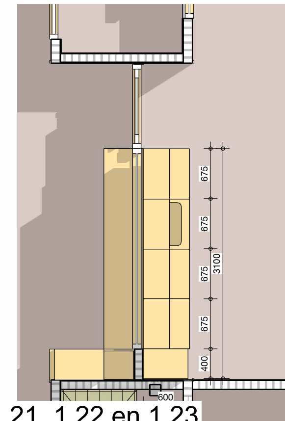
Pantry 1.21, 1.22 en 1.23
