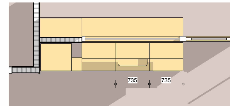
Pantry 1.01 en 1.04
