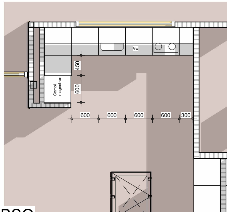
Keuken BSO
