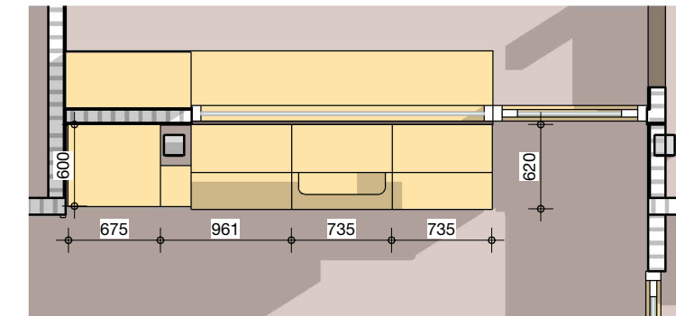
Pantry 1.02 en 1.03
