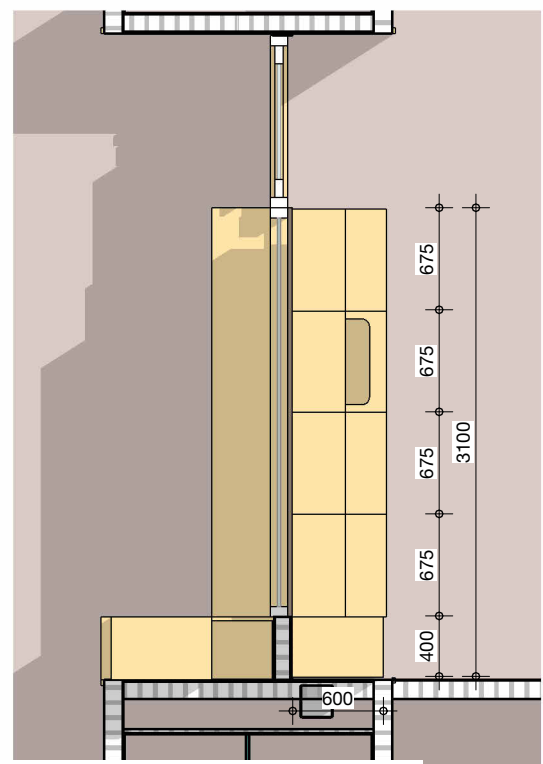
Pantry 0.35, 0.36 en 0.37
