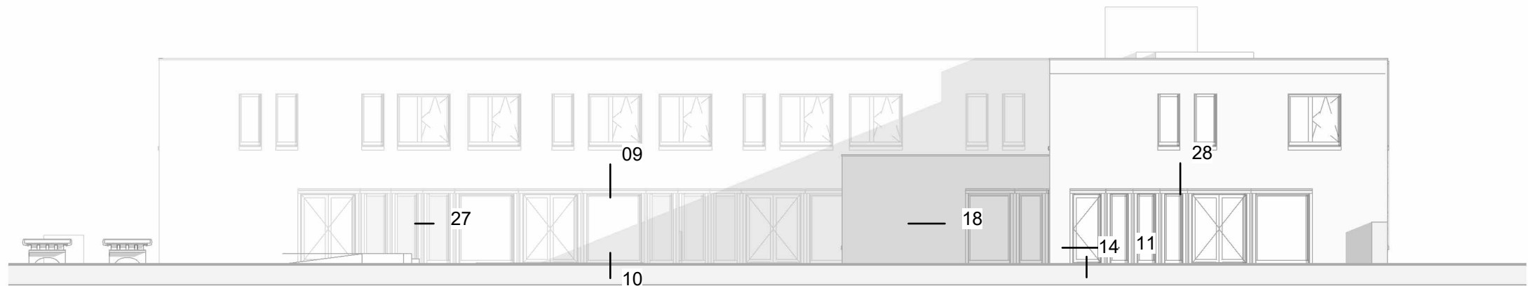
Zuidgevel
