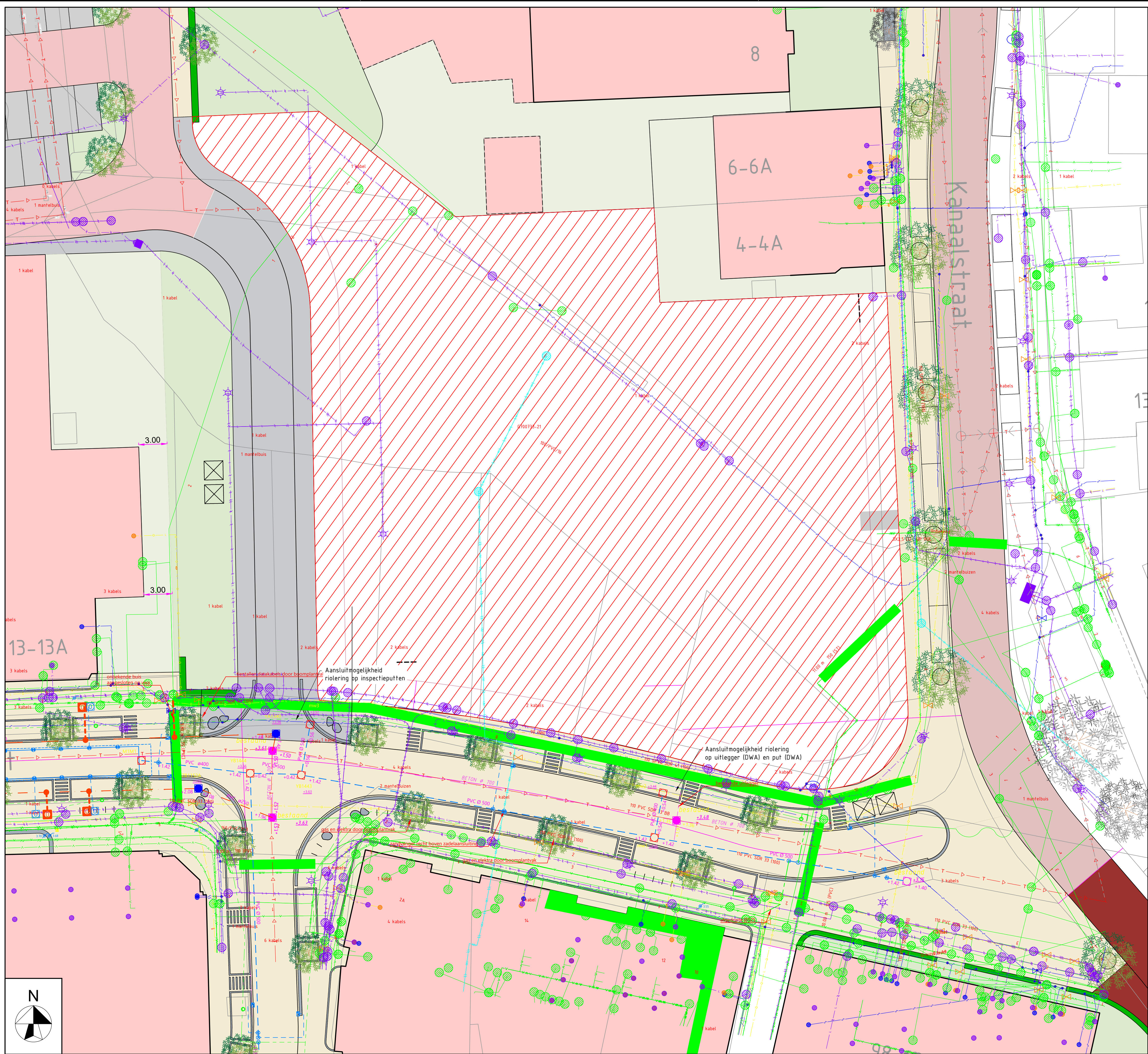
SITUATIE Schaal 1:1000
