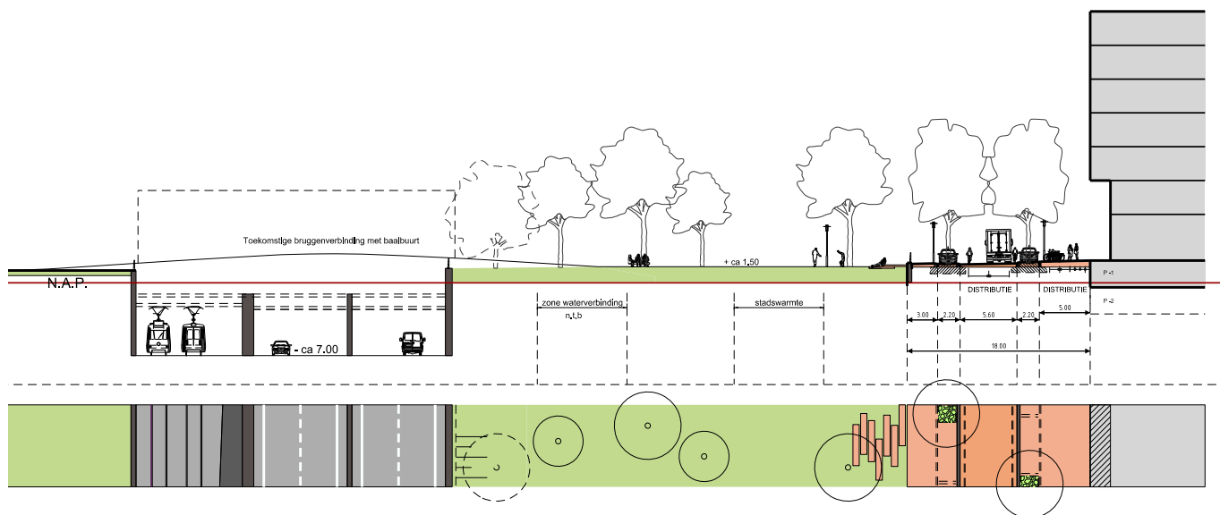
Profiel 9
