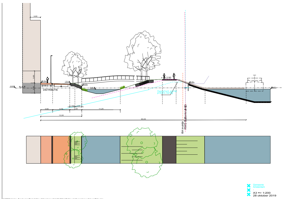
Profiel 6
