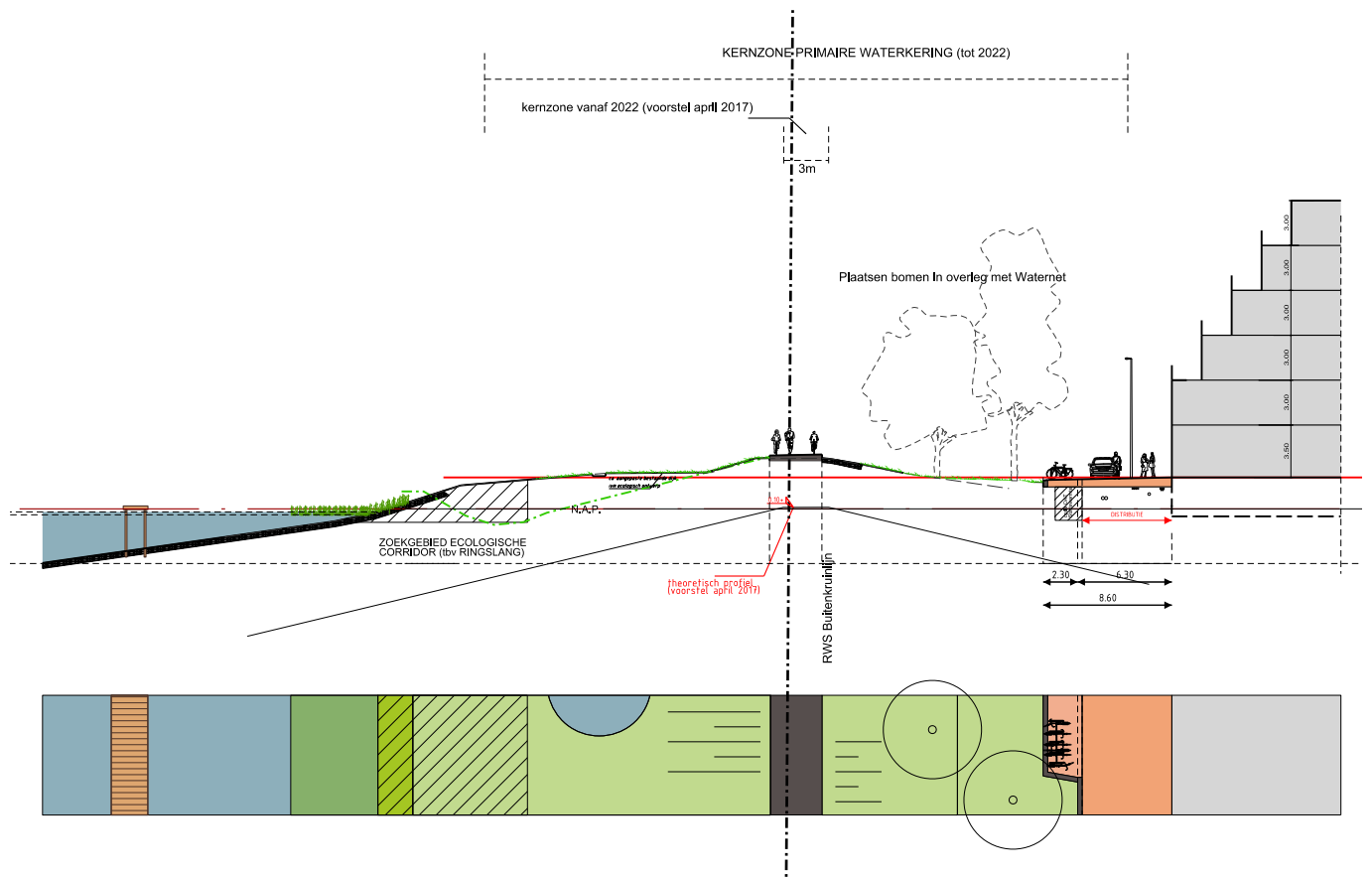
Profiel 4
