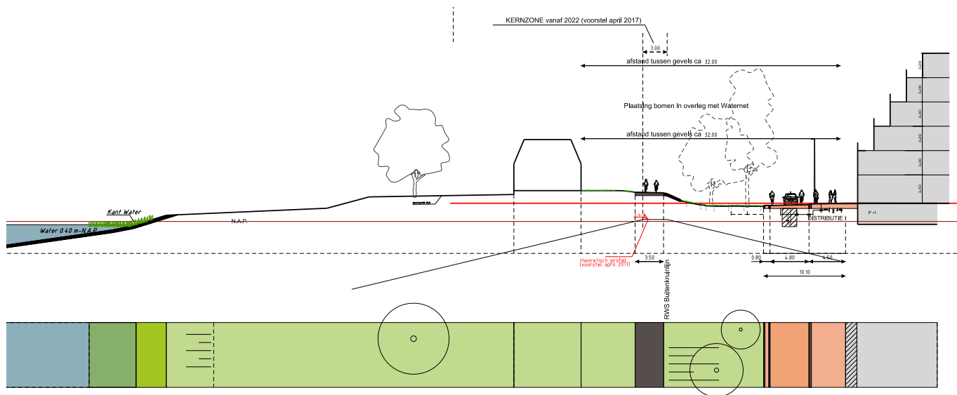
Profiel 5
