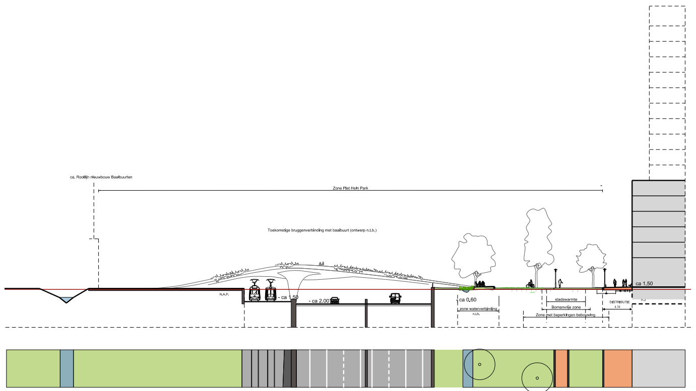
Profiel 8
