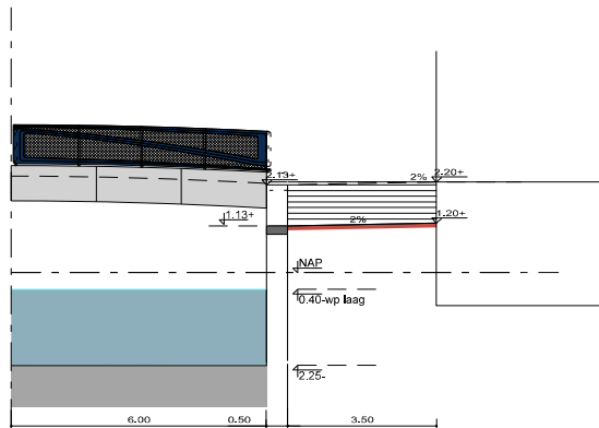
halfhoge kade
