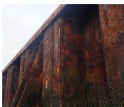
Figuur 7.5: Corrosie aan de damwanden.
