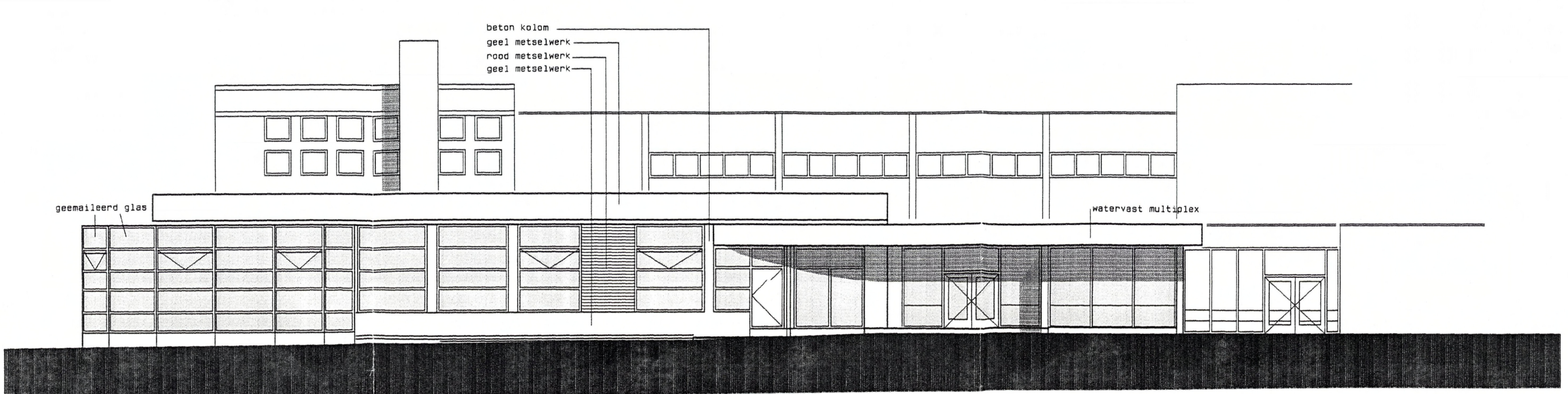
GEVEL 2 SCHOOLSTRAAT
