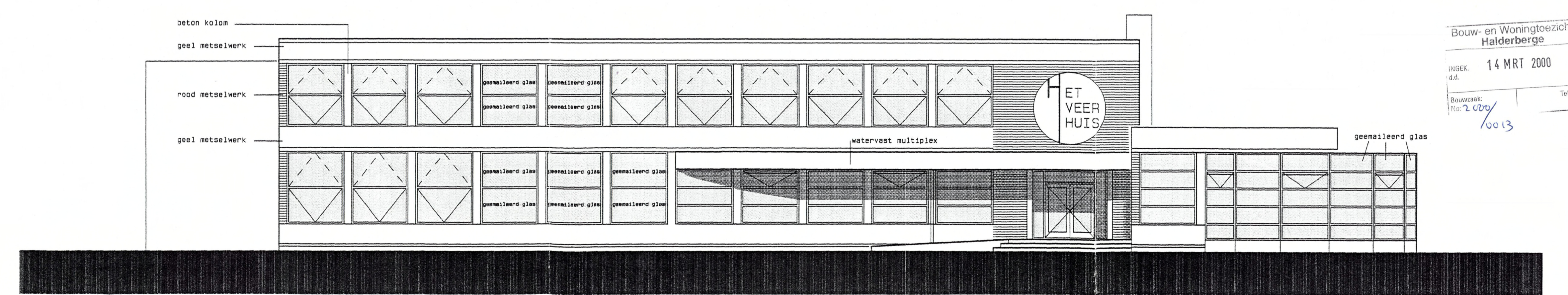
GEVEL 1 VEERKENSEWEG
