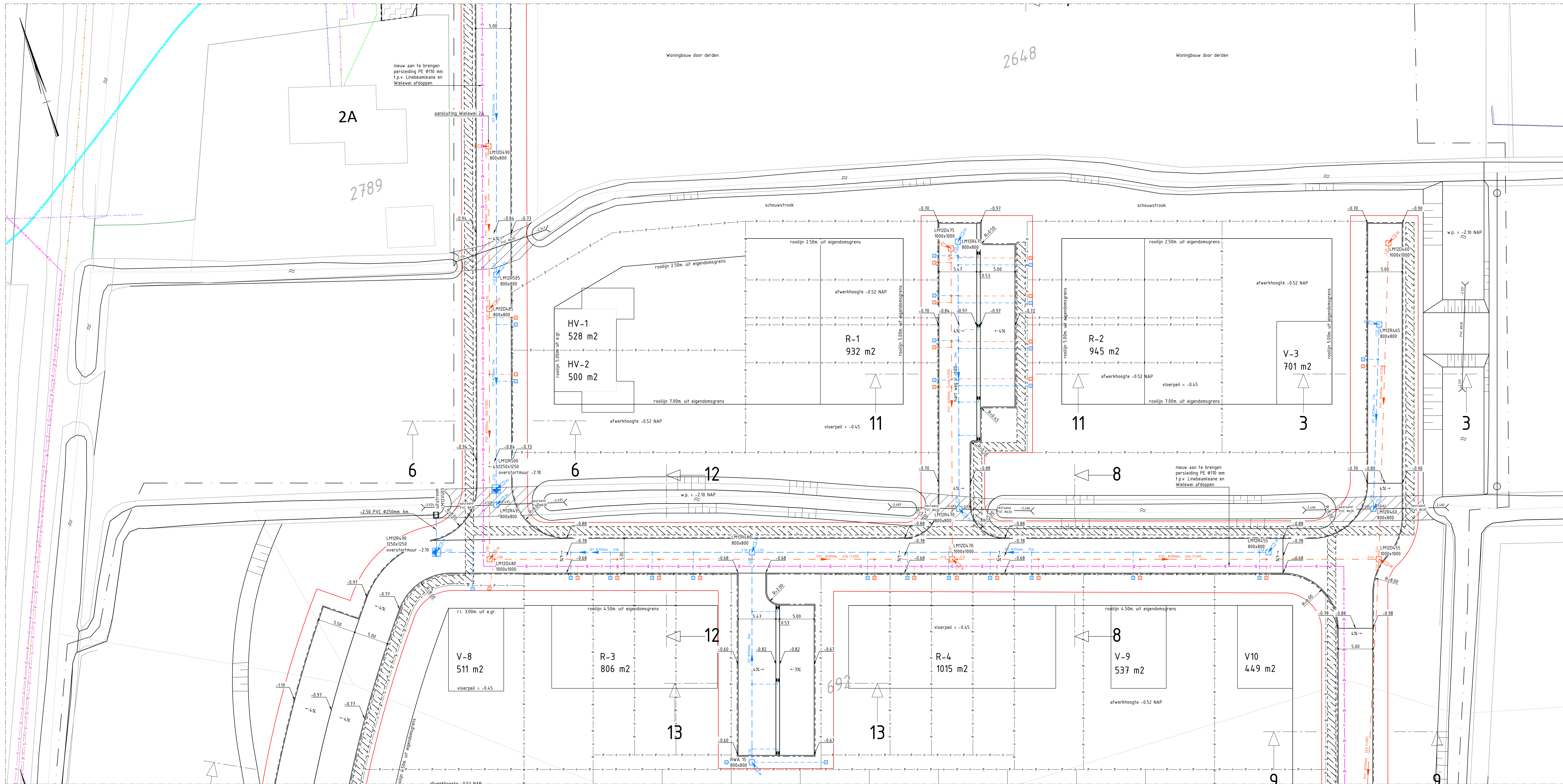
Bovenaanzicht schaal 1:200
