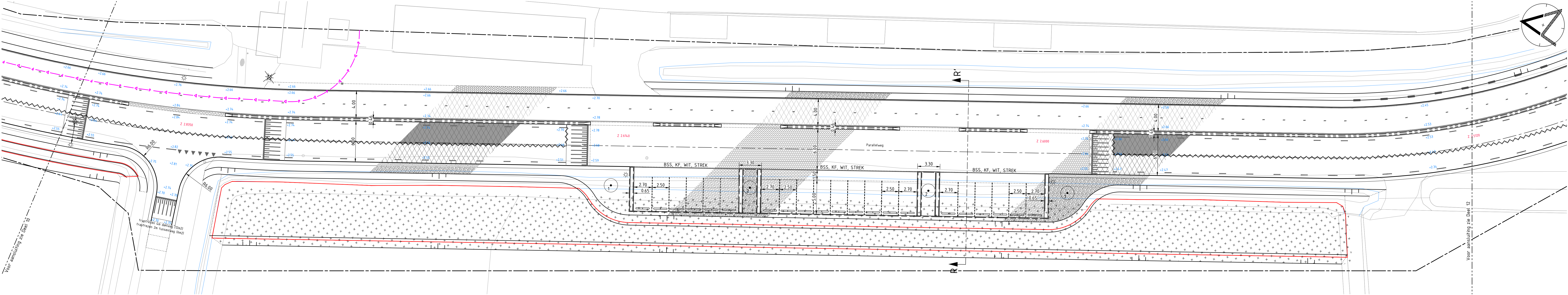
Deel 11 - PARALLELWEG - DE LUCHT Schaal 1:200
