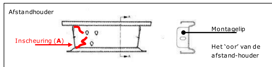
Afbeelding 25 Schematische weergave van een ingescheurde afstandhouder
