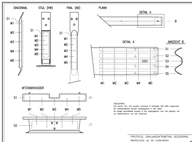
Afbeelding 36 Geleiderailonderdelen
