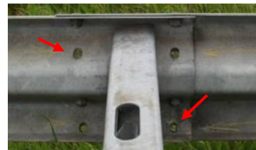
Afbeelding 13 Bevestigingsmiddelen ontbreken
