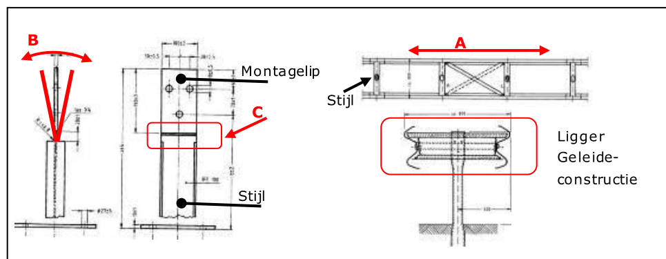
Afbeelding 27 Schematische weergave van een ingescheurde stijl
