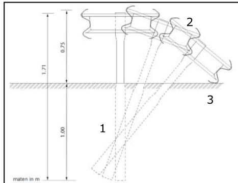
Afbeelding 2 De tweetrapswerking van een geleideconstructie
