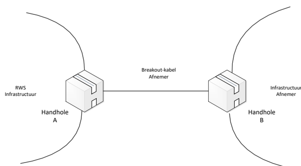
Figuur 52: Aansluitvariant Handhole
