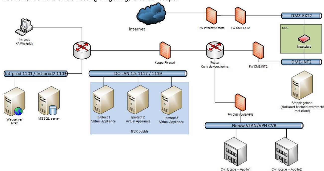
Figuur 9: Centrale omgeving iProtect en iVisit (ODC)
