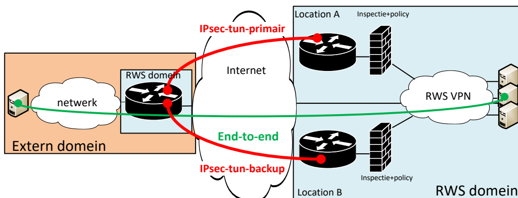
Figuur 36 - IPsec + MCPE
