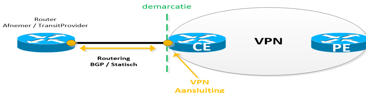
Figuur 30: Standaard routing VPN Aansluiting
