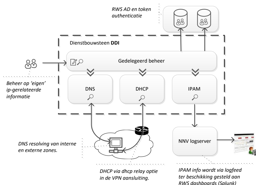
Figuur 19: onderdelen dienstbouwsteen DDI
