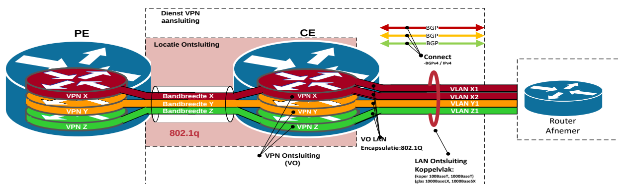
Figuur 32: Dynamische routing - VPN Aansluiting Connect
