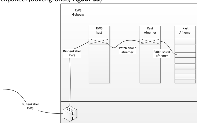
Figuur 53: Aansluitvariant Patchpaneel
