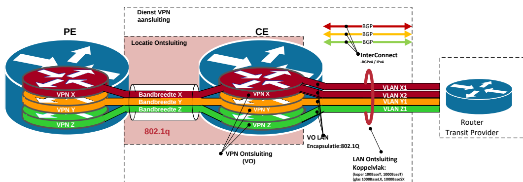
Figuur 33: Dynamische routing - VPN Aansluiting InterConnect
