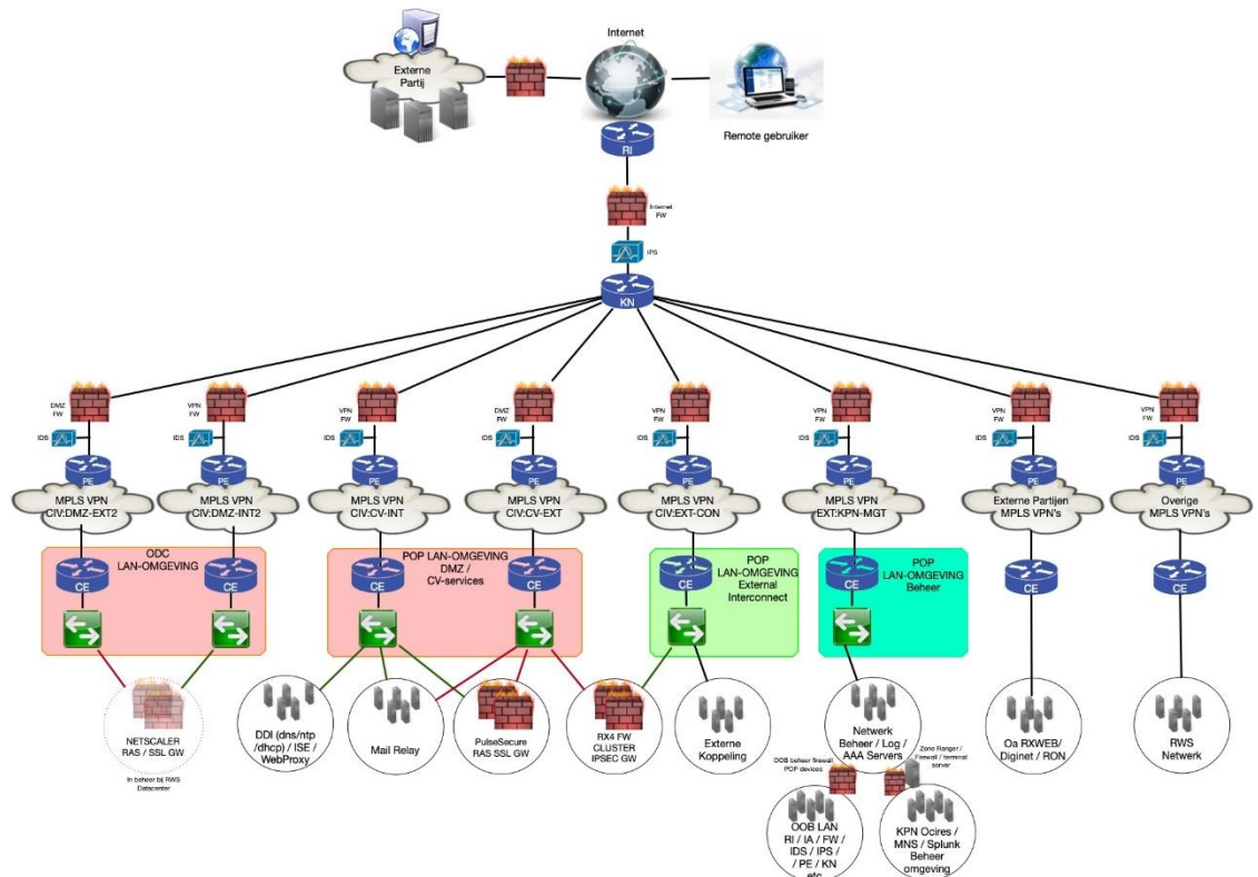
Figuur 18: samenhang dienstbouwstenen categorie VPN
