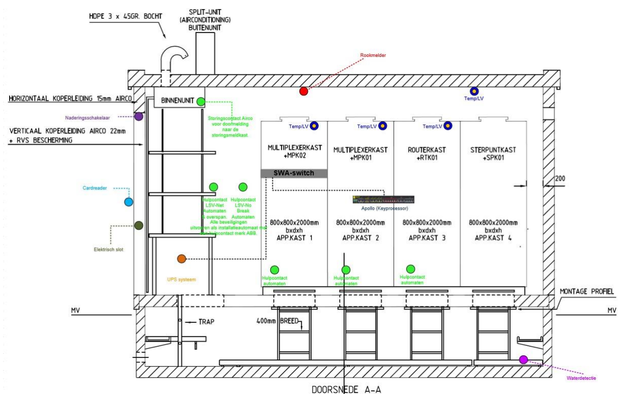
Figuur 9: Decentrale omgeving Apollo en aansluitingen (CVR)
