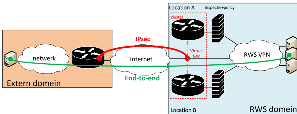
Figuur 35 - IPsec
