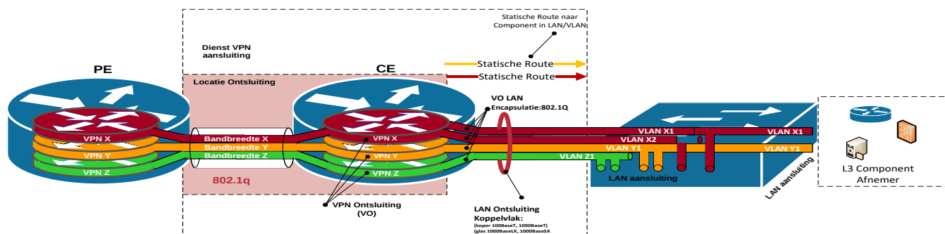
Figuur 31: Statische routing VPN Aansluiting
