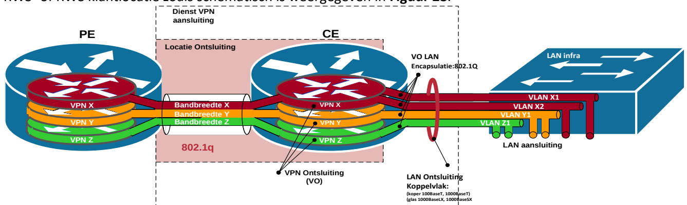
Figuur 28: Schematische weergave van de VPN aansluiting
