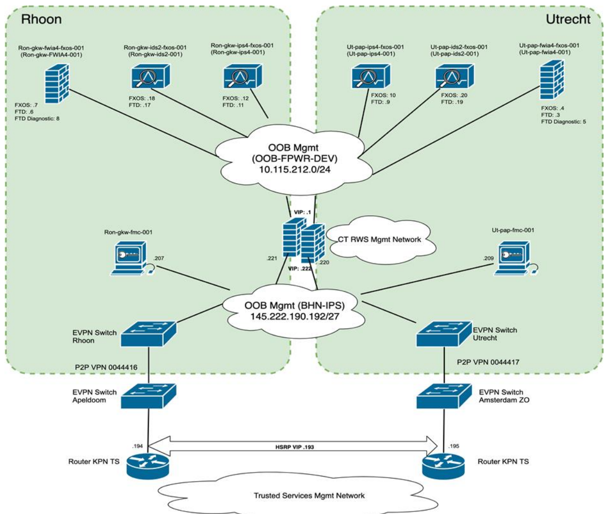
Figuur 6: Overzicht IDS-IPS
