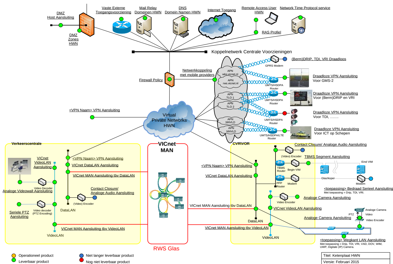
Figuur 34: Schematische weergave draadloze VPN Aansluiting
