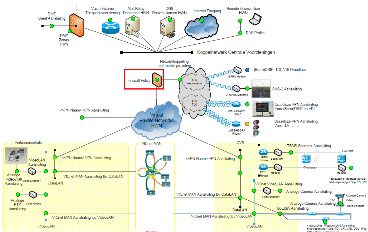
Figuur 16: Virtual Firewall overzicht
