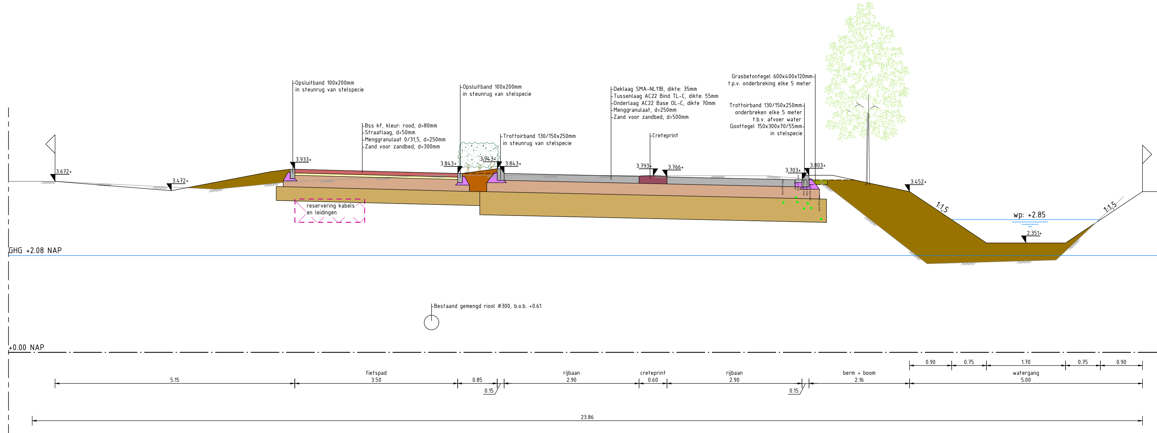
Doorsnede D-D Schaal 1:50
