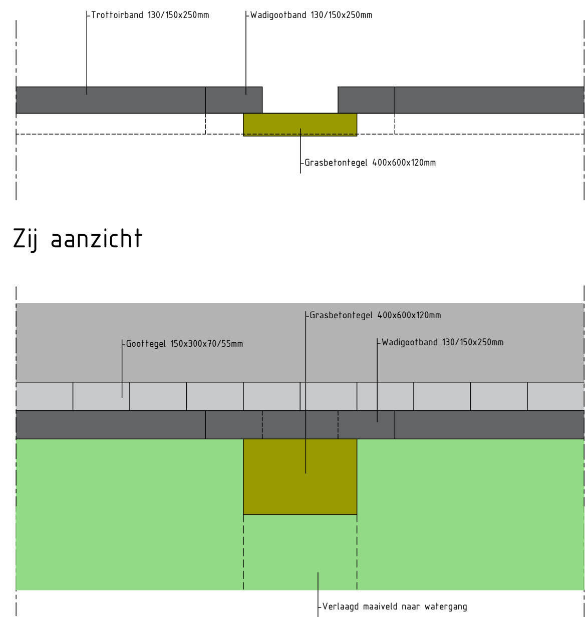
Zij aanzicht
