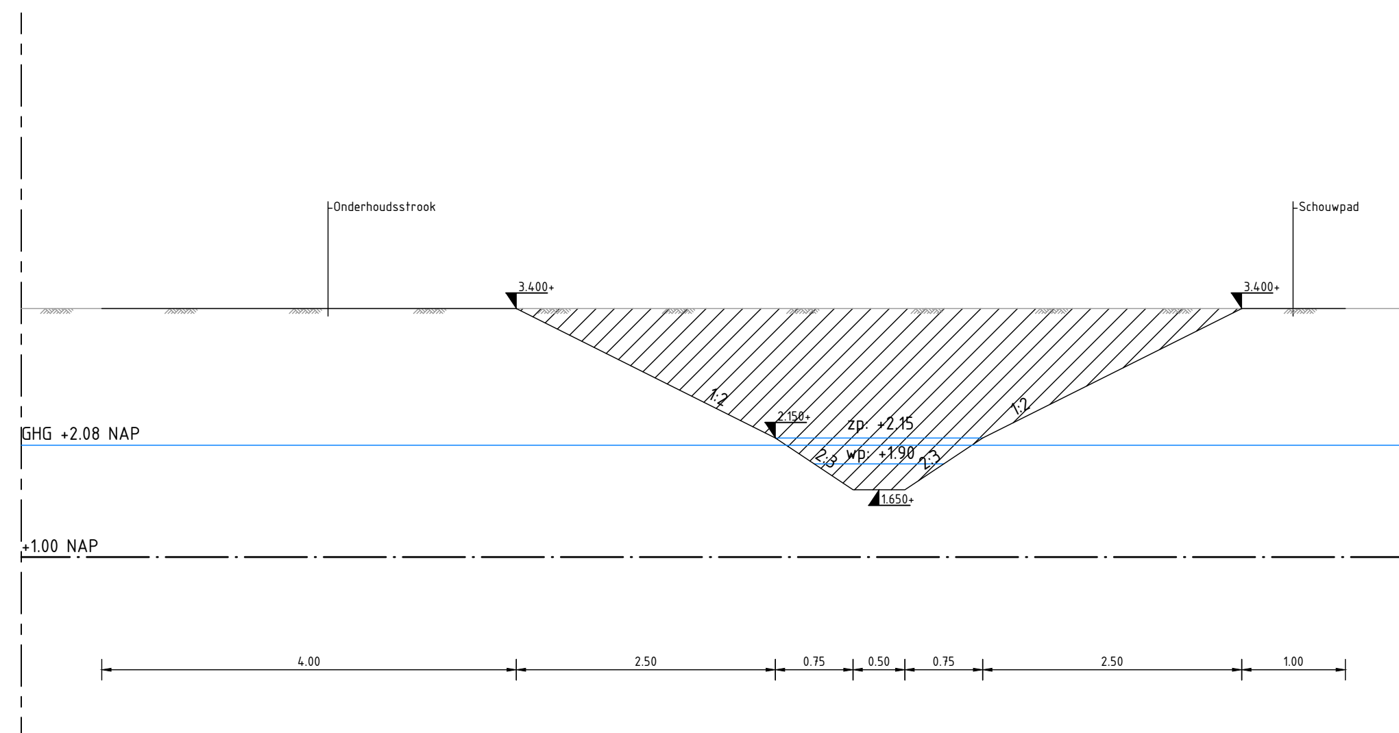
Doorsnede G-G Schaal 1:50
