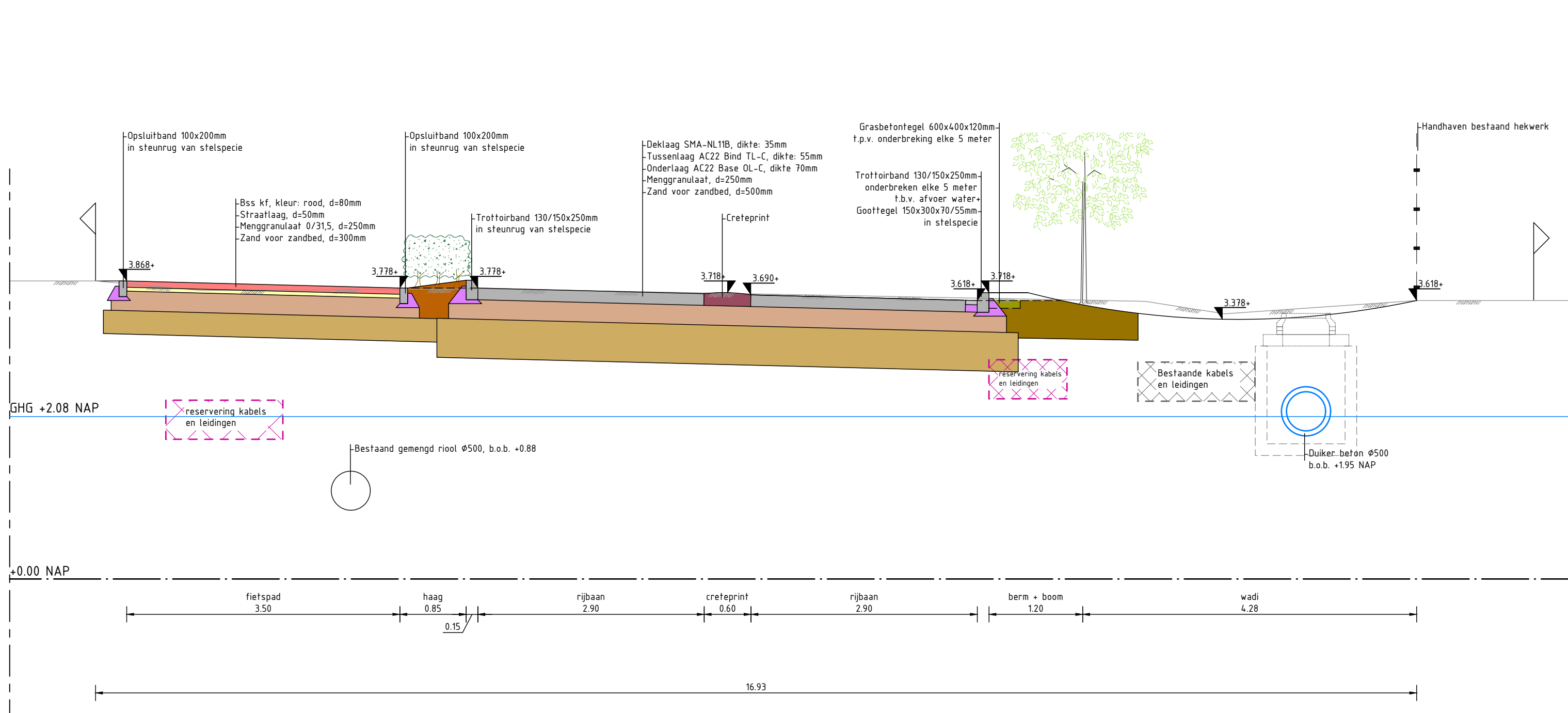
Doorsnede B-B Schaal 1:50
