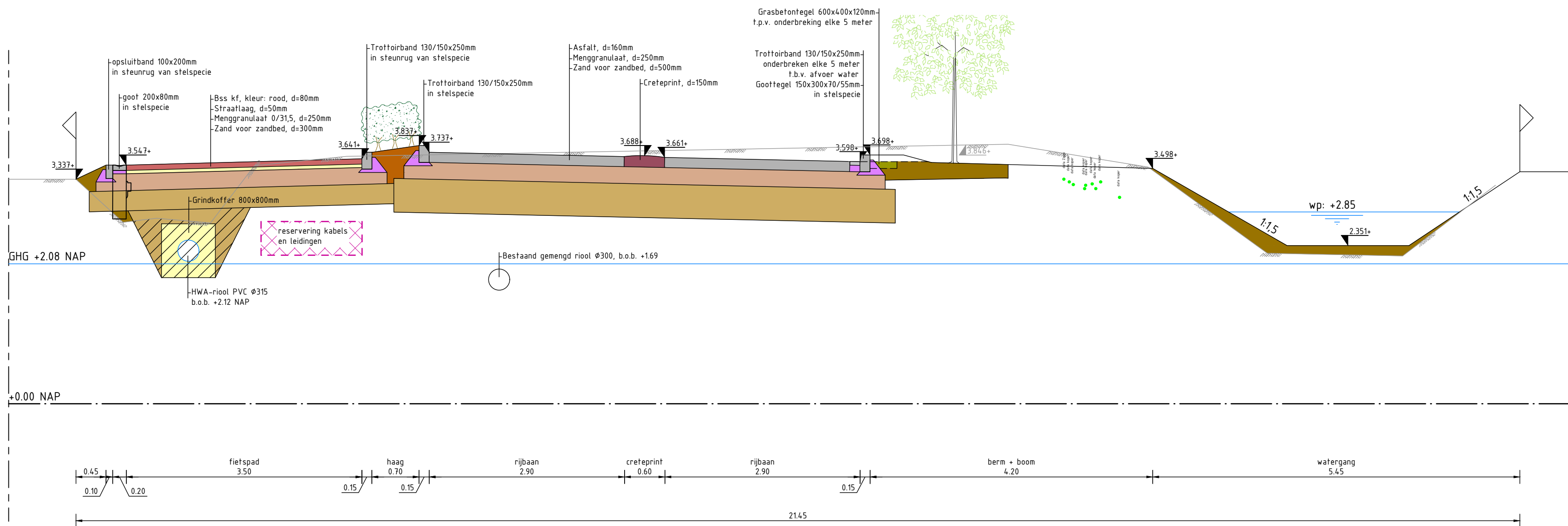
Doorsnede E-E Schaal 1:50
