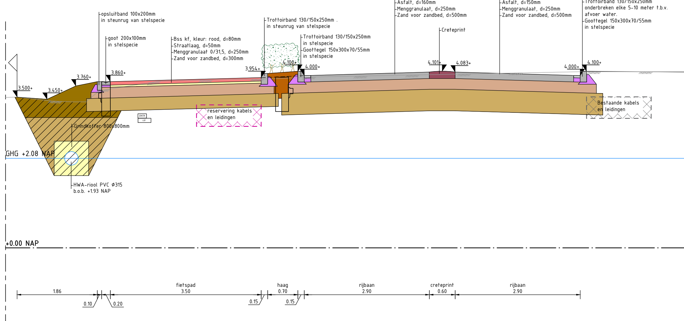
Doorsnede F-F Schaal 1:50
