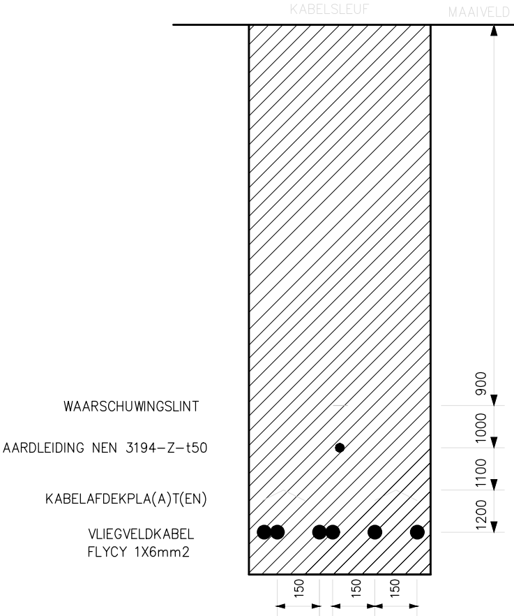
Indeling kabelsleuf buiten het defensieterrein
