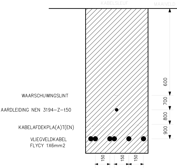
Indeling kabelsleuf binnen het defensieterrein
