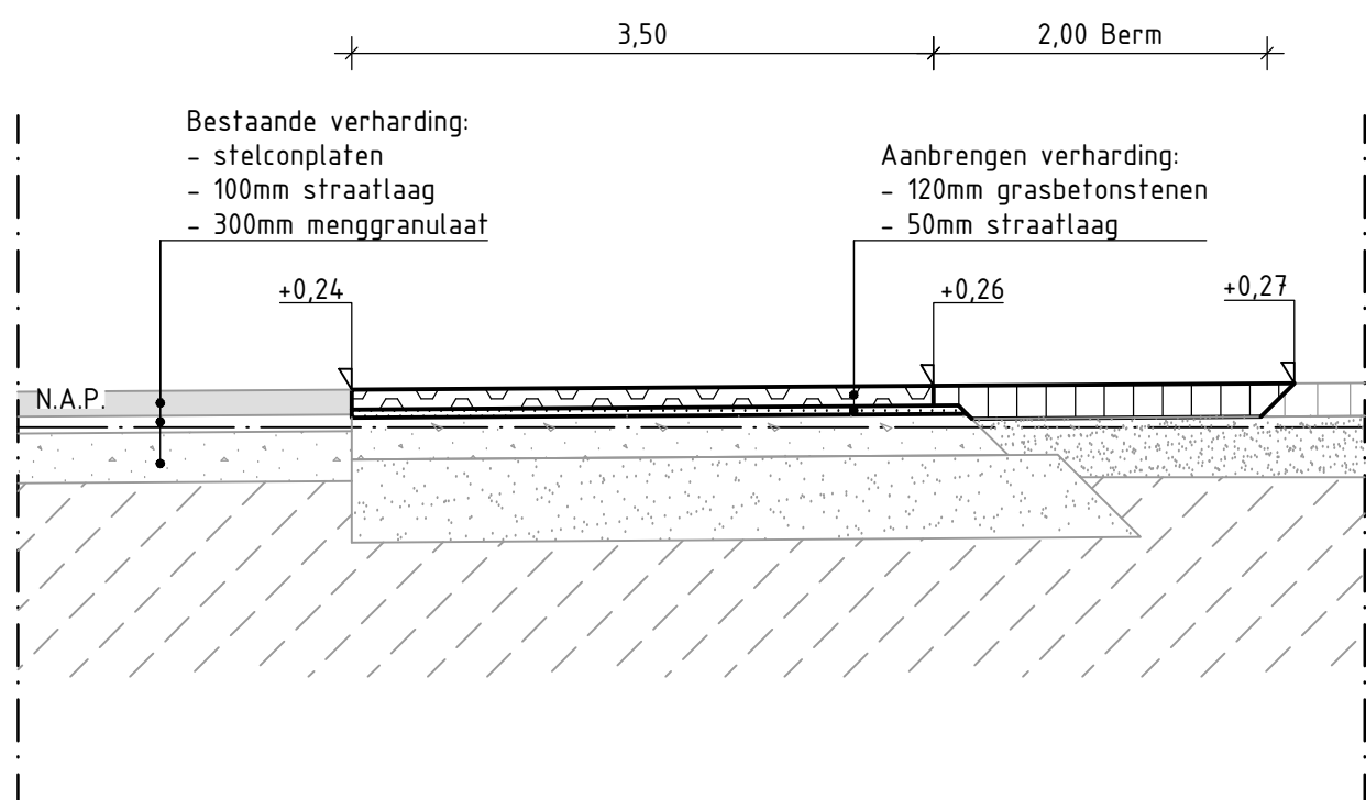
DOORSNEDE H-H - FASE 2: AANBRENGEN NIEUWE RIJBAAN
