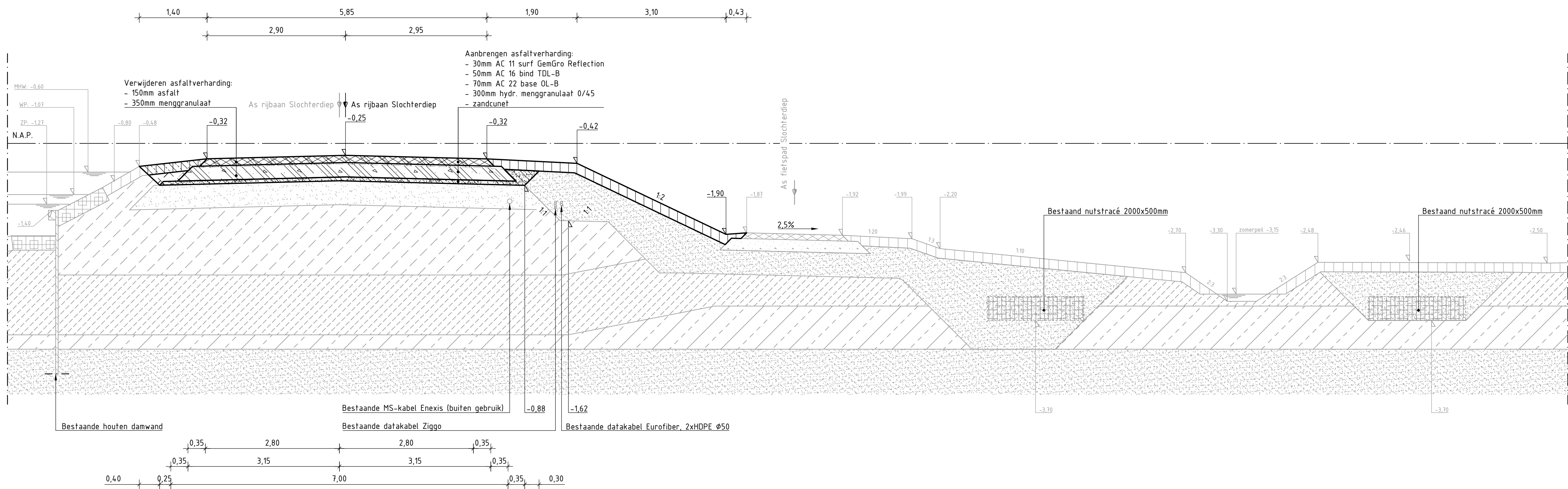
DOORSNEDE A-A - FASE 2: AANBRENGEN NIEUWE RIJBAAN
