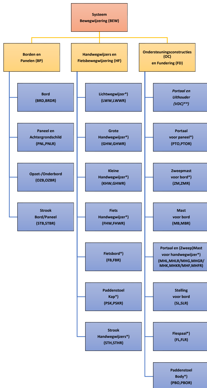
Figuur 3: Objectenboom
