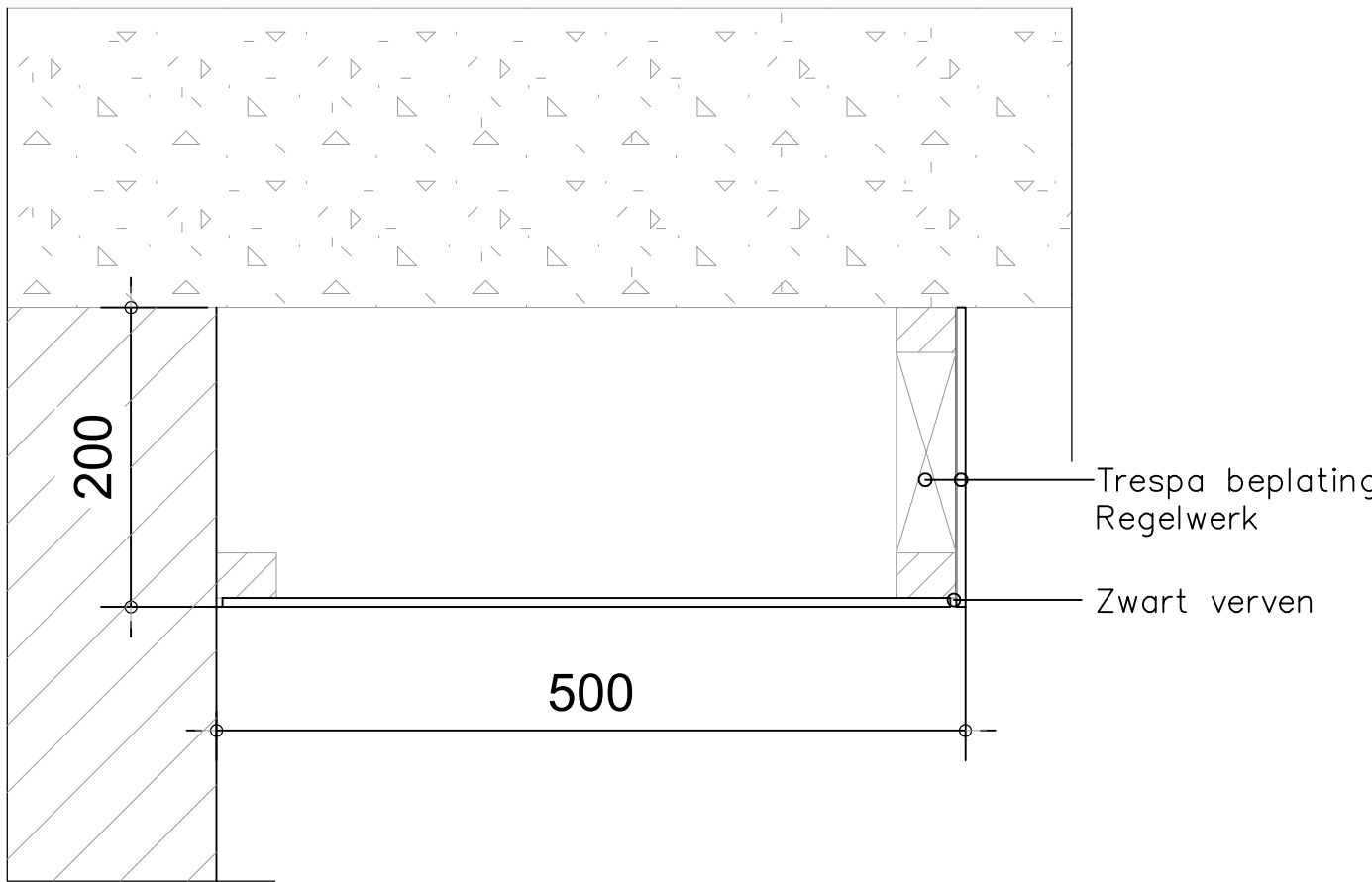
Principedetail koofaftrimmering
