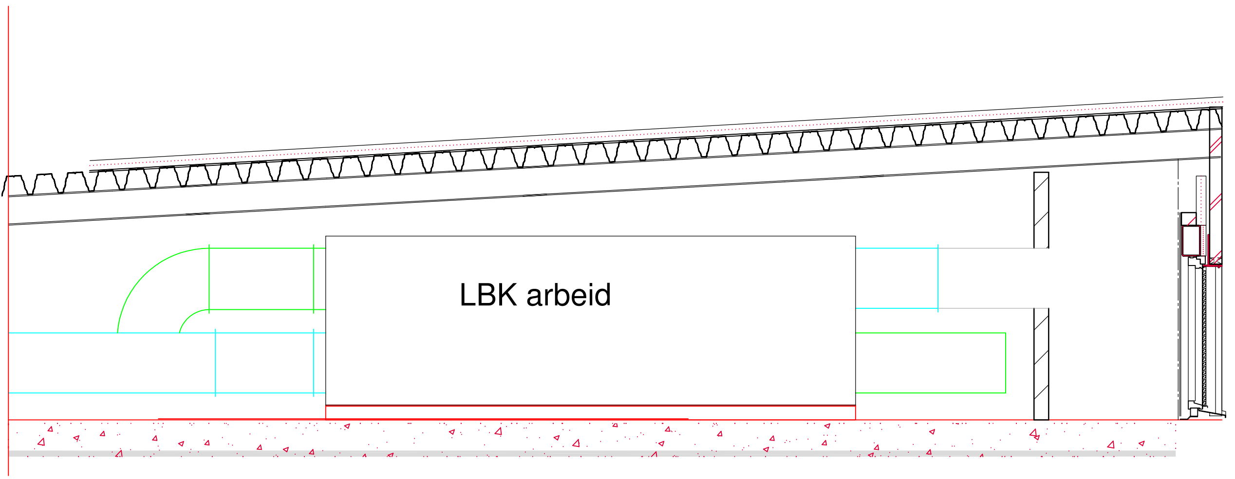
Doorsnede B-B 1:30
