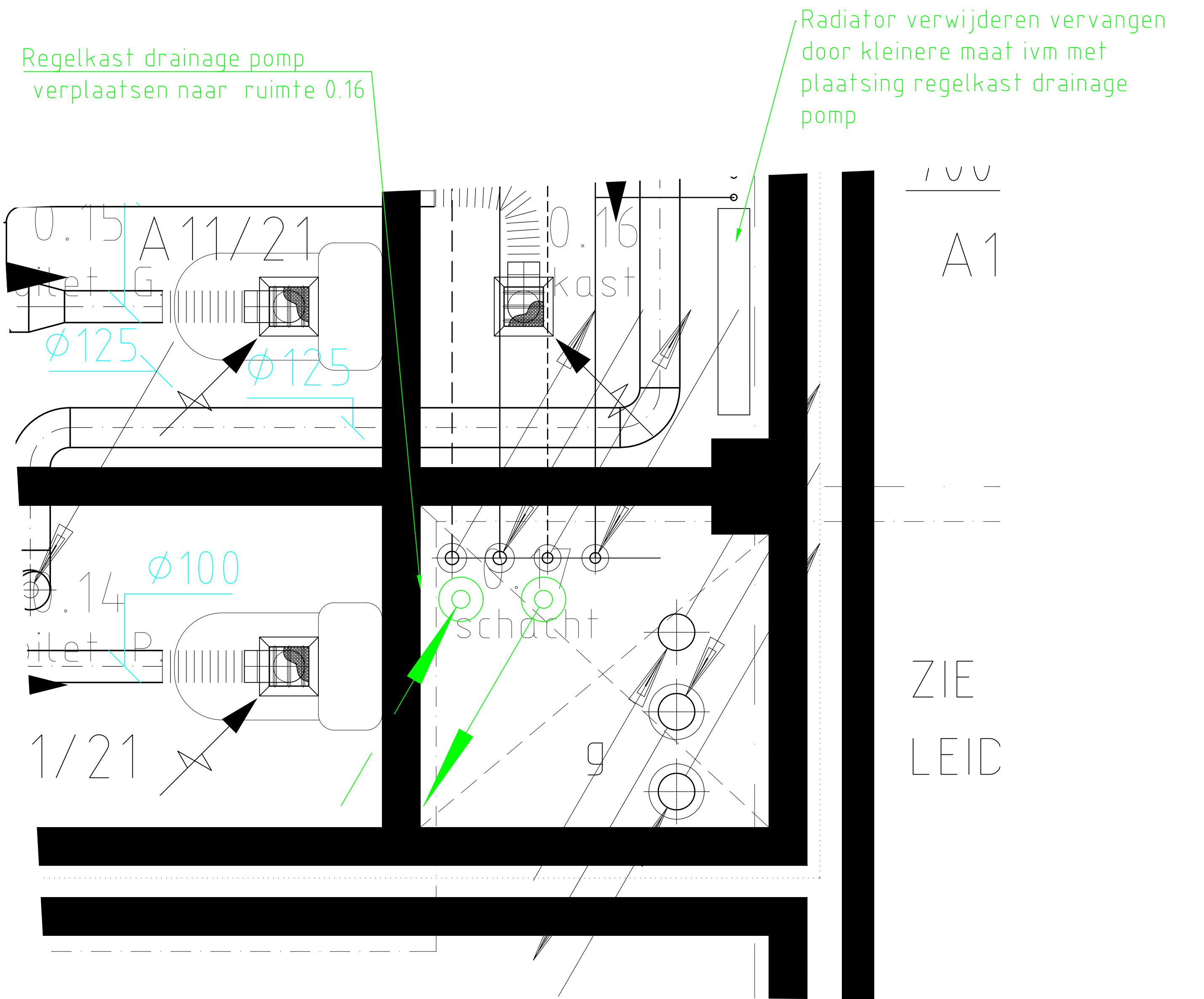
Schacht begane grond 1:10
