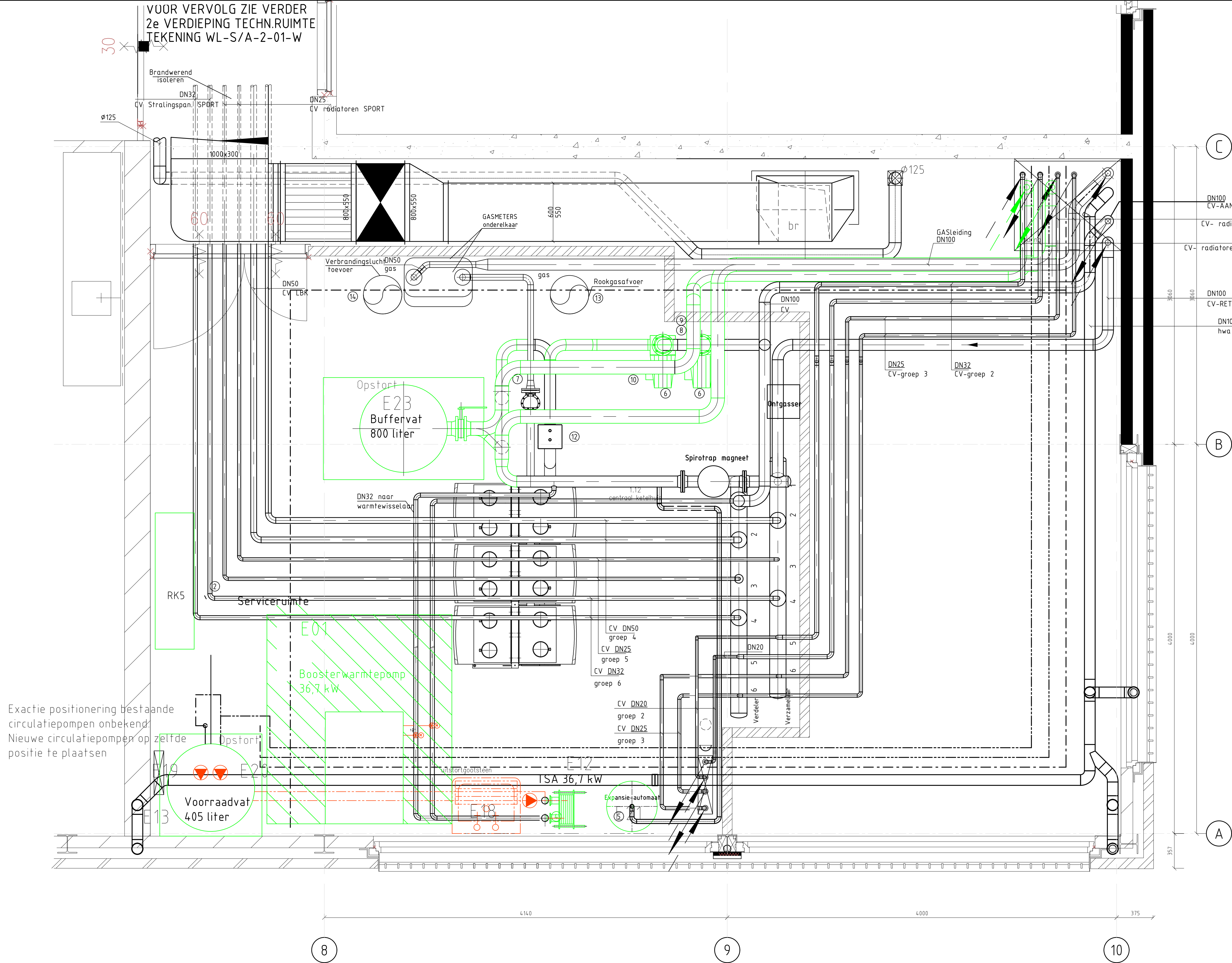
1ste verdieping technische ruimte 1:20
