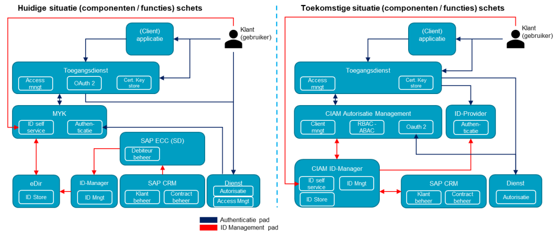
Figuur 2: Globaal logisch applicatiemodel CIAM-transitie
