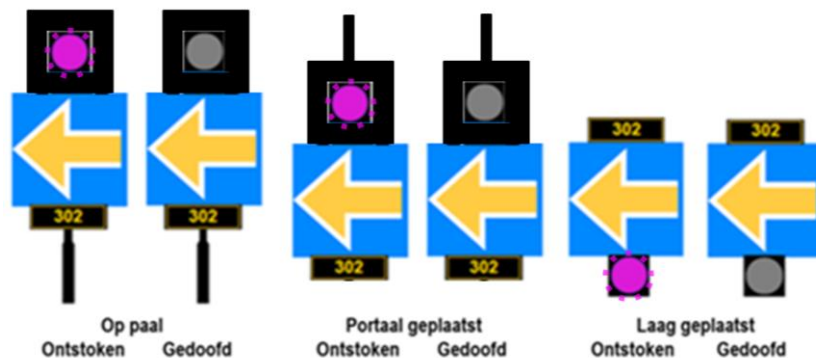
Figuur 3. Lichtbeeld Rangeerrijweg (knipper) in alle uitvoeringsvormen (met SMB en seinnummerbord)
