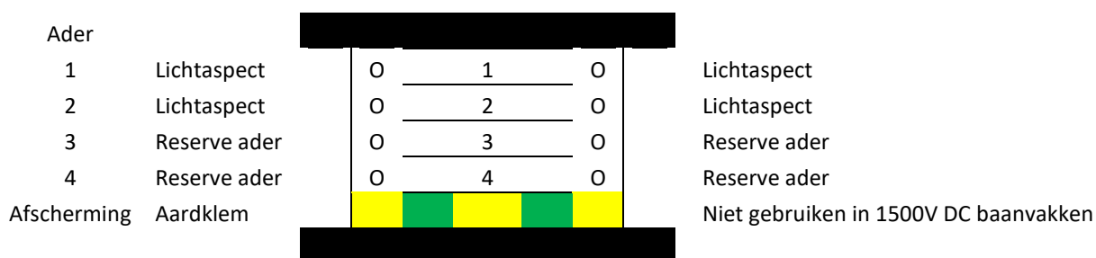
Figuur 10. Indeling klemmenstrook
