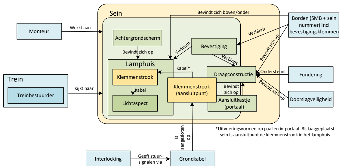
Figuur 1: Beschrijving van algemene Systeemgrenzen en scope. Geel: Te leveren (inclusief standaard objecten), Groen: Te ontwikkelen binnen levering, Blauw: Interfaces
