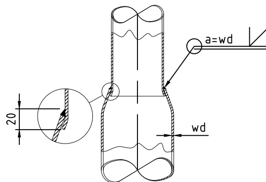
DETAIL VERLOPEN
