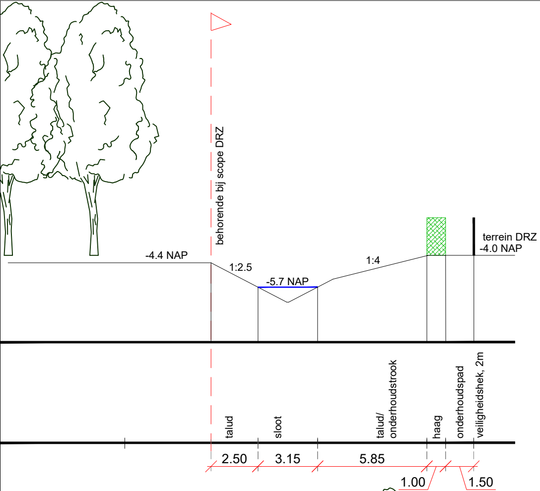
Profiel A/C t.h.v. sloot
