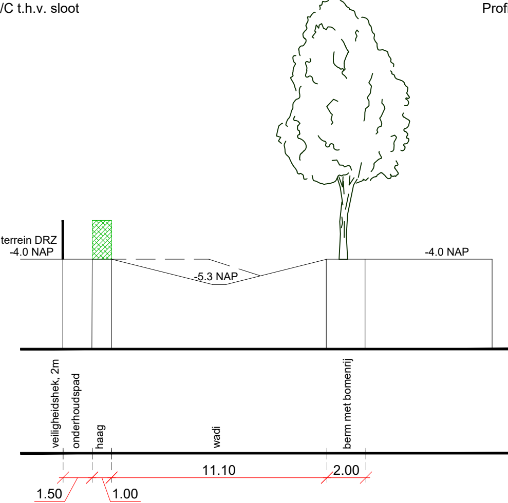
Profiel C t.h.v. gasleiding
