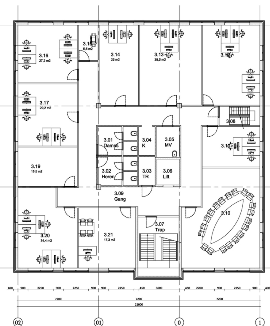
3e verdieping 10300+ bestaand
