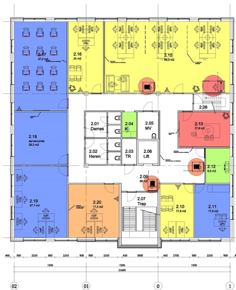
2e verdieping 7000+ nieuw
