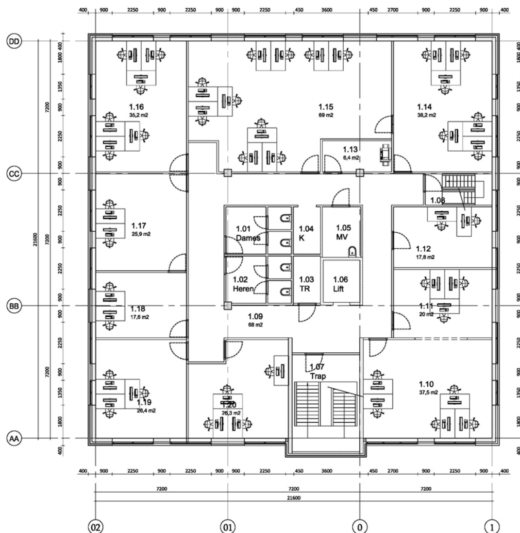
1e verdieping 3700+ bestaand
