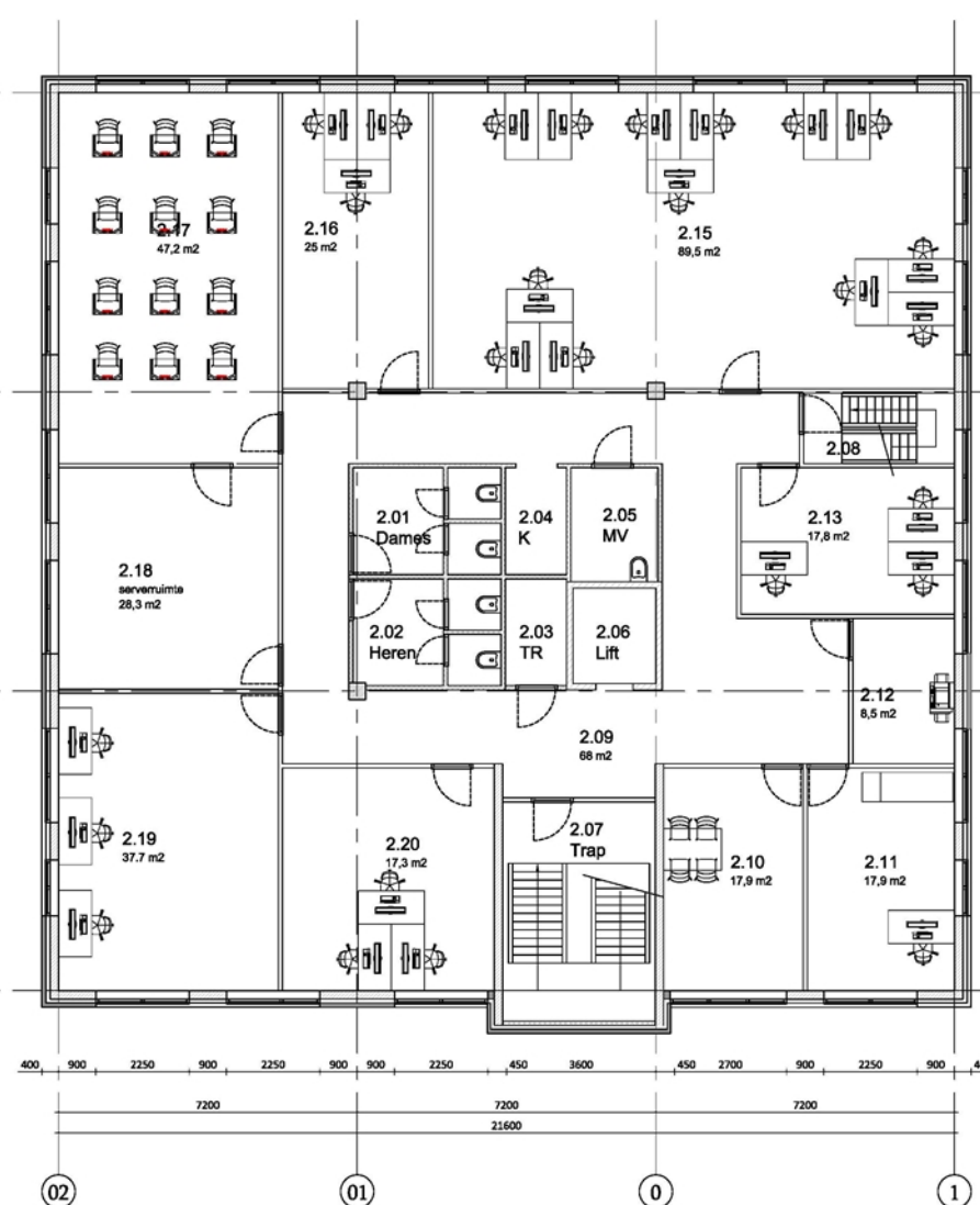
2e verdieping 7000+ bestaand
