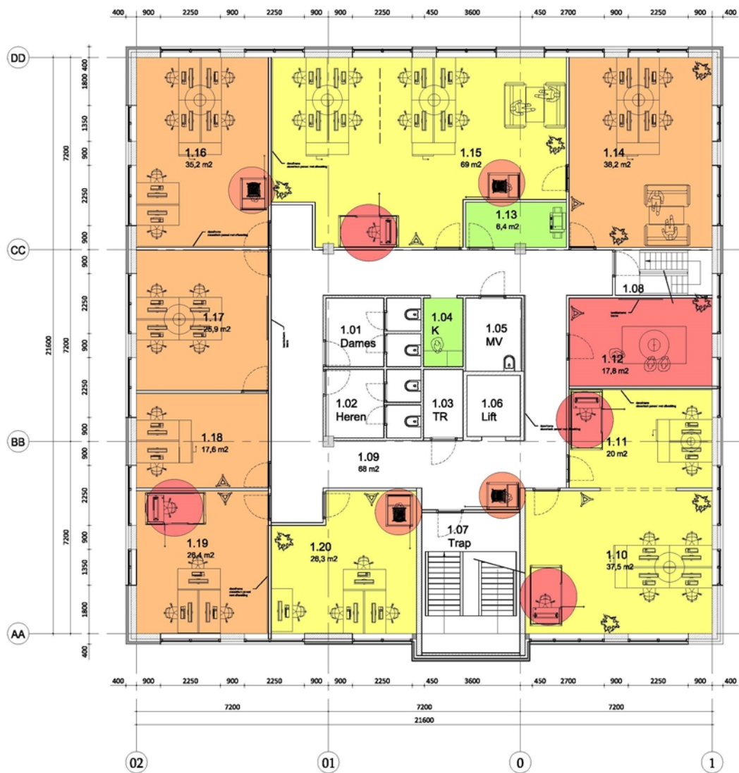
1e verdieping 3700+ nieuw
