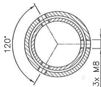
Doorsnede A-A.
