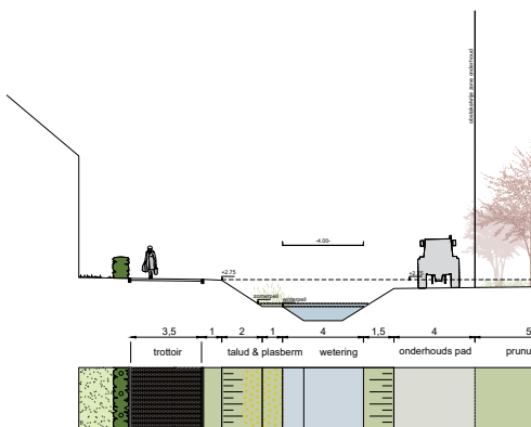
Doorsnede K
