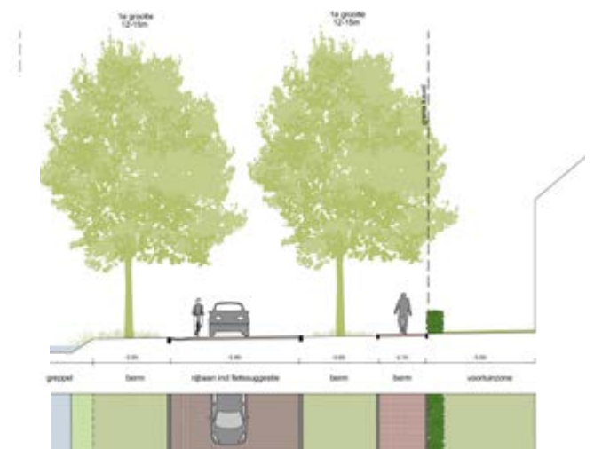
Doorsnede B
