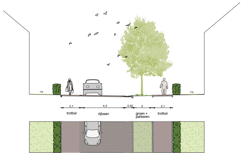
Doorsnede D
