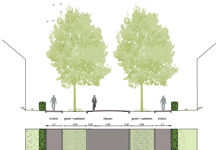
Doorsnede C
