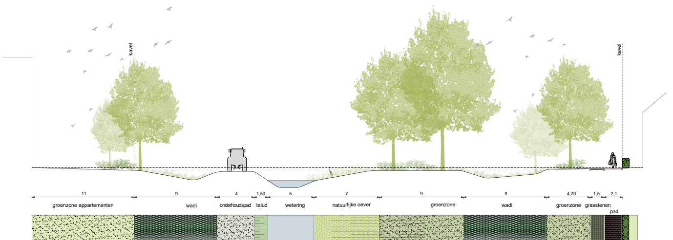
Doorsnede I
