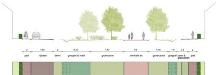
Doorsnede J
