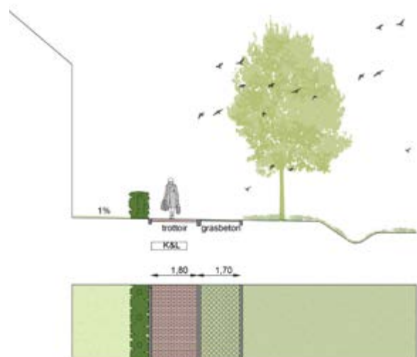
Doorsnede G
