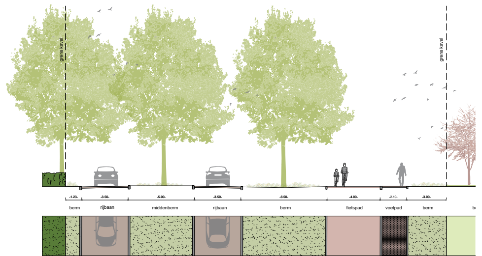
Doorsnede A
