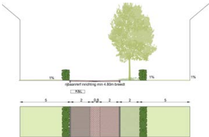
Doorsnede H
