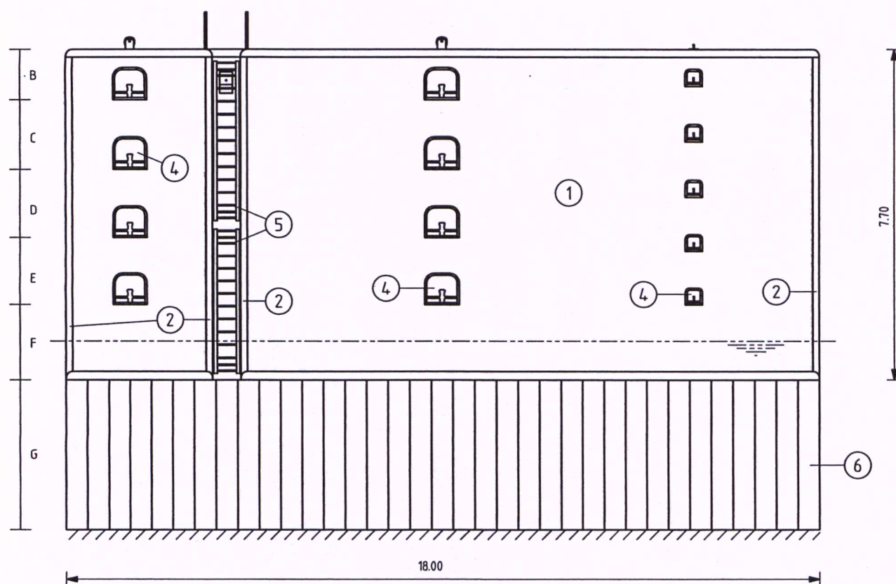
VOORAANZICHT
