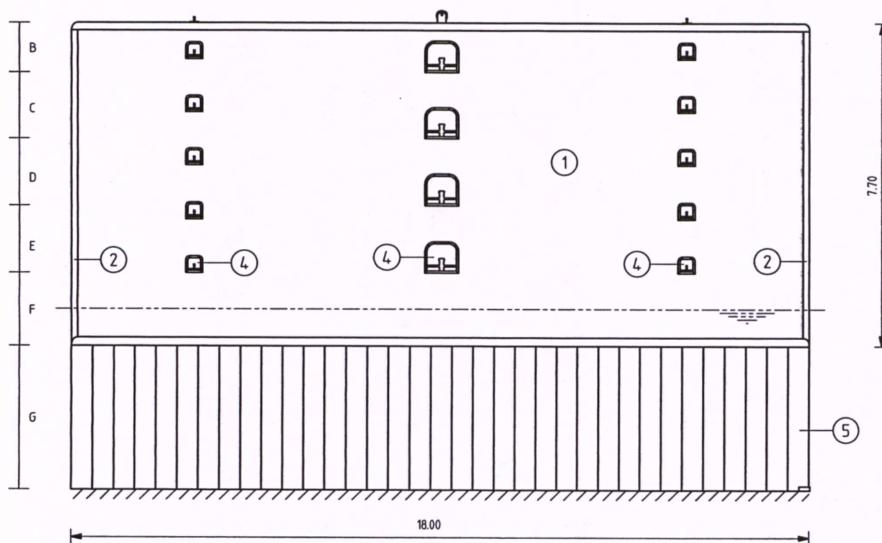
VOORAANZICHT
