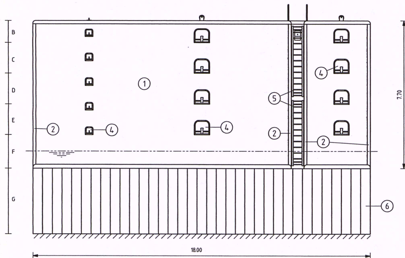
VOORAANZICHT
