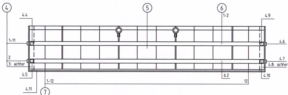
SCHOTBALK 1 EN 2
