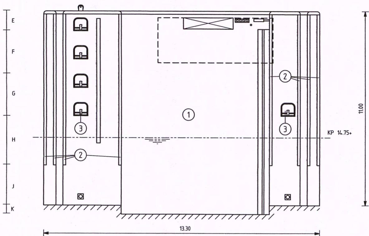
VOORAANZICHT
