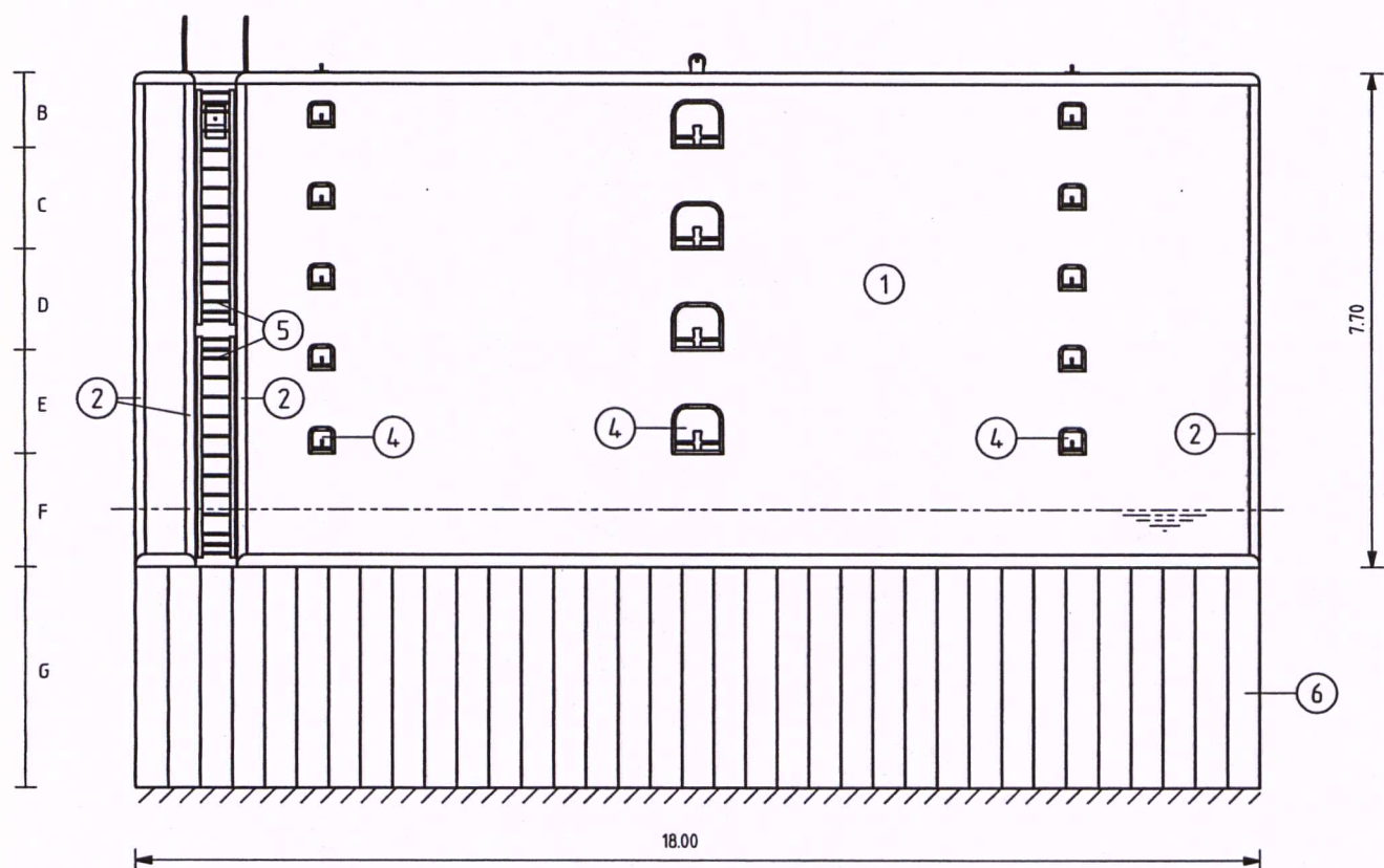
VOORAANZICHT
