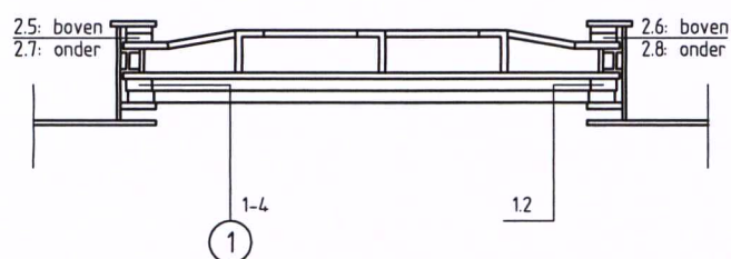
DOORSNEDE B-B
