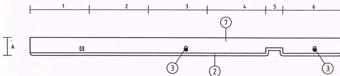
BOVENAANZICHT
