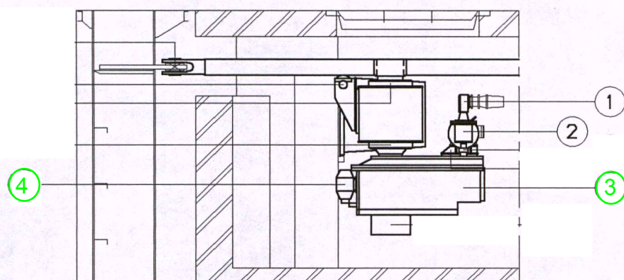
Aanzicht A-A
