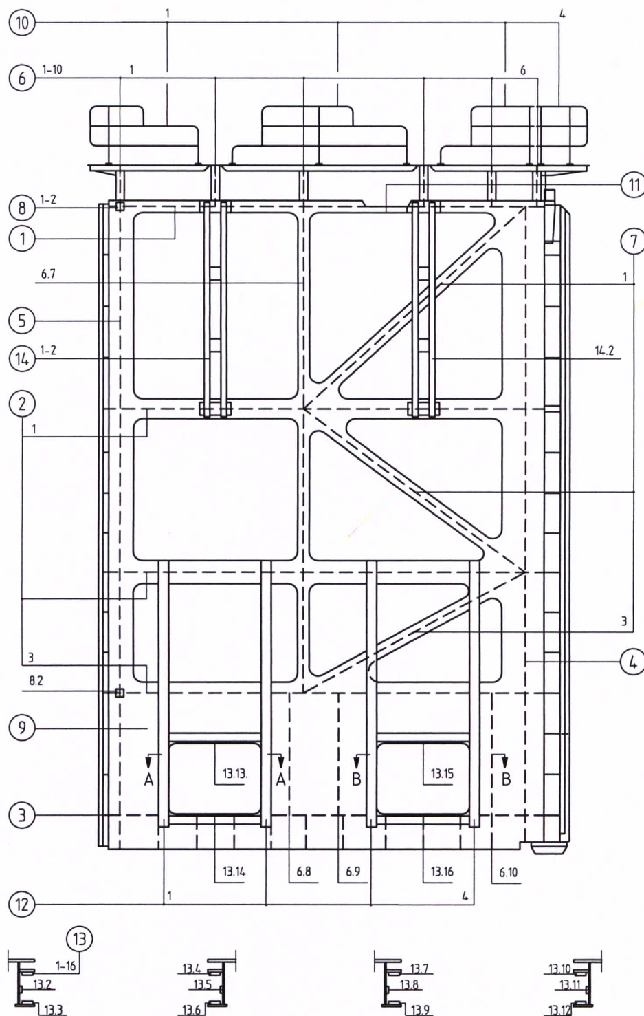
DOORSNEDE A-A
