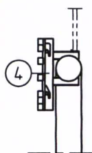
DOORSNEDE
