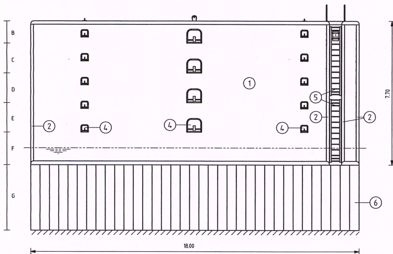
VOORAANZICHT
