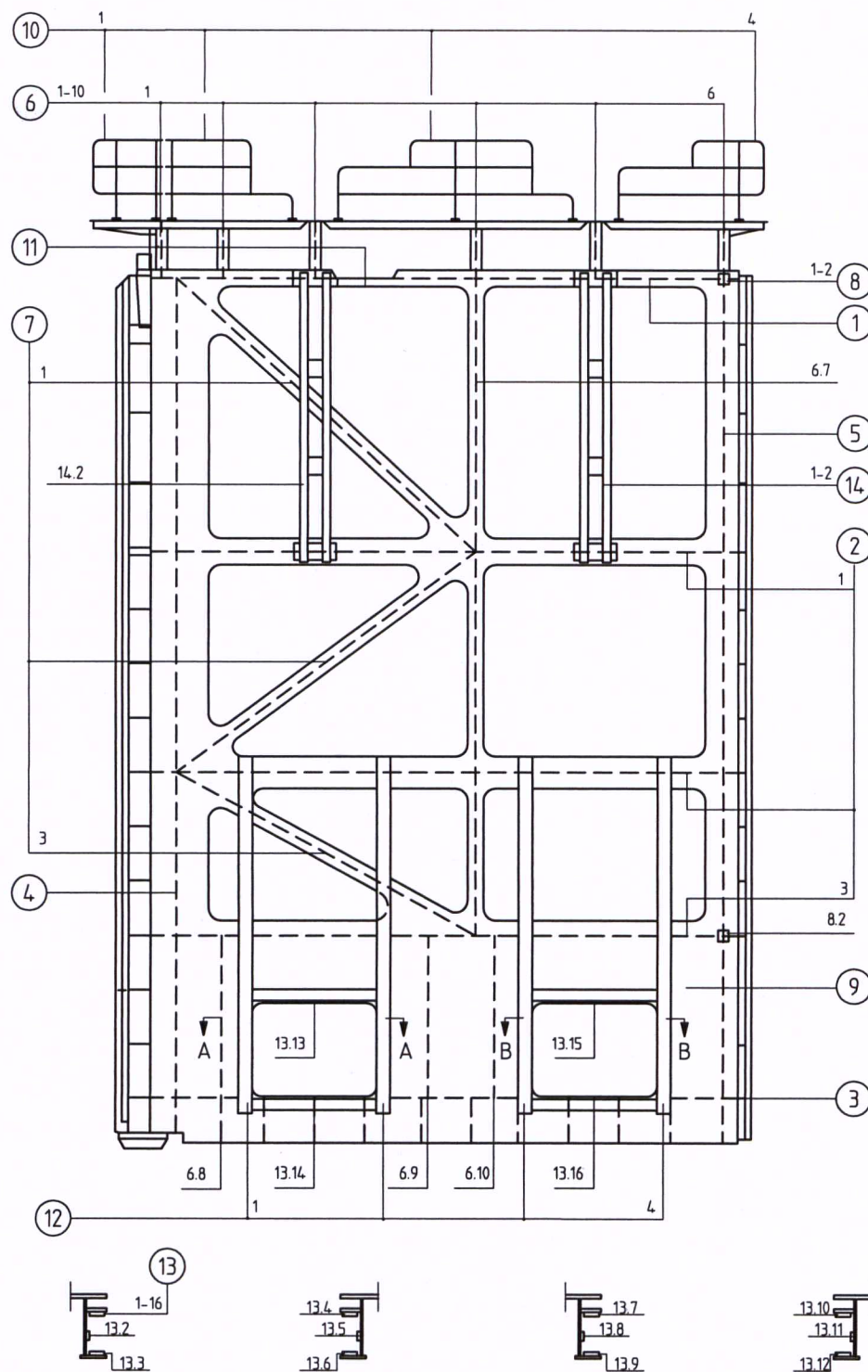
DOORSNEDE A-A
