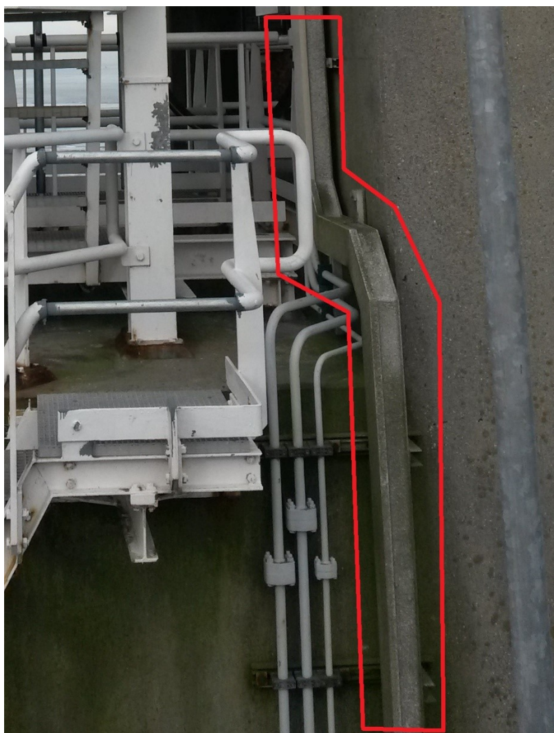
OBT-00037 Kabel en kabelgoot op de pijler
