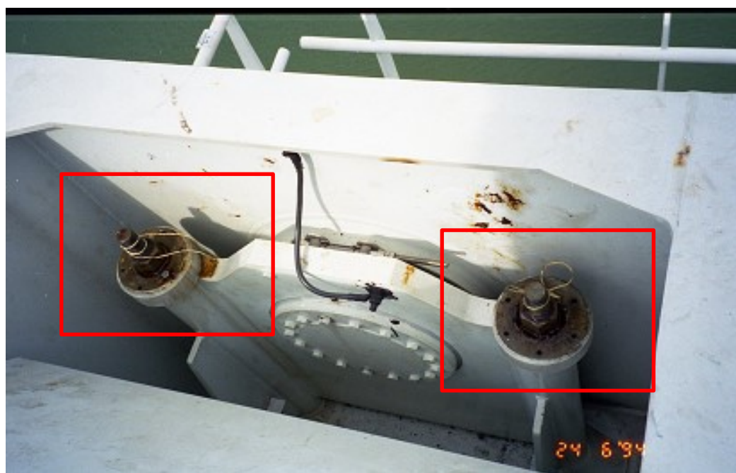
OBT-00126 Cardanstoelankerstang en moeren M48,M56
