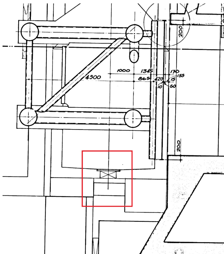
OBT-00023 Pijlersponningoplegvlak
