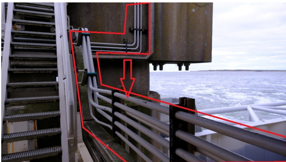
OBT-00098 Hydrauliekleidingen van de EH-eenheid
