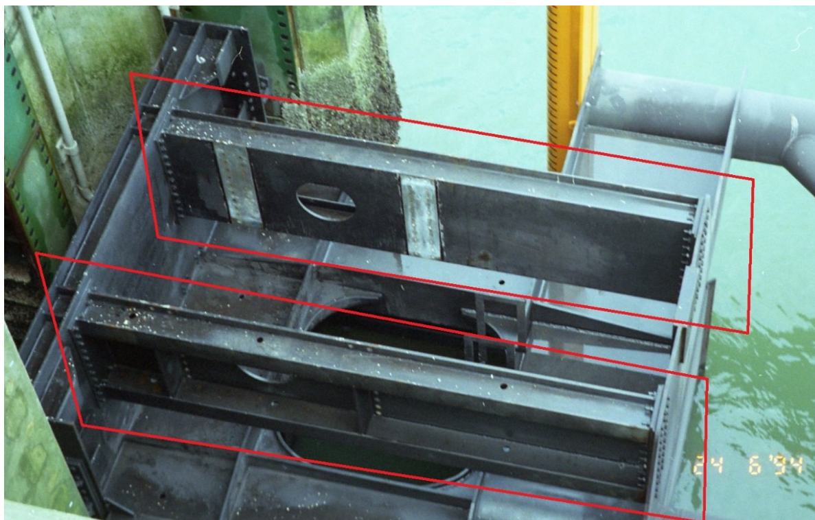
OBT-00114 Schuifophangbalk ( waar de overgangsconstructie van het onderoog aan vast zit)
