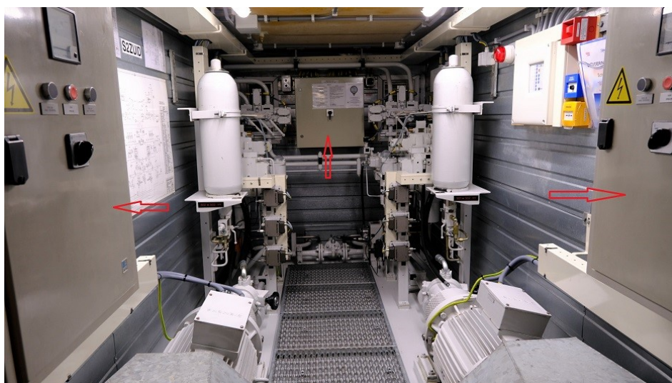
OBT-00097 E-voedingseenheid( regeling en bew) in de container van de EH-eenheid
