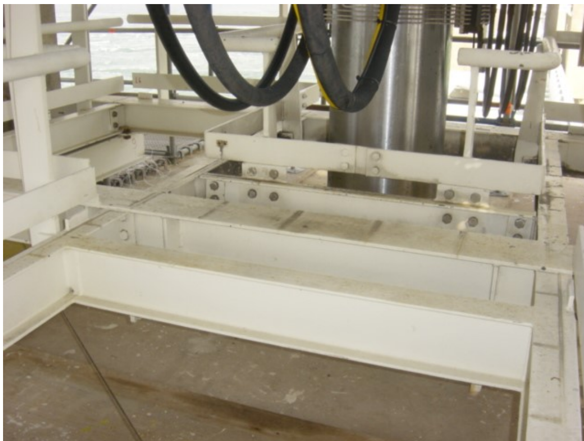
OBT-00032 draagconstructie van het bordes op de pijler
