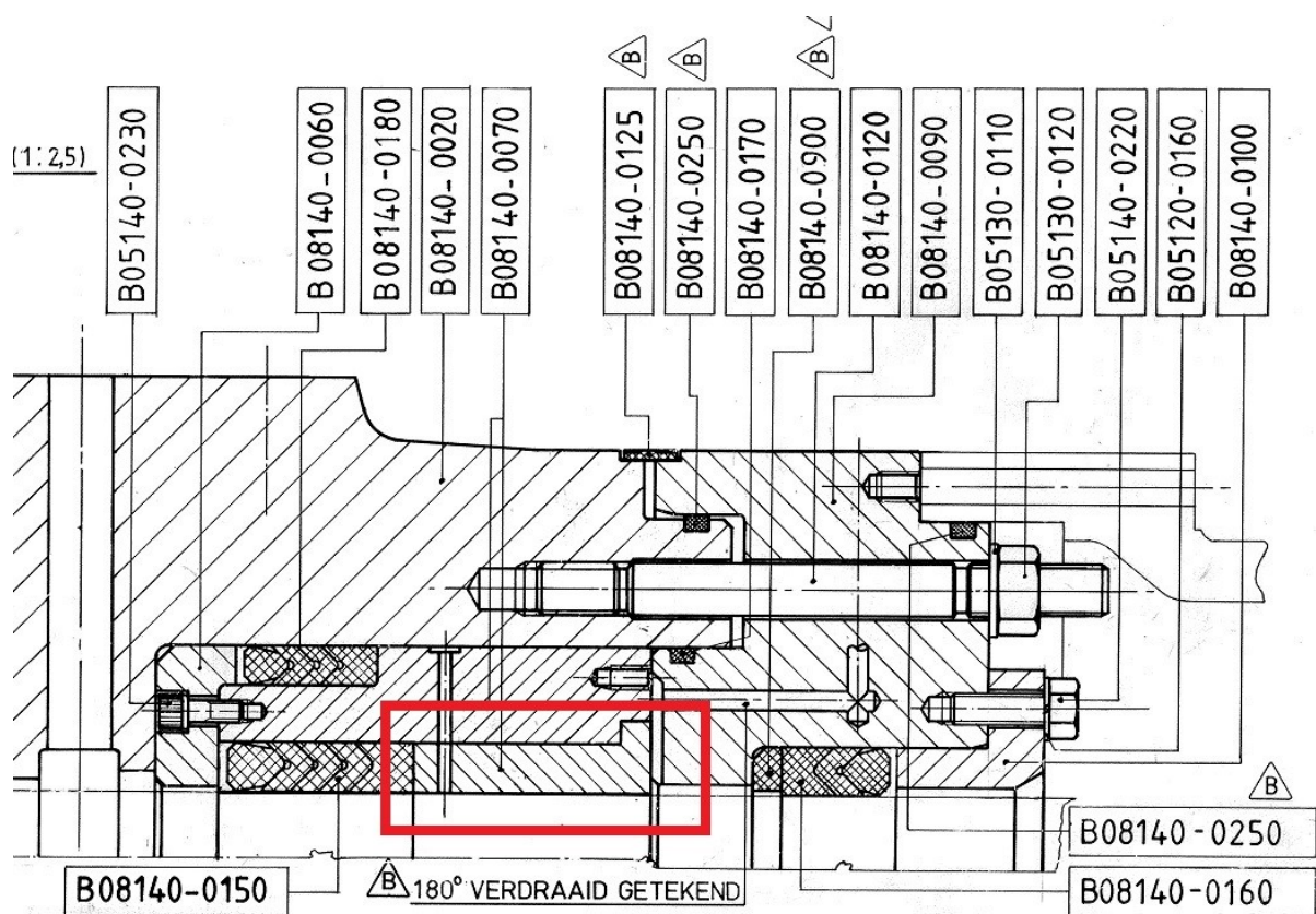
OBT-00062 geleidebus van het lantaarnstuk
