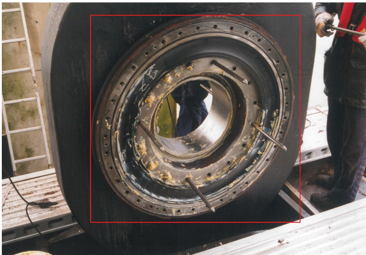
OBT-00082 Onderooglagerafdichting
