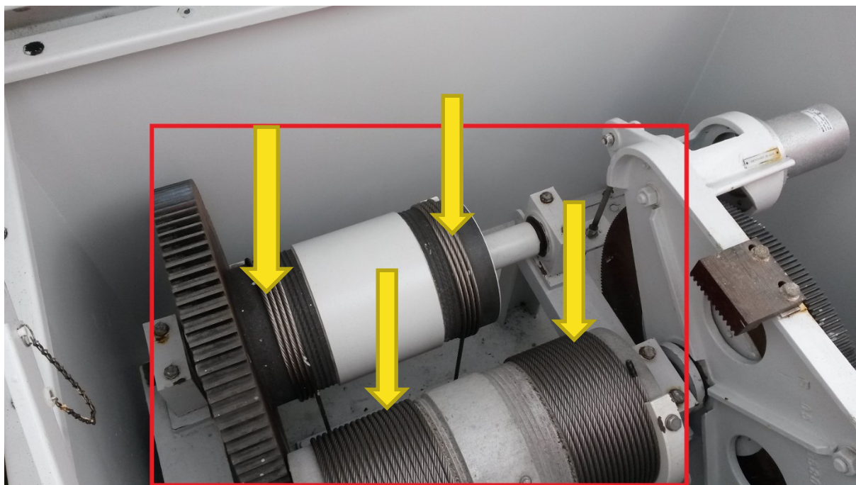
OBT-00108 Staalkabel van de gelijkloopinstallatie
