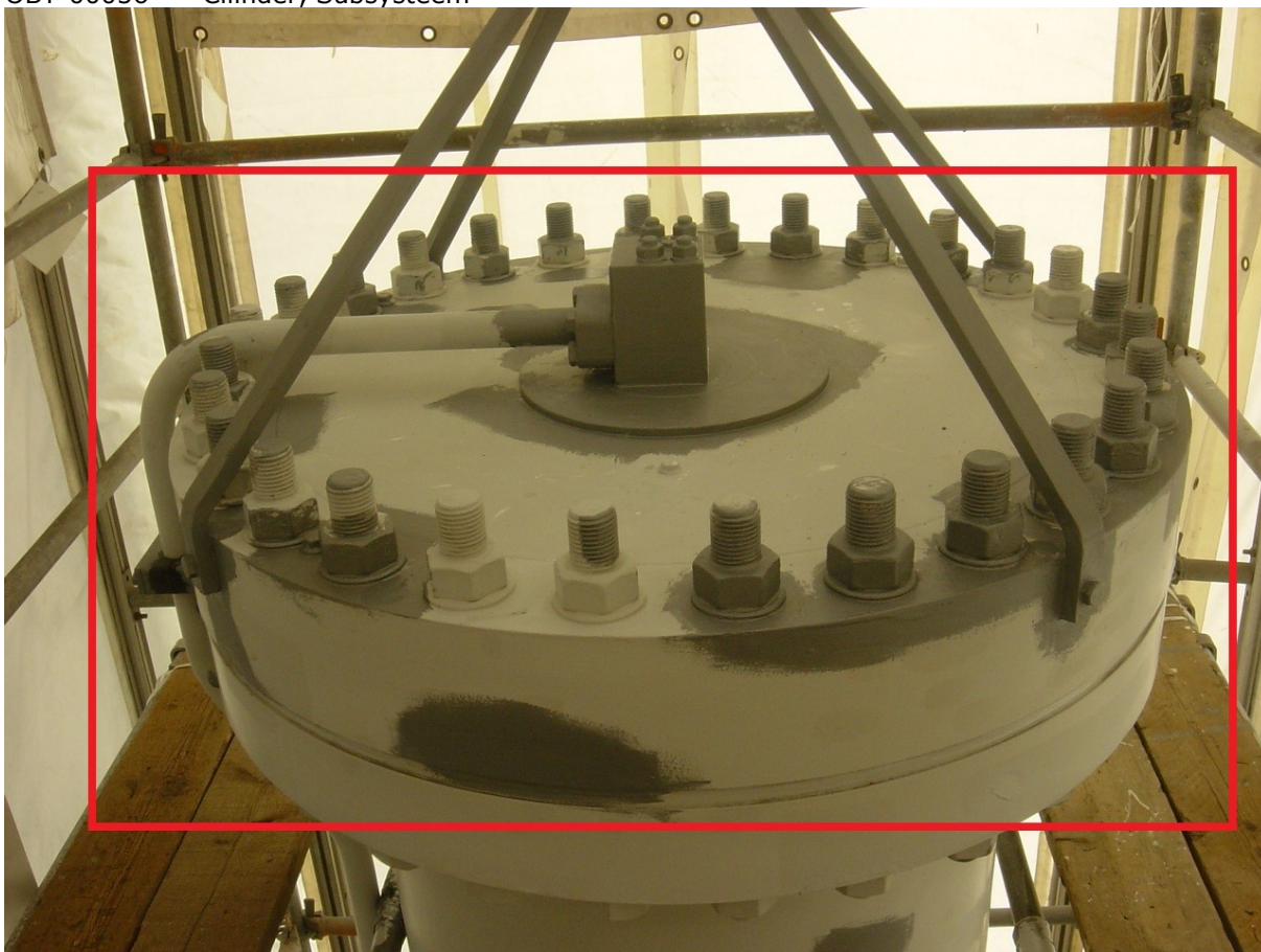
OBT-00057 Cilinderdeksel
