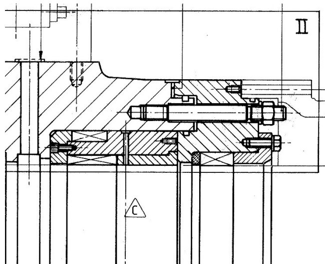
OBT-00133 Lantaarnstuk Pakkinghouder
