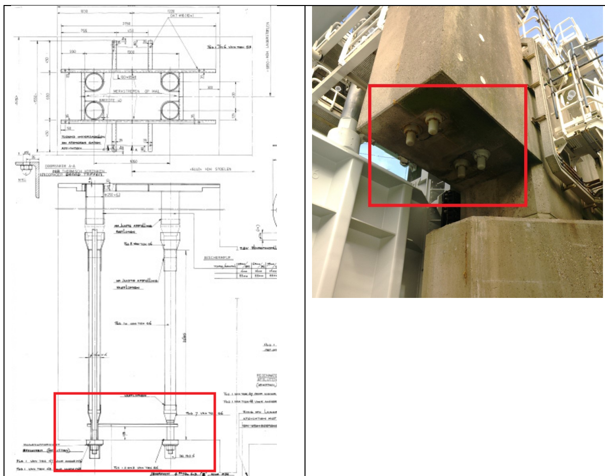
OBT-00026 Pijlerhamerstukonderframe
