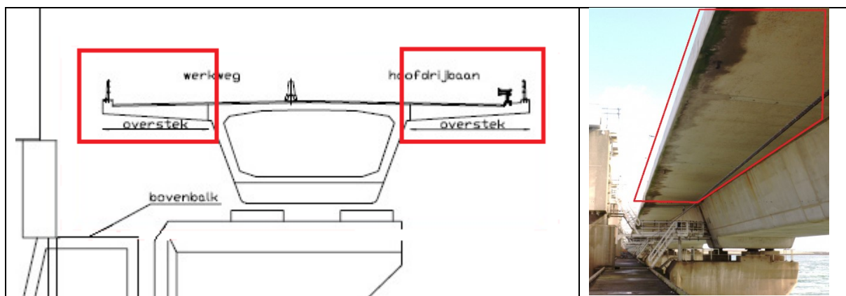
OBT-00006 Uitkragingen
