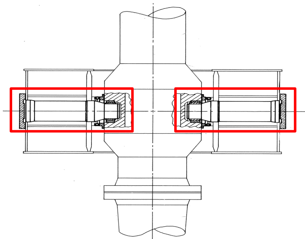
OBT-00045 Cardanbalkscharnierpen naar de cilinder, Substysteem
