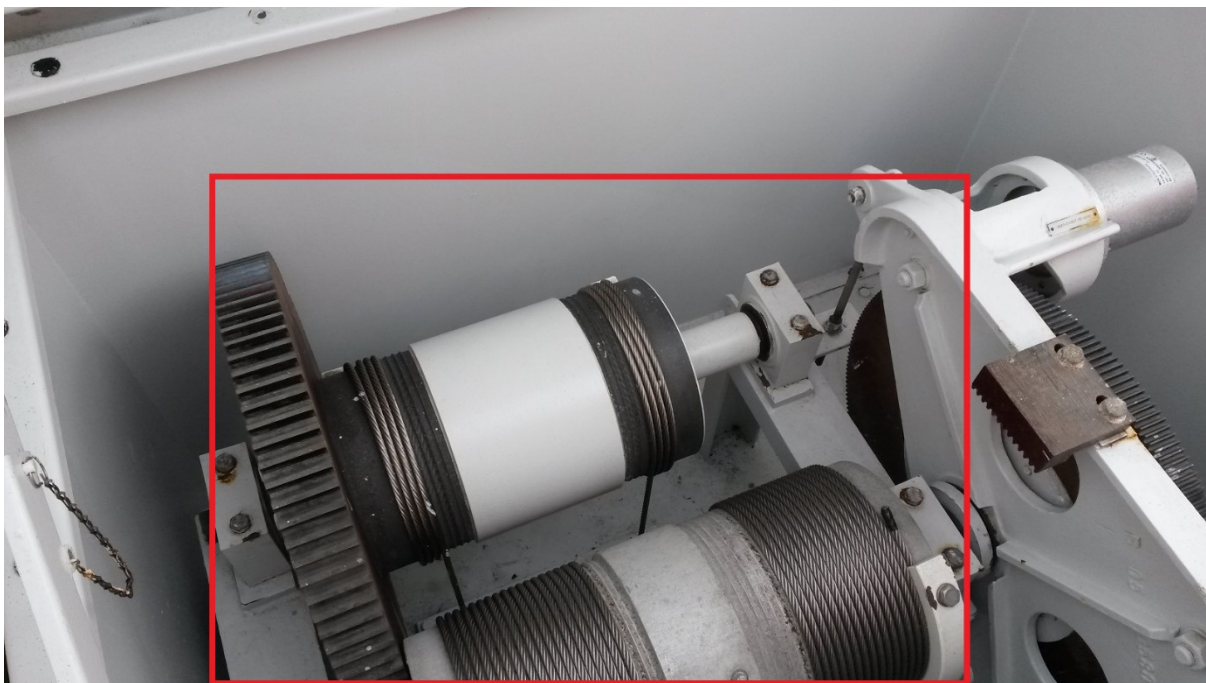
OBT-00106 Kabeltrommel van de gelijkloopinstallatie
