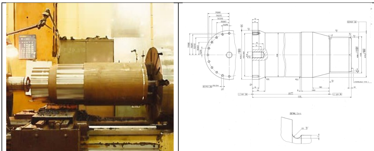
OBT-00124 Cardanbalkscharnieren naar Cilinder
