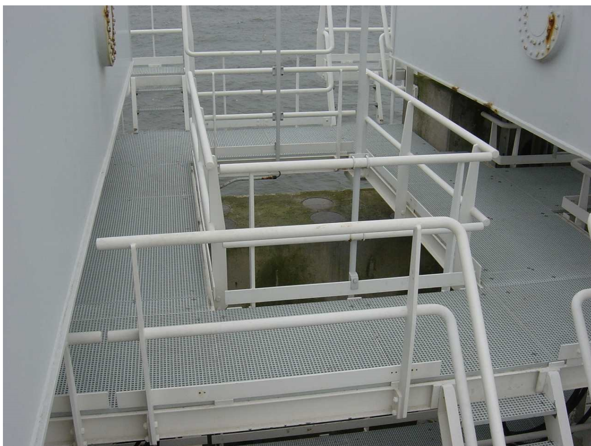
OBT-00031 Pijlerbordes
