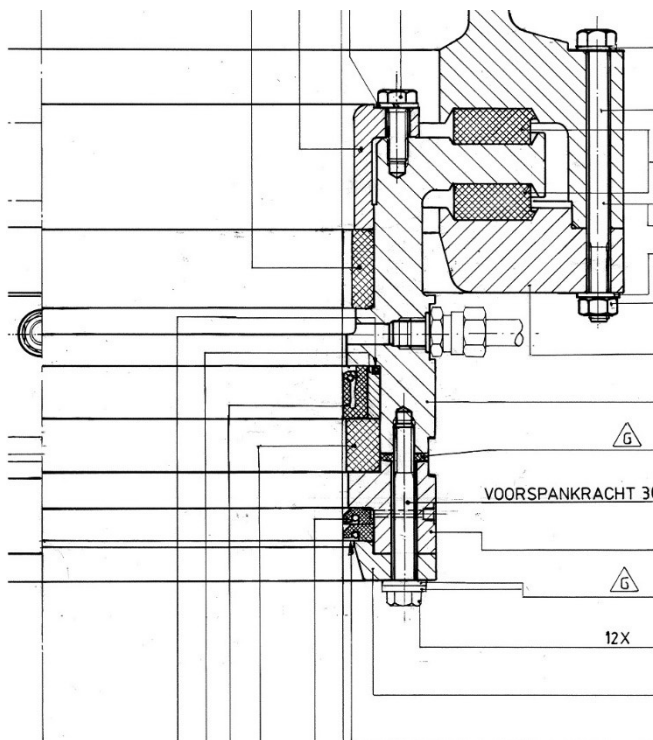
OBT-00140 Conserveringsolie-ruimte afdichting met zuigerstang
