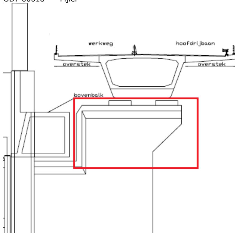
OBT-00019 Pijlerkop
