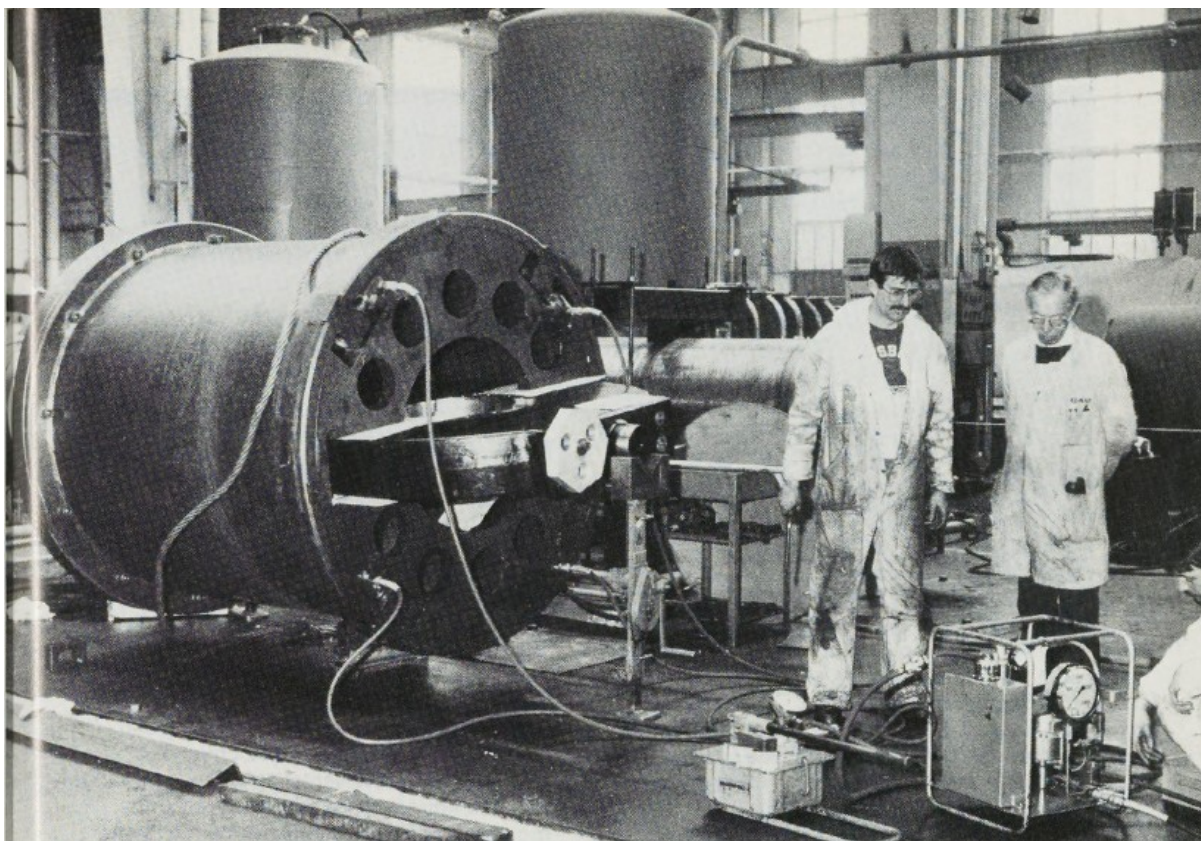
OBT-00077 Onderoog-hulpgereedschap om de zuigerstang te monteren
