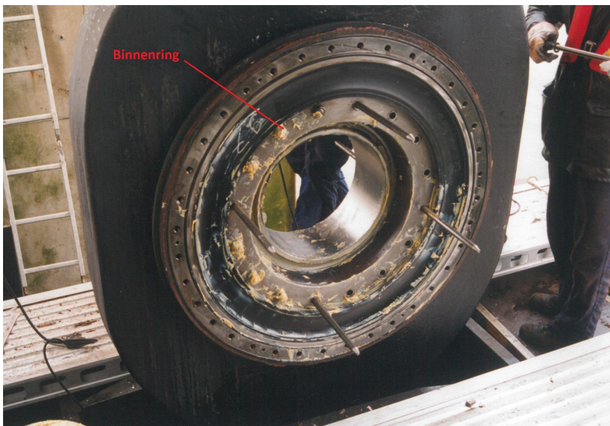
OBT-00085 Binnenring van de onderooglagerafdichting
