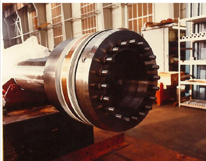
OBT-00067 Zuigergedeelte van de zuigerstang, Substelsiem
