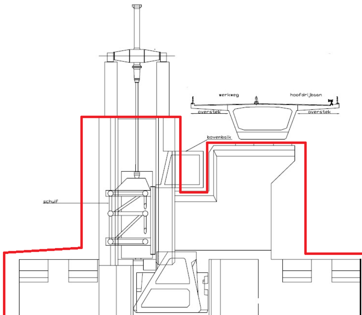
OBT-00018 Pijler
