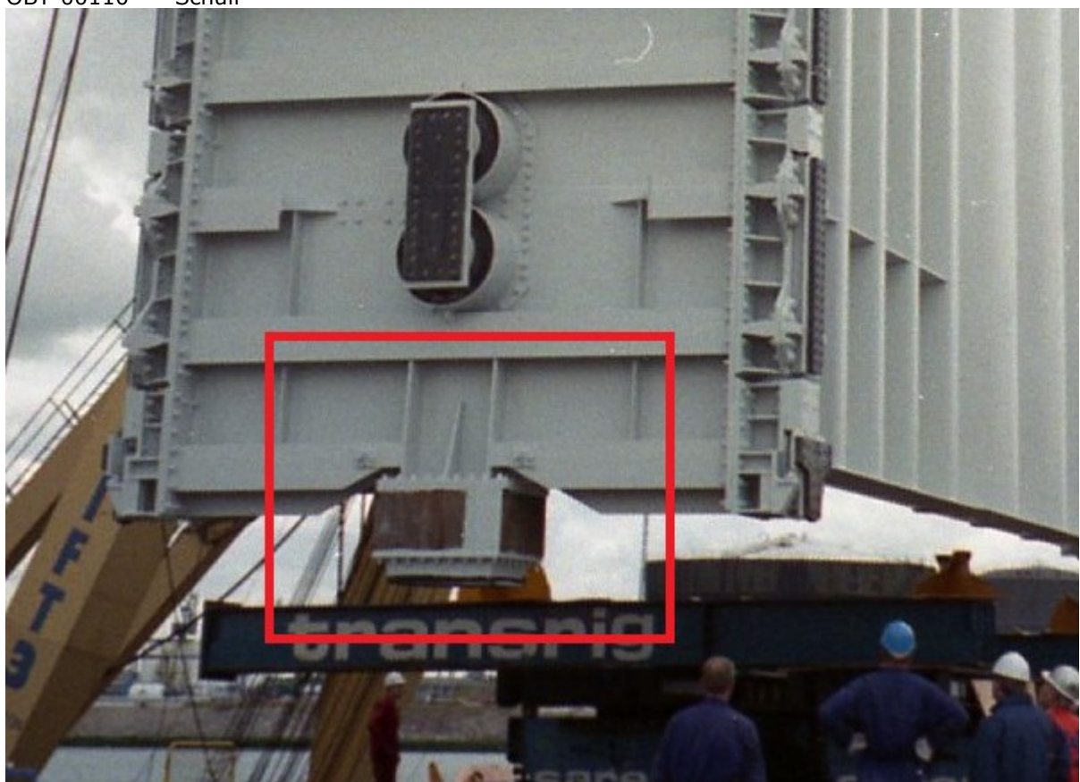
OBT-00111 Schuifonderaanslag
