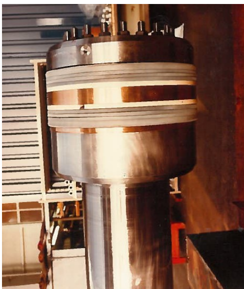
OBT-00067 Zuigergedeelte van de zuigerstang, Substelsiem
