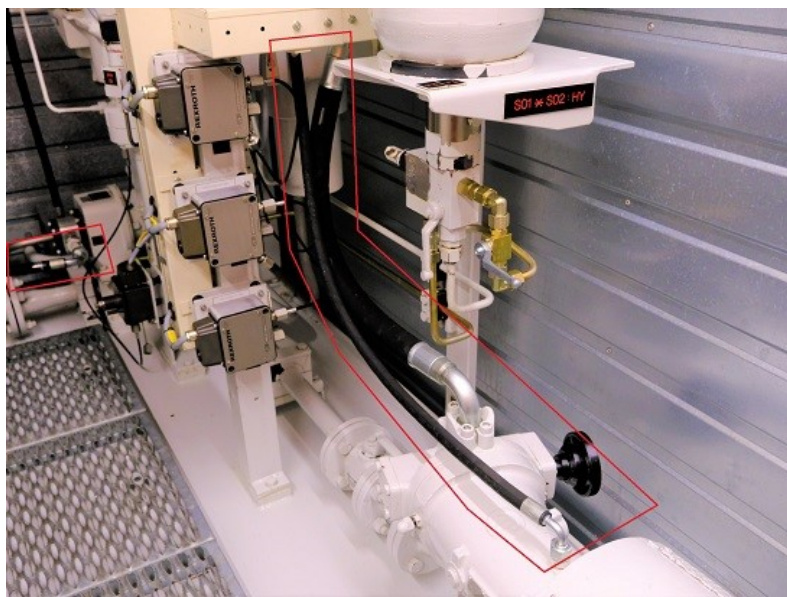
OBT-00101 Flexibele leiding van de EH-eenheid
