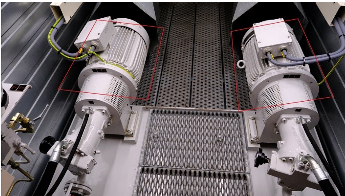
OBT-00092 E-motor in de container van de EH-eenheid
