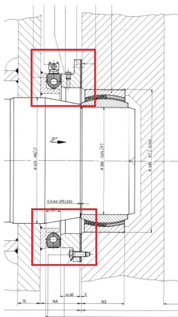
OBT-00047 Afdichtprofiel met steuning van de cardanbalkscharnieren
