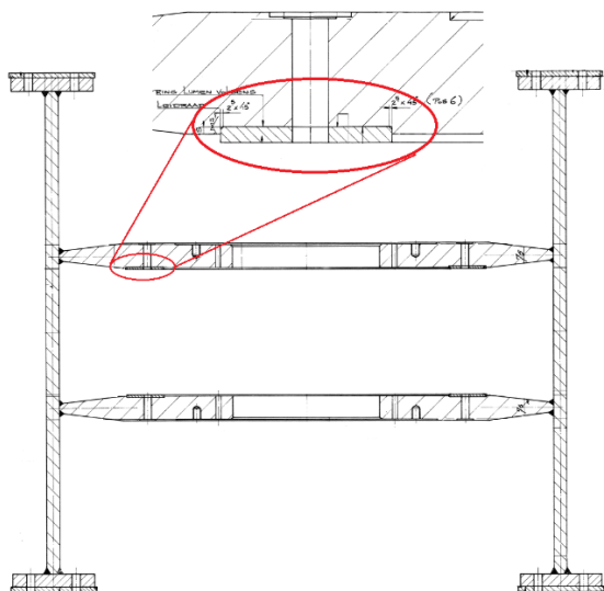
OBT-00088 Ingelijmde ring van de overgangsconstructie
