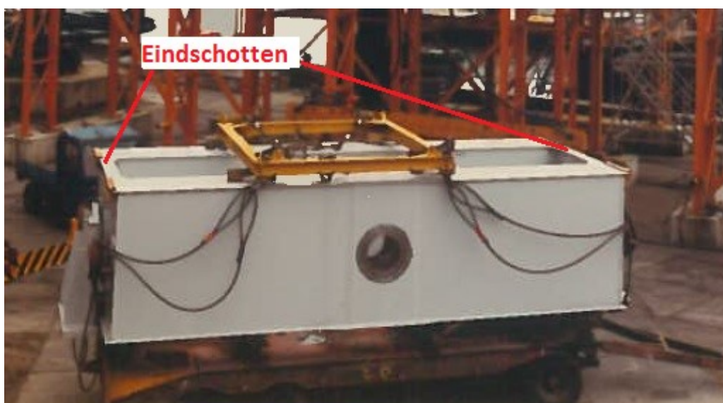
OBT-00043 Eindschot van de cardanbalk
