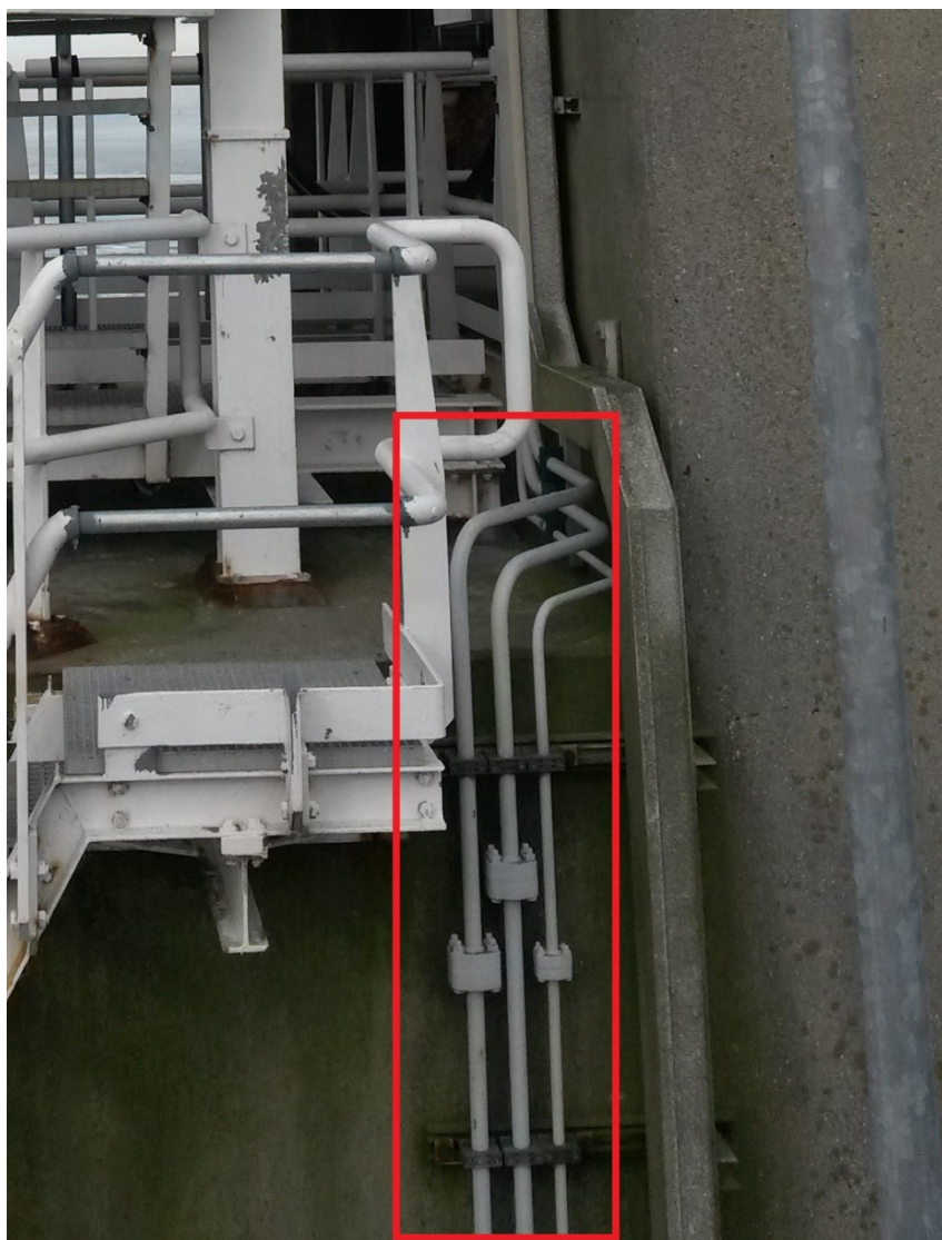
OBT-00038 Hydraulische leidingen op de pijler
