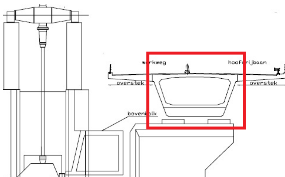
OBT-00010 Verkeerskoker
