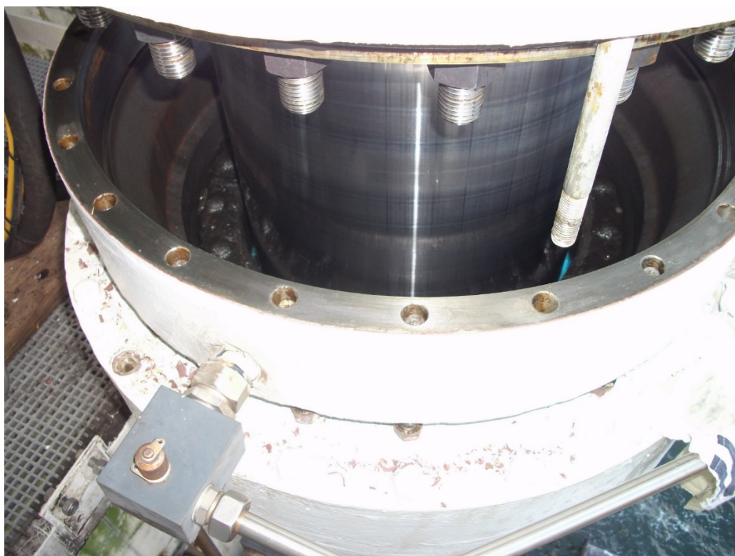
OBT-00063 Conserveringsolie-ruimte, Subsysteem
