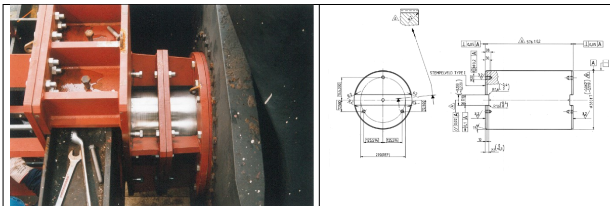
OBT-00086 Onderoogpen
