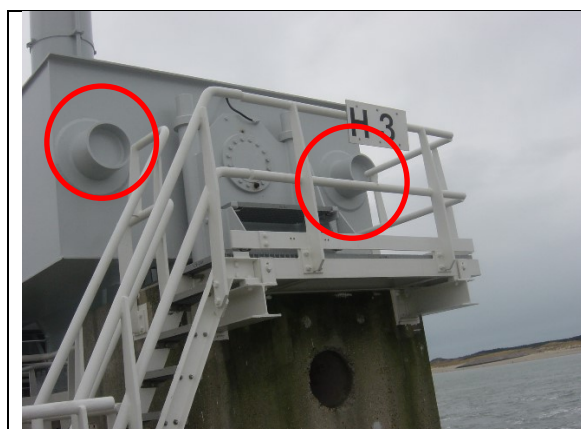
OBT-00044 Cardanbalkhijspunt
