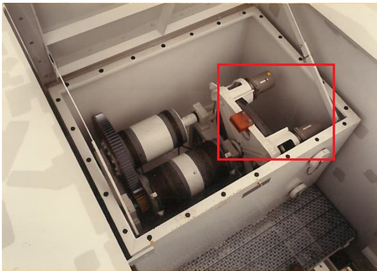
OBT-00109 Codegever van de gelijkloopinstallatie
