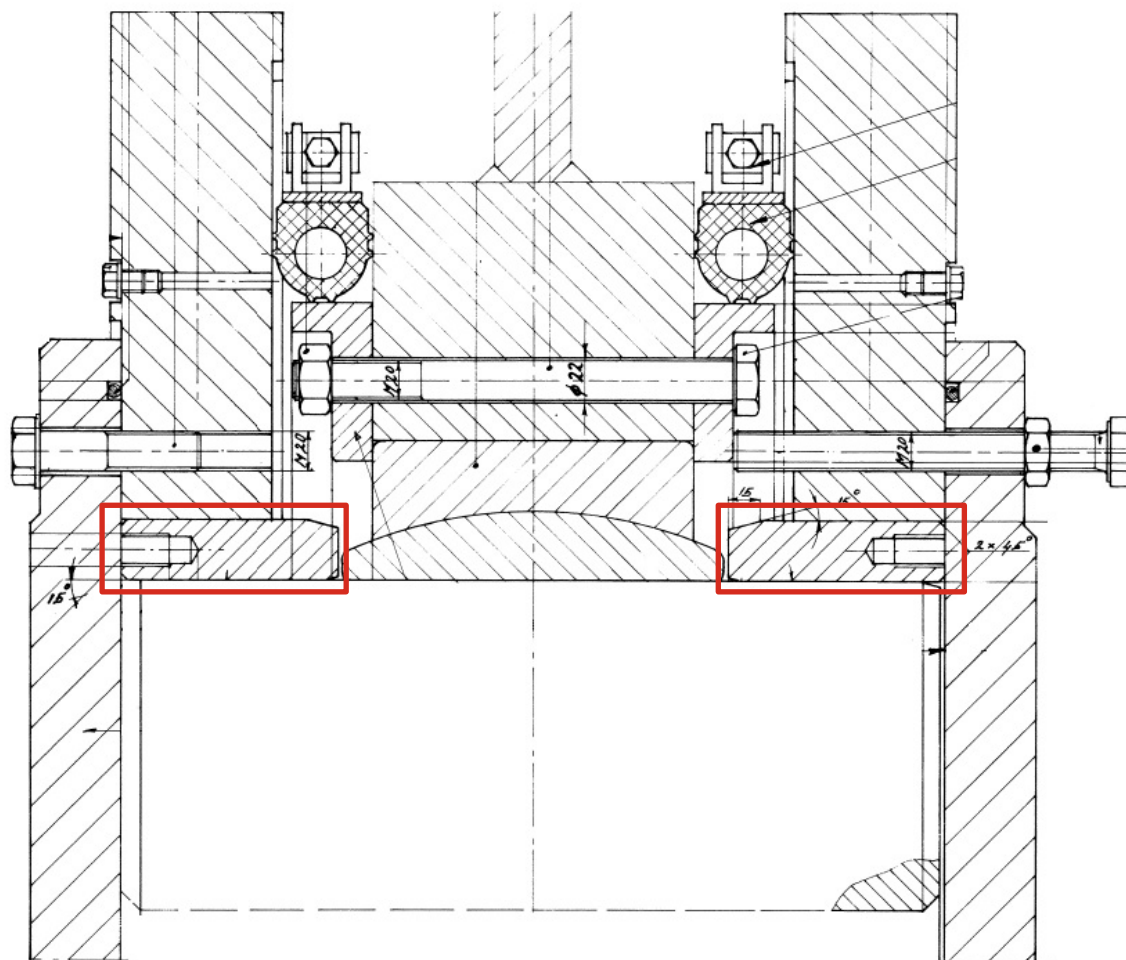
OBT-00054 cardanstoellagerafstandsbus
