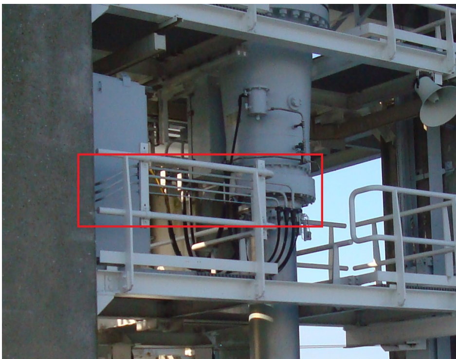
OBT-00144 Conserveringsolie-installatie Leidingen naar Cilinderlantaarnstuk
