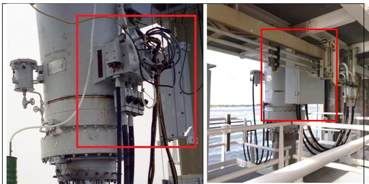
OBT-00065 Hydrauliekmontageblok (POS 72) van de cilinder
