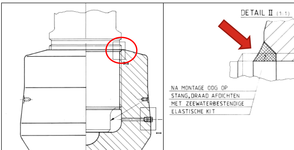
OBT-00135 Onderoog schroefdraadafdichting
