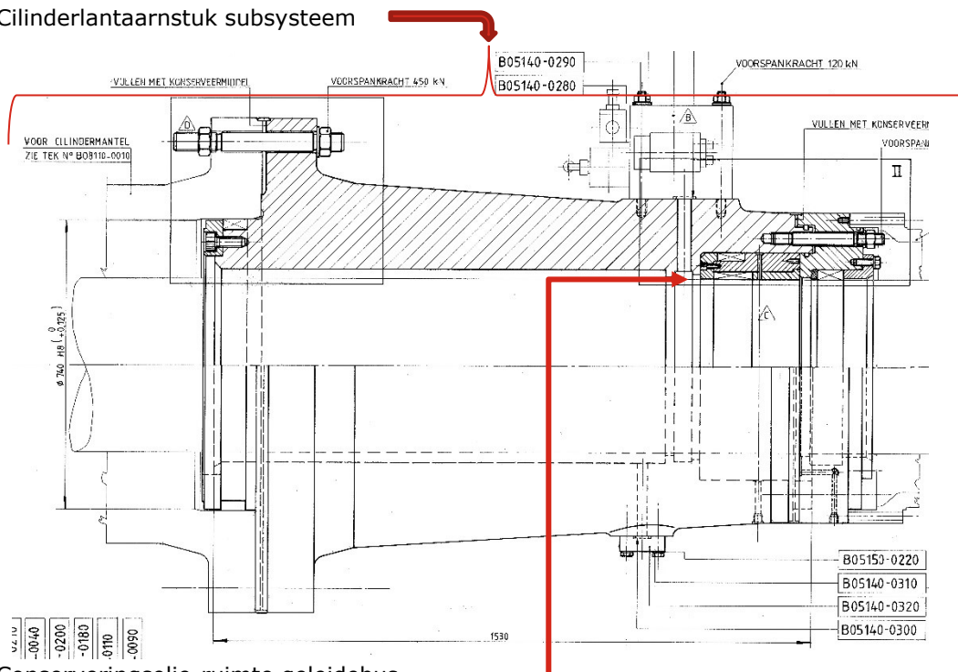
OBT-00132 Conserveringsolie-ruimte geleidebus
