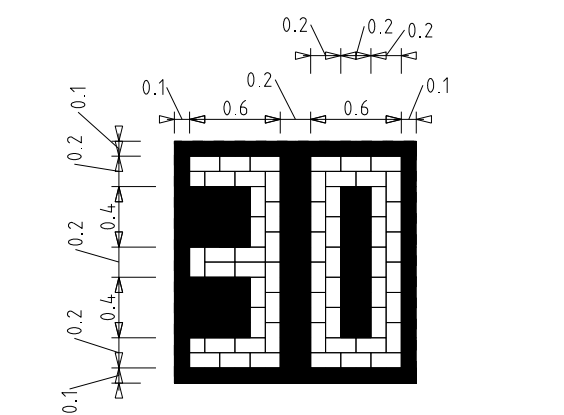
Detail tekst '30'
