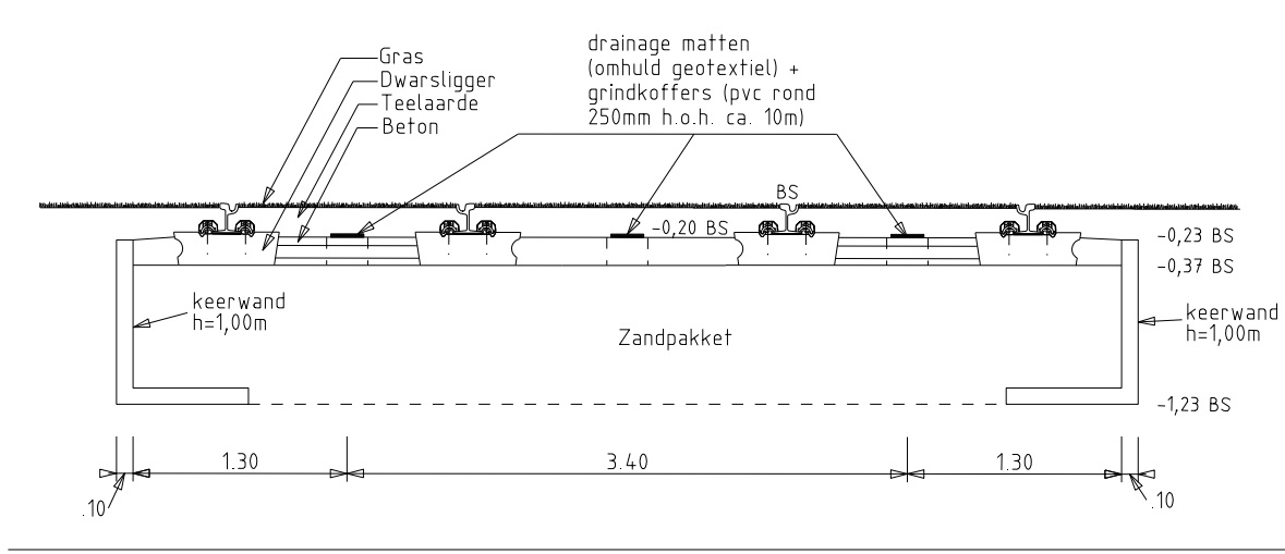
DWARSDOORSNEDE D-D (1:50)
