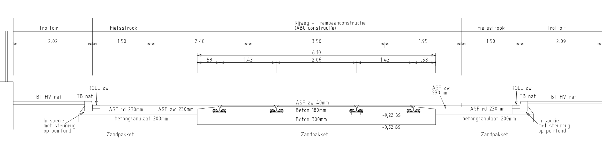
DWARSDOORSNEDE B-B (1:50)
