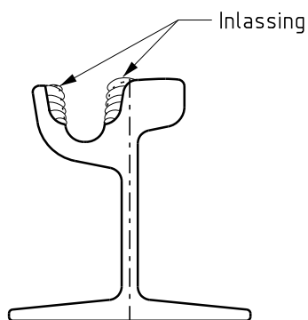
Aanzicht A-A
