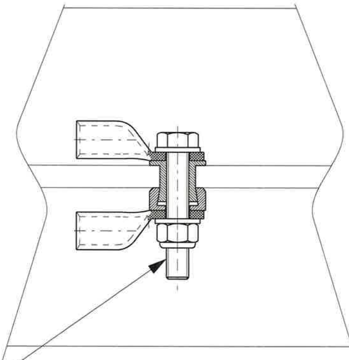
Doorsnede AA
