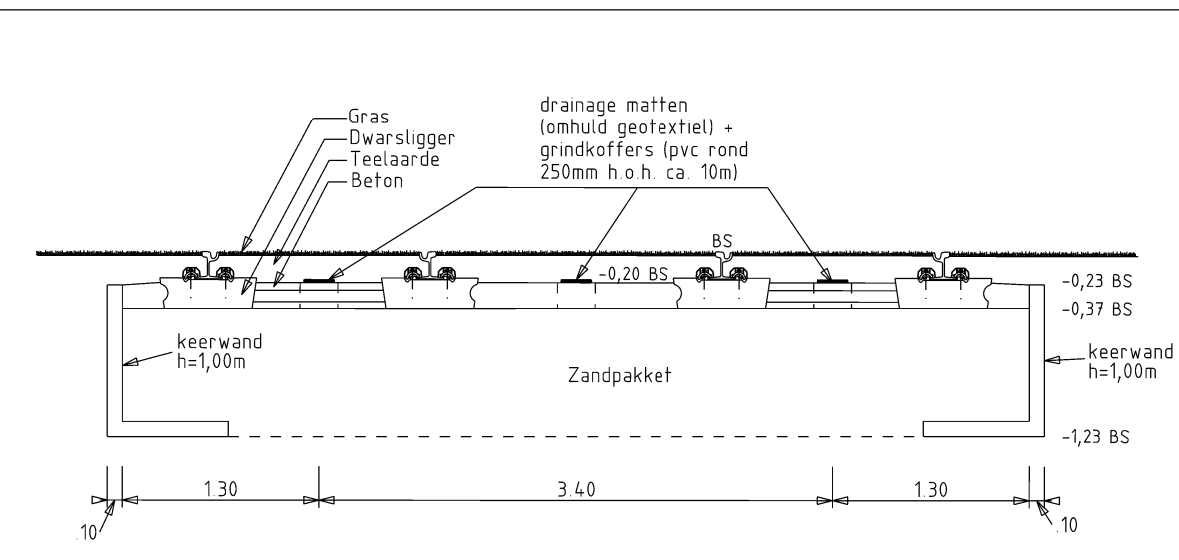
DWARSDOORSNEDE D-D (1:50)
