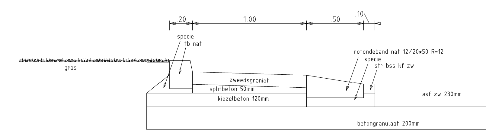
Detail Doorsnede rotonde (zonder trambaan)
