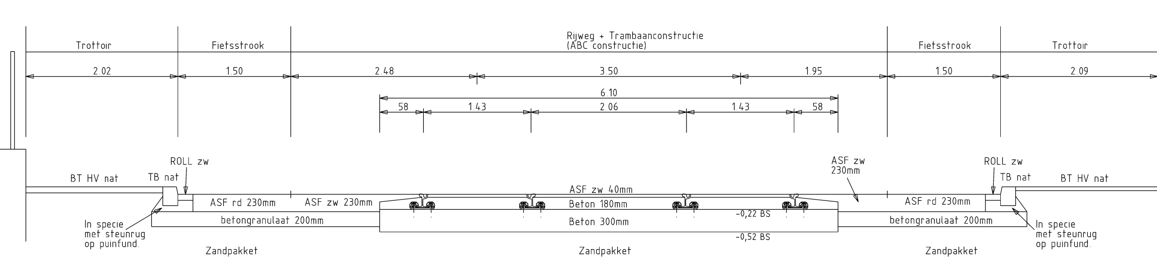
DWARSDOORSNEDE B-B (1:50)
