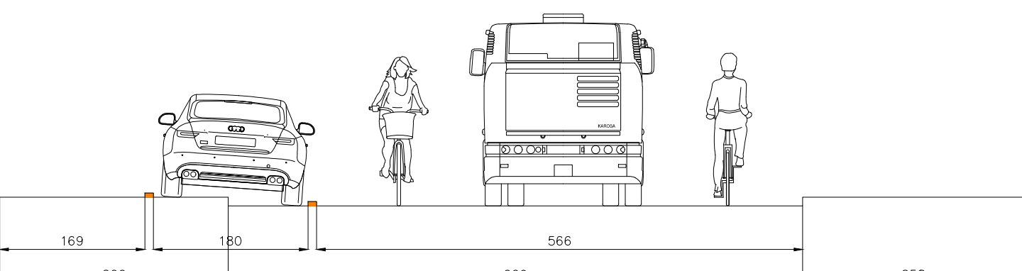
Dwarsprofiel E
