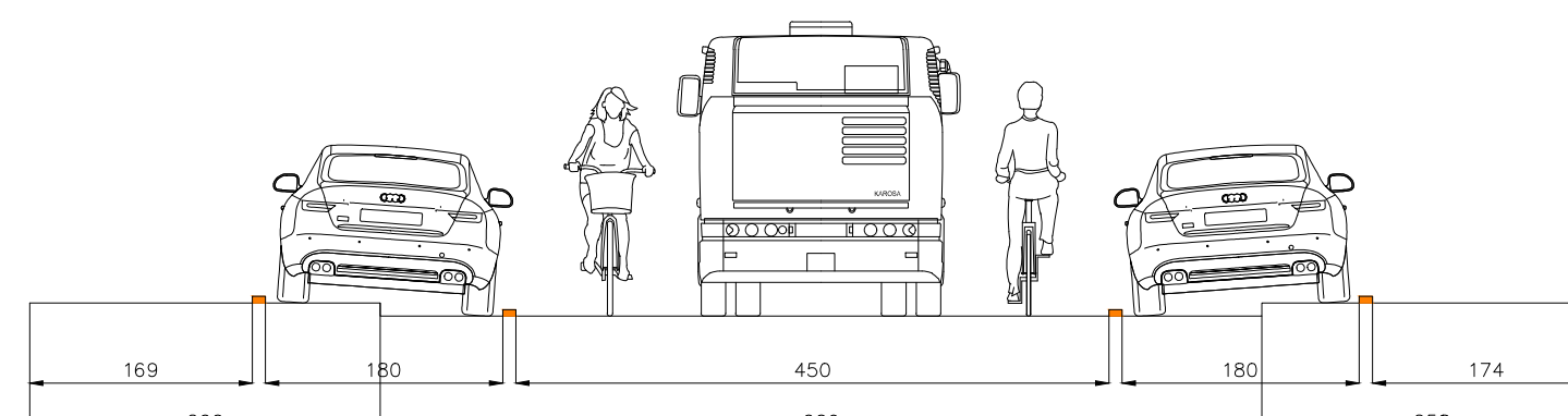
Dwarsprofiel D
